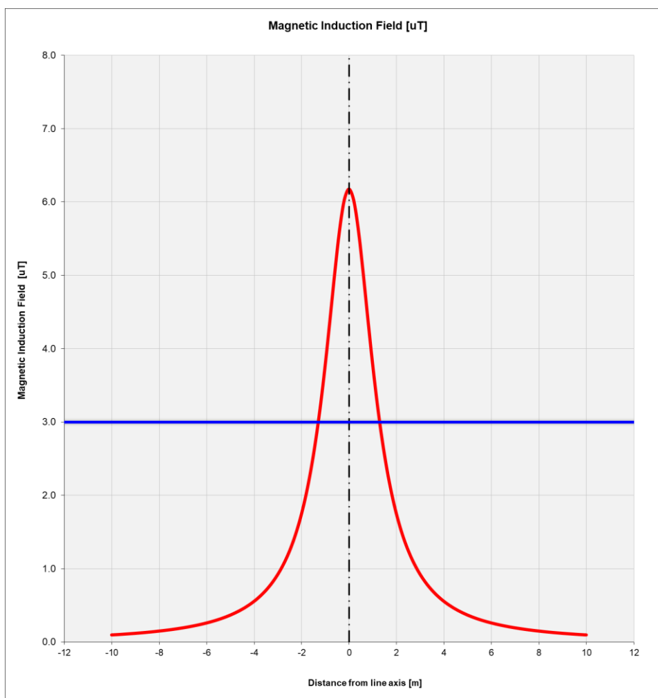
Figura 3: Andamento dell'induzione magnetica prodotta dalla linea in cavo AT calcolata a livello del suolo
