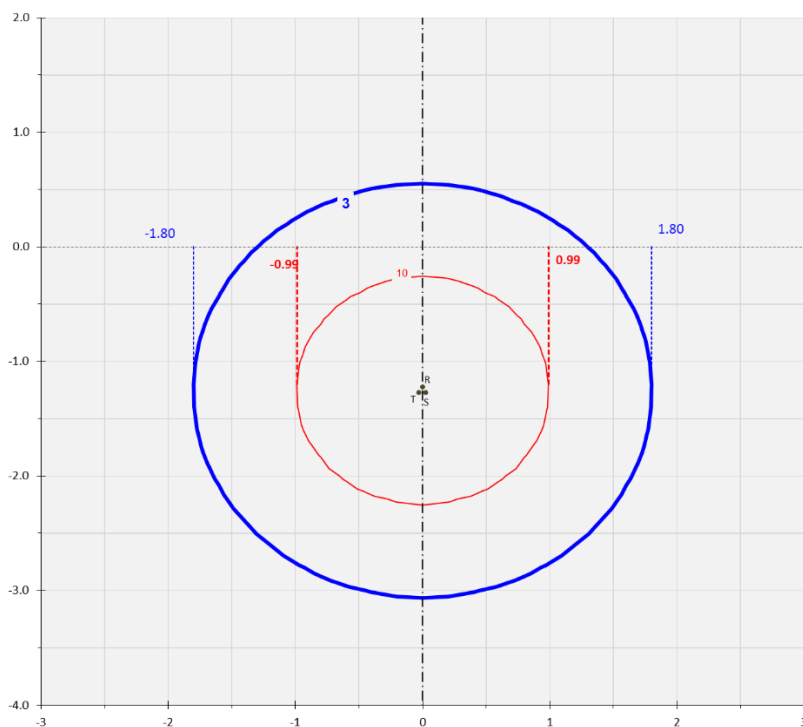
Figura 2: Andamento dell'induzione magnetica prodotta dalla linea in cavo AT calcolata a livello del suolo
