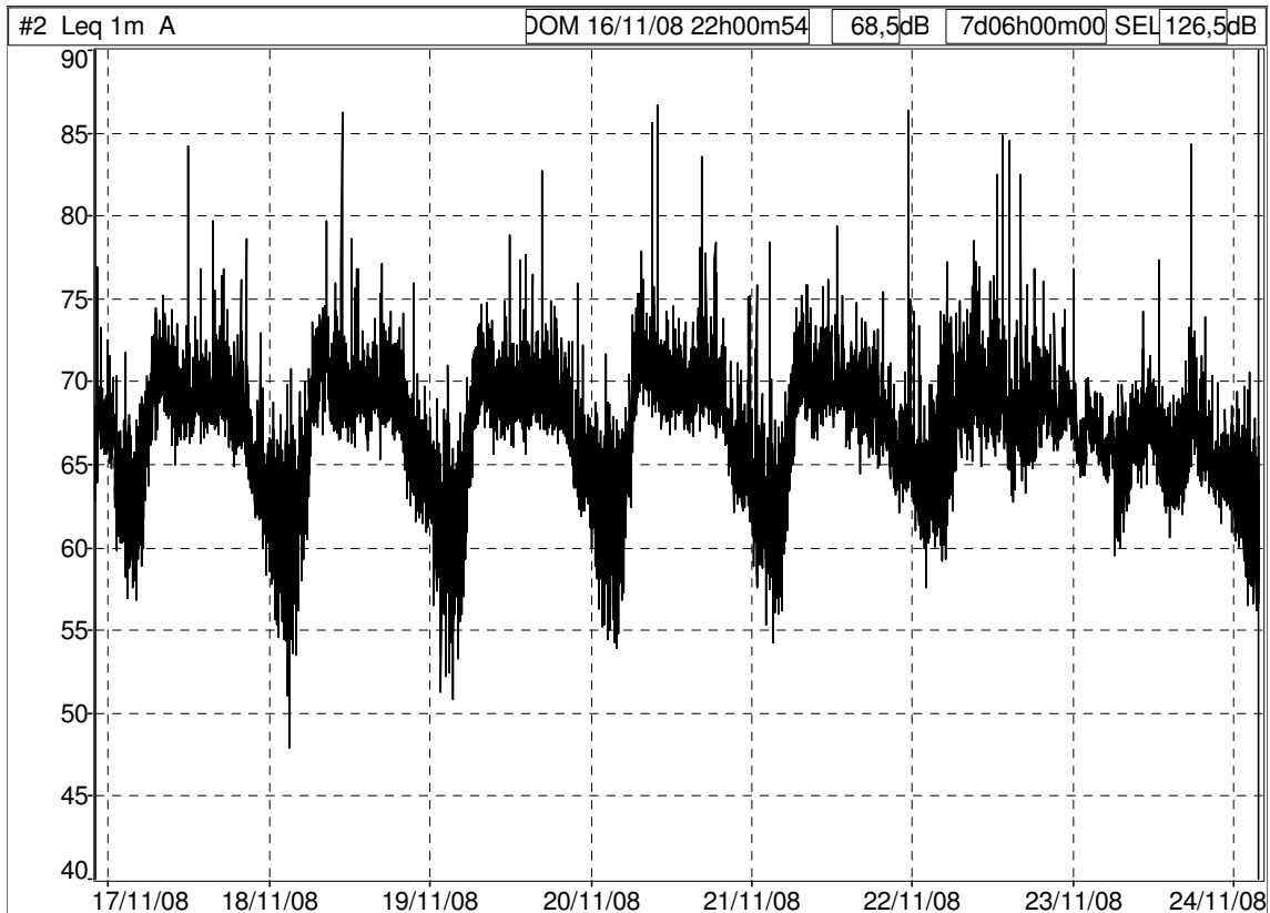
Storia temporale settimanale, sito Parking Amari (Fonte: dB TRAIT).
