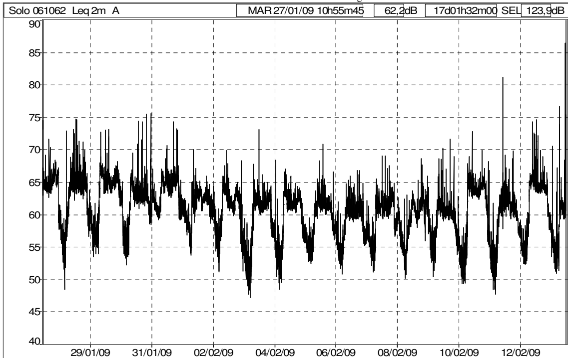
Storia temporale, sito Capitaneria di Porto (Fonte: dB TRAIT).
