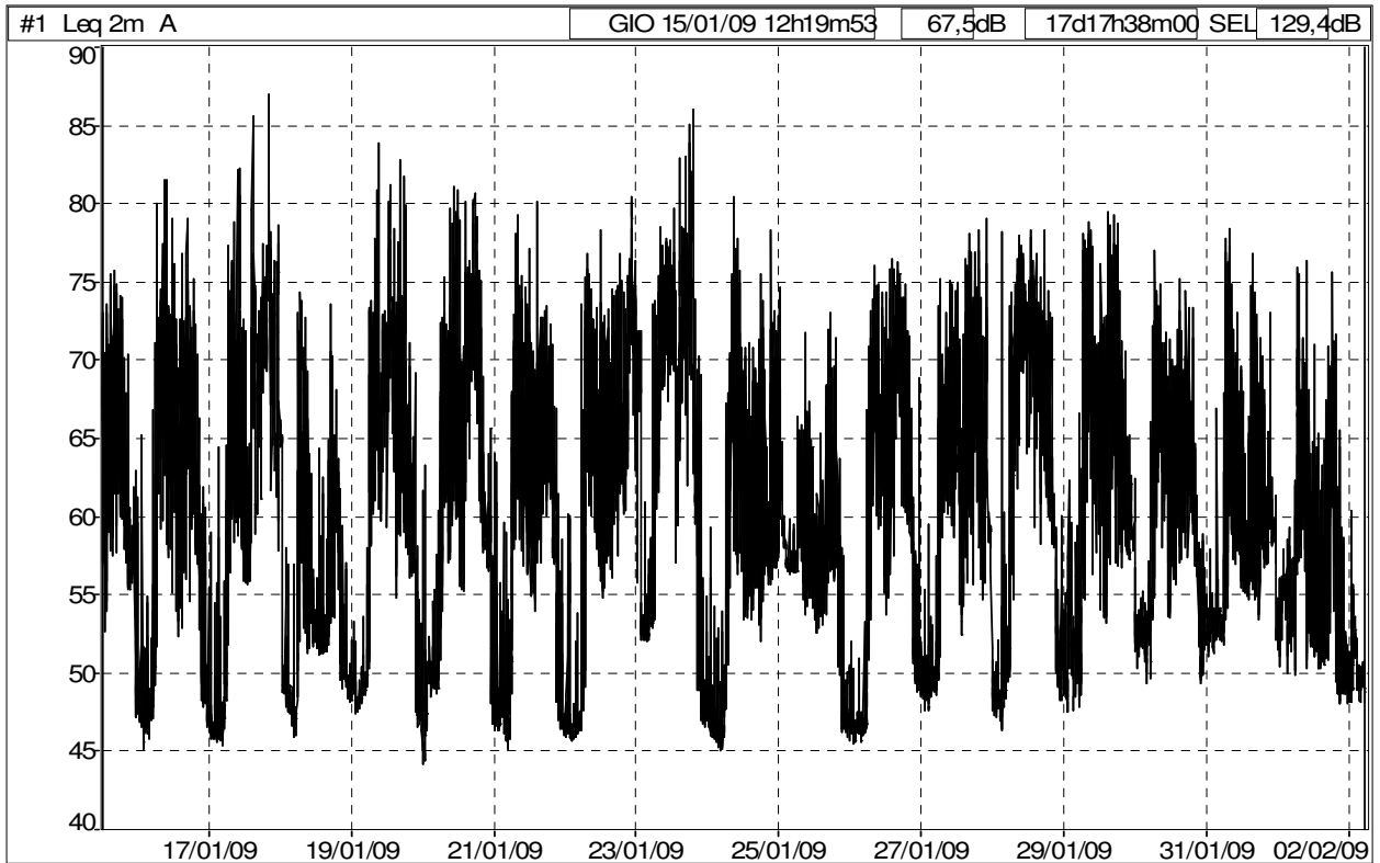
Storia temporale, sito Deposito Containers (Fonte: dB TRAIT).
