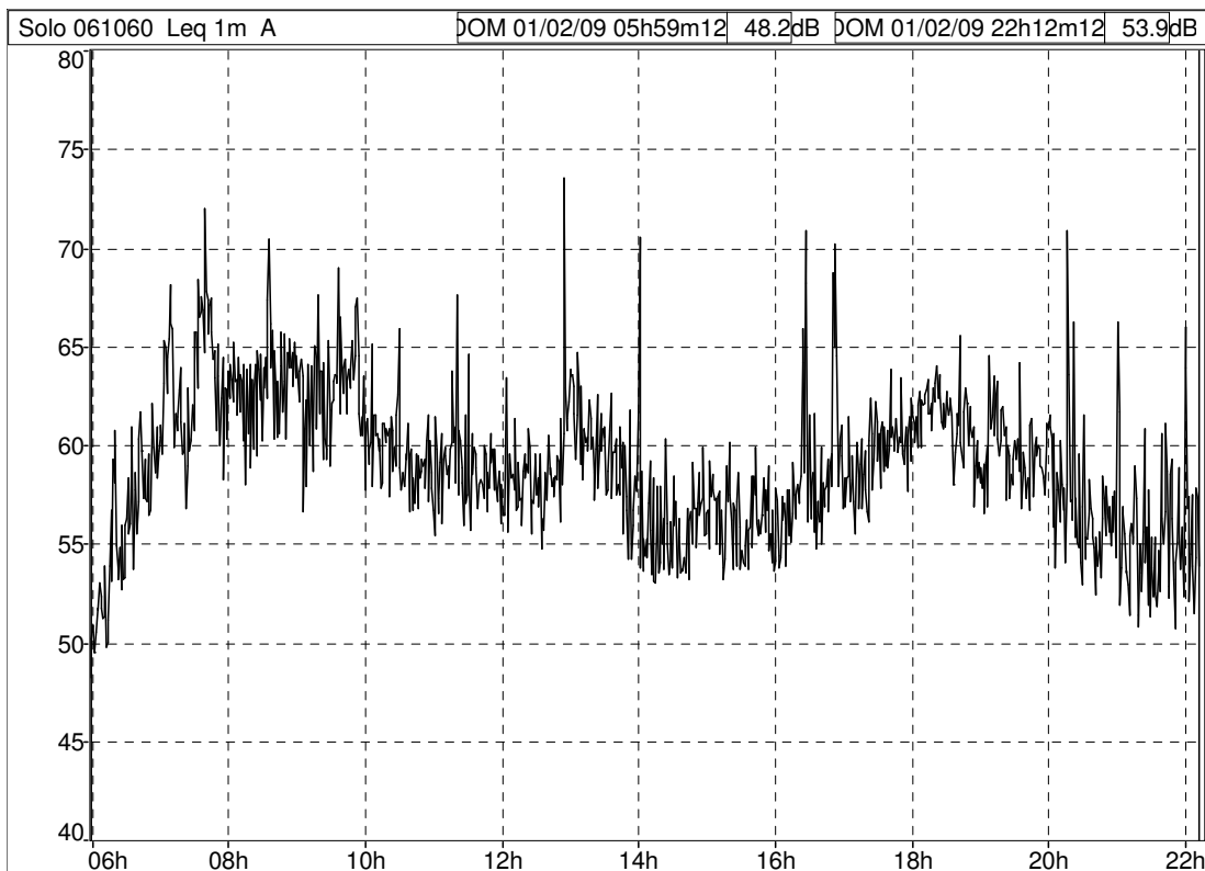
Storia temporale giornaliera per una domenica, sito via C. Colombo (Fonte: dB TRAIT).
