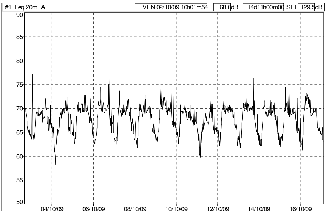
Storia temporale dal 02/10/09 al 17/10/09, sito Parking Amari (Fonte: dB TRAIT).
