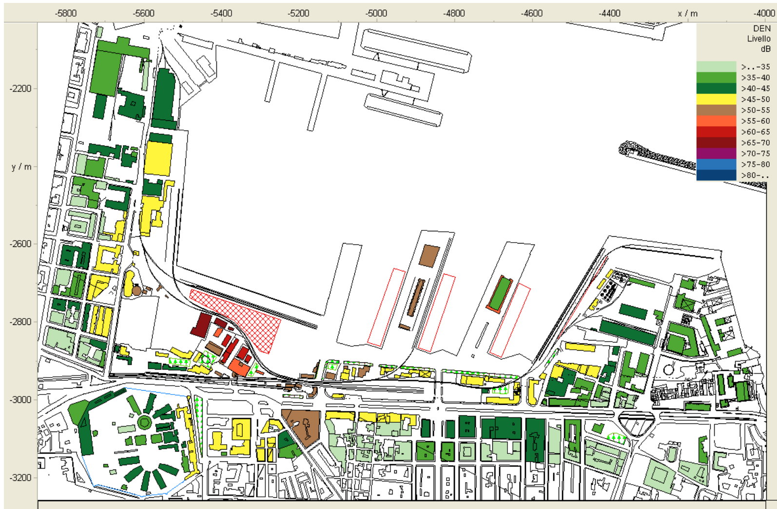
Mappa L DEN , livelli di facciata, simulazione "Rumore portuale" (Fonte: IMMI).
