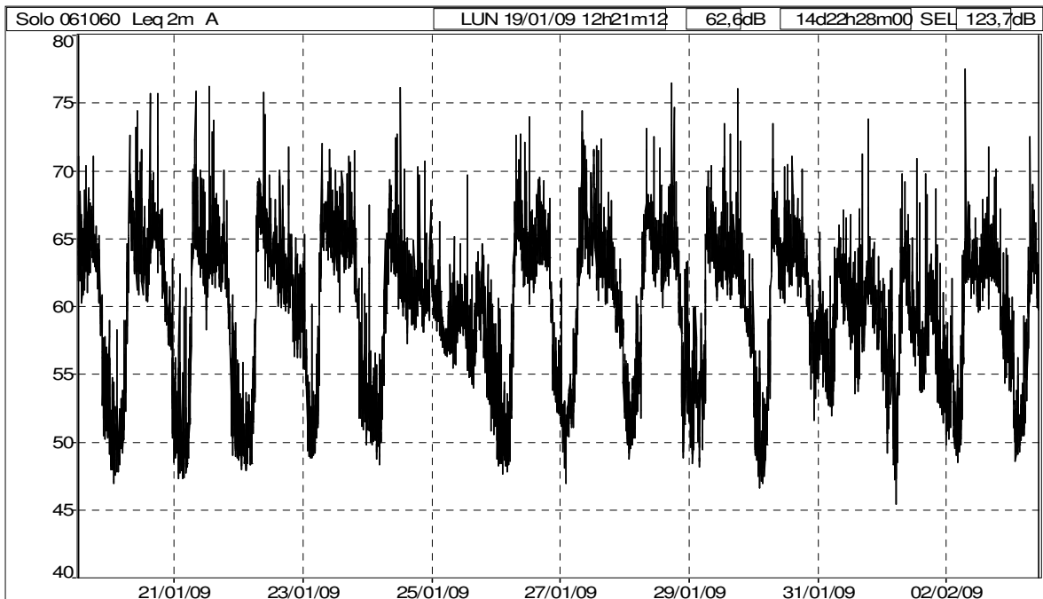
Storia temporale sito via C. Colombo (Fonte: dB TRAIT).
