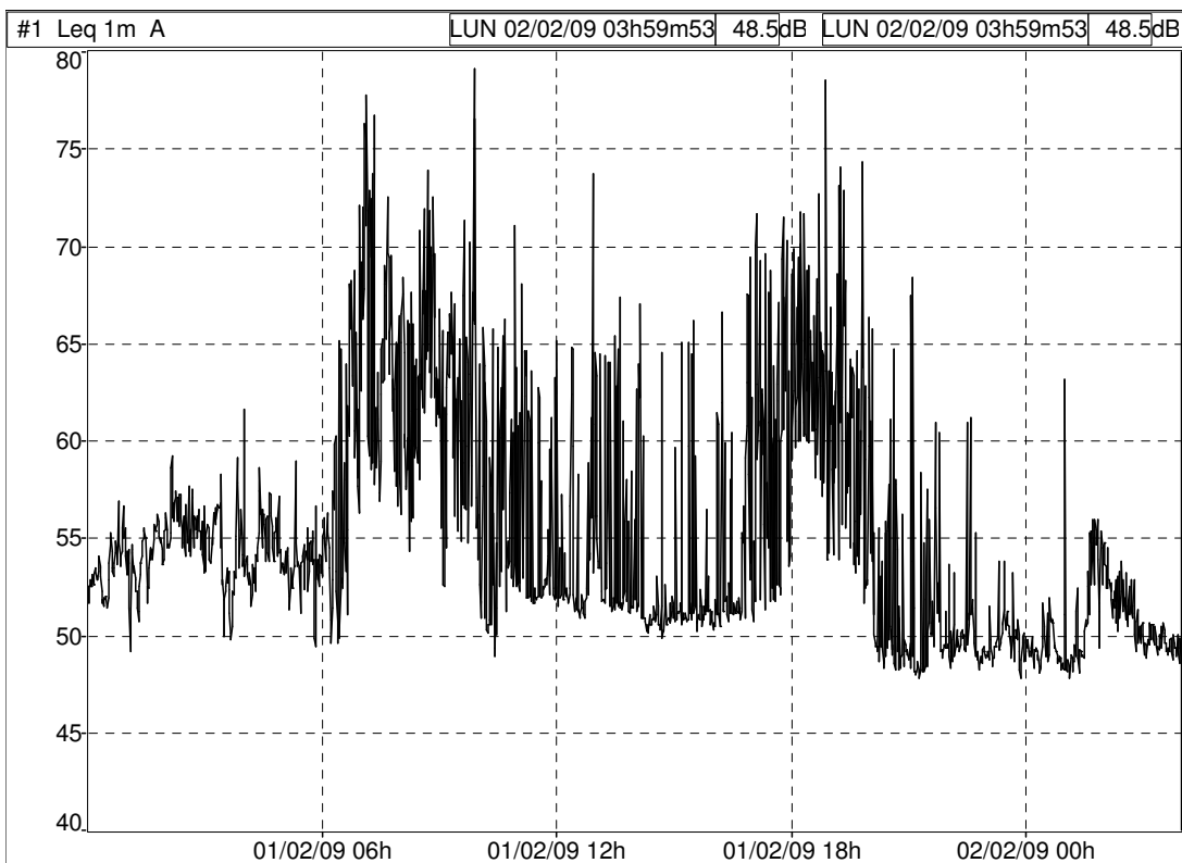
Storia temporale domenica 01/02/2009, sito Deposito Containers (Fonte: dB TRAIT).
