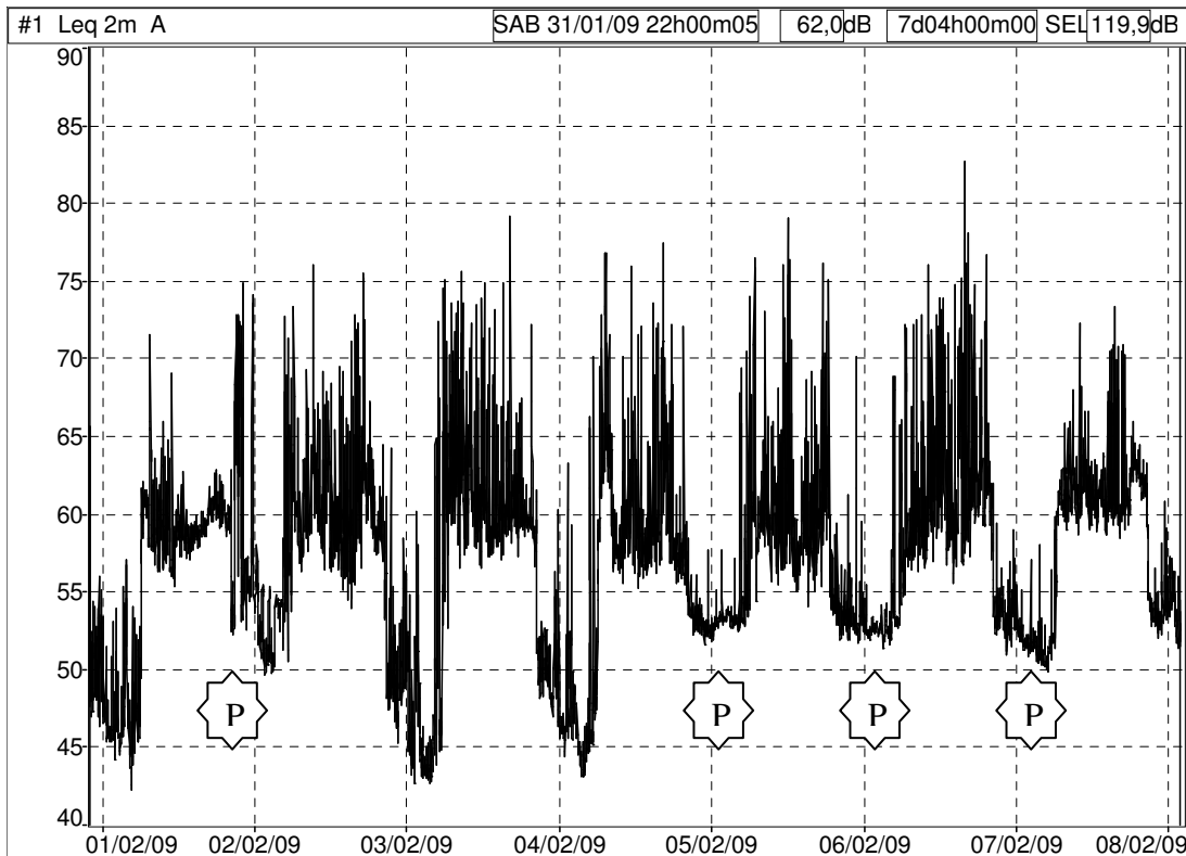
Storia temporale settimanale sito Sammuzzo (Fonte: dB TRAIT).
