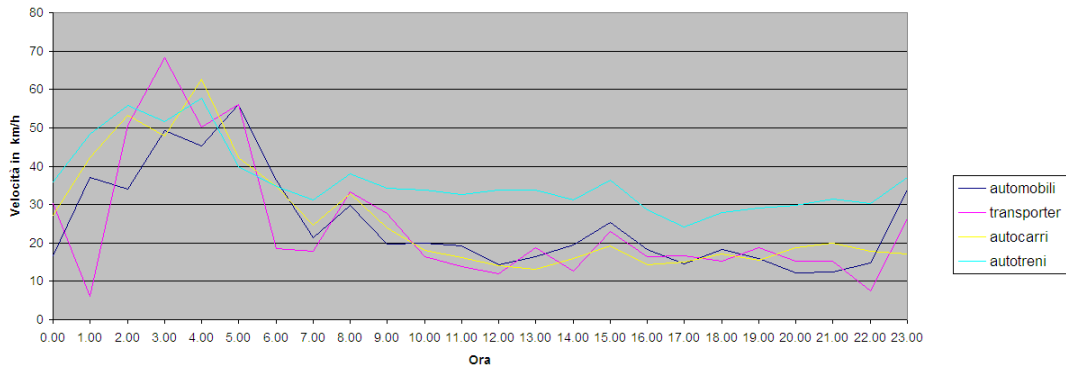
Andamento velocità minima
