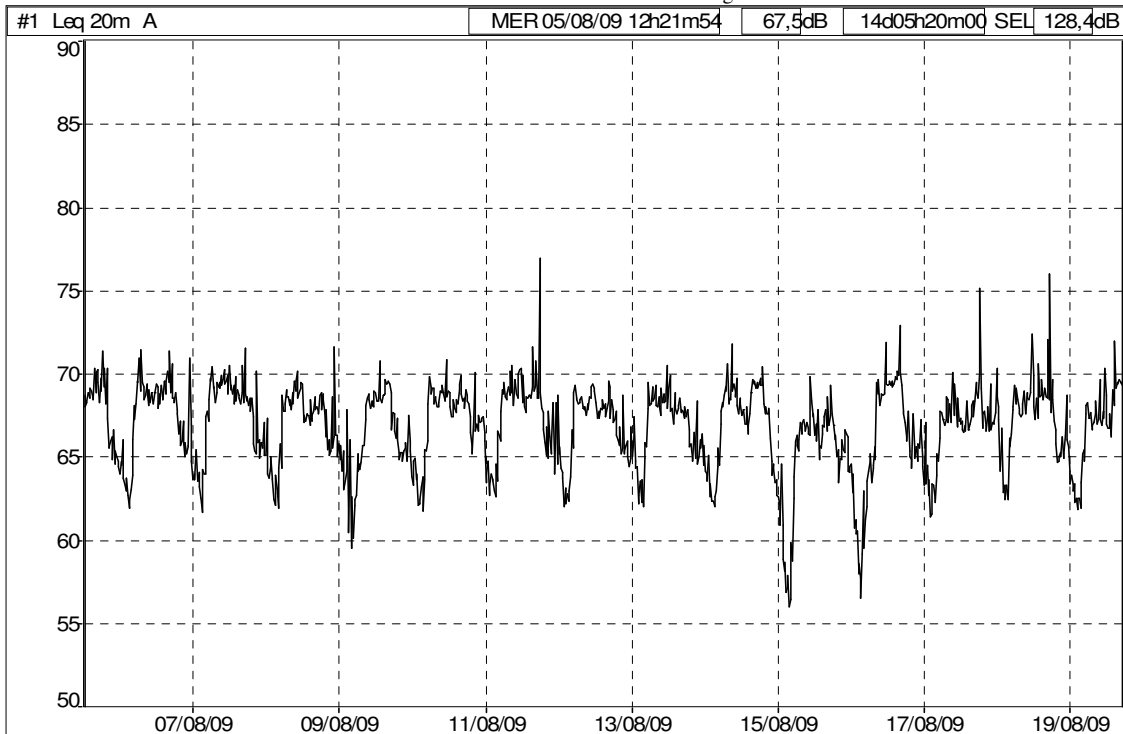
Storia temporale dal 05/08/09 al 19/08/09, sito Parking Amari (Fonte: dB TRAIT).
