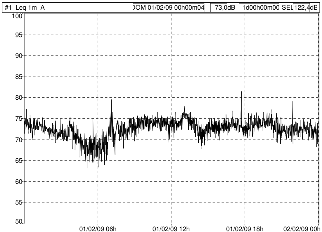
Storia temporale domenica 01/02/2009, sito via Crispi 120(Fonte: dB TRAIT).
