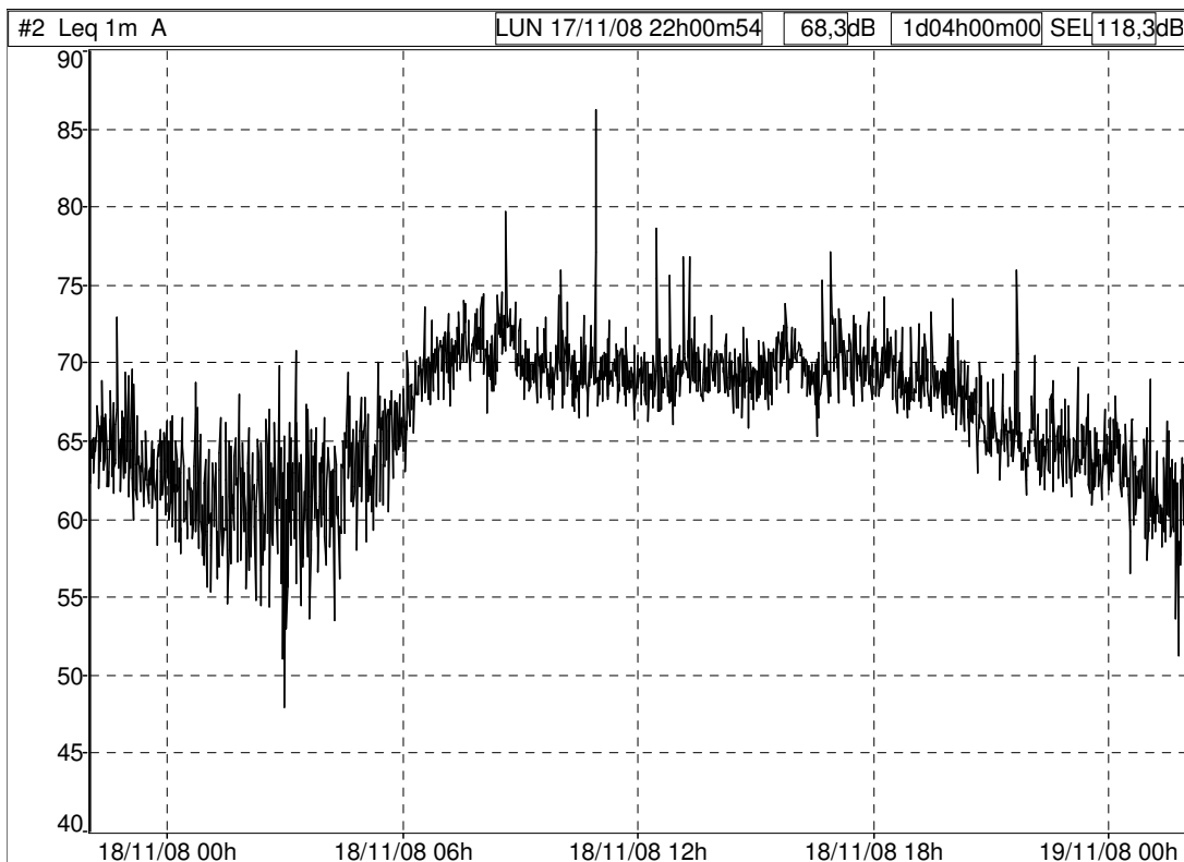
Storia temporale giorno feriale, sito Parcheggio (Fonte: dB TRAIT).
