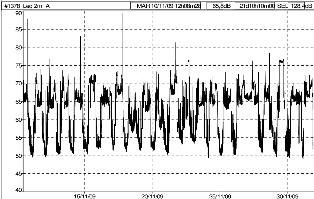
Storia temporale Stazione Marittima (Fonte: dB TRAIT).
