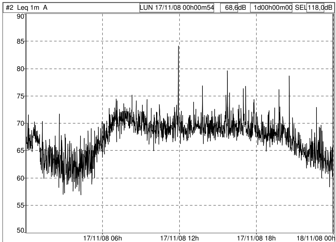
Storia temporale giornaliera, sito Parcheggio (Fonte: dB TRAIT).
