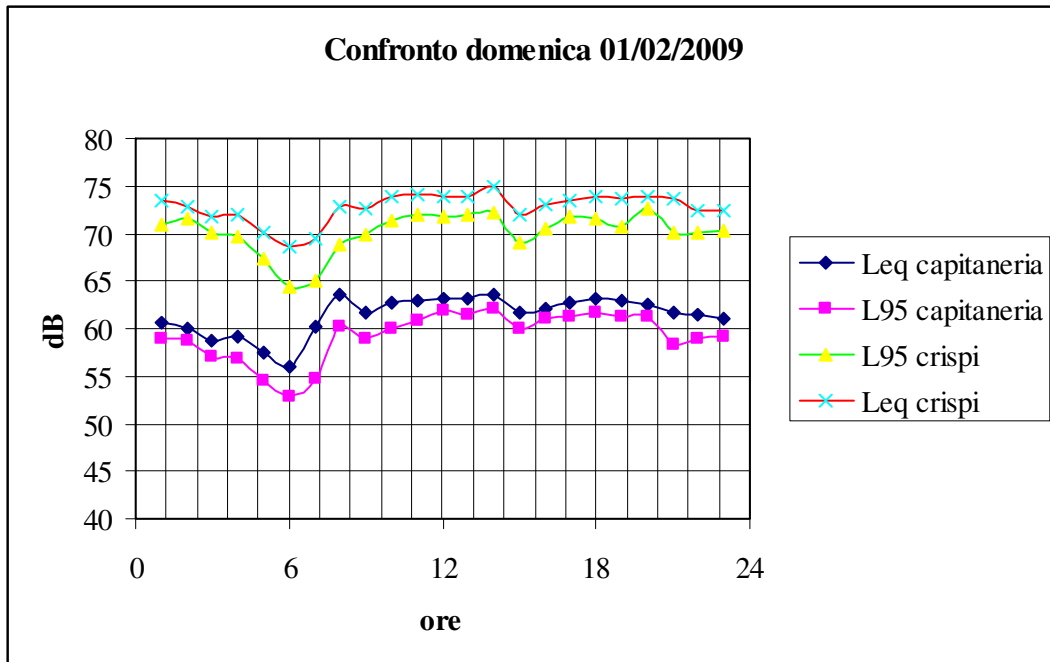
Grafico L_{eq} e L_{95} , domenica 01/02/2009, confronto (Fonte dati: DB TRAIT).
