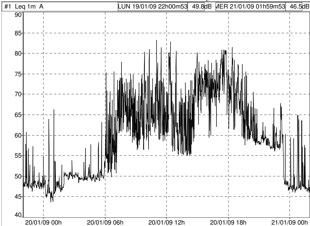
Storia temporale giorno feriale, sito Deposito Containers (Fonte: dB TRAIT).
