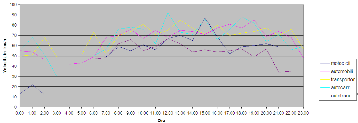
Andamento velocità massima
