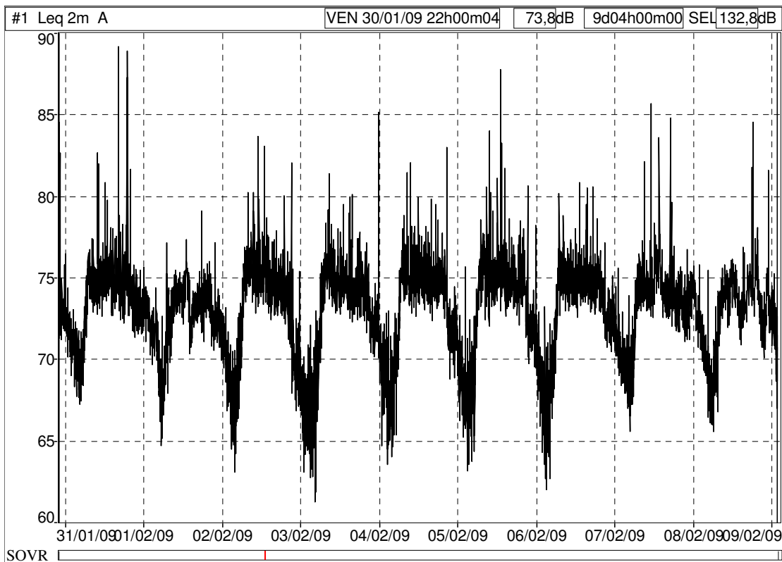
Storia temporale settimanale, sito via Crispi 120 (Fonte: dB TRAIT).
