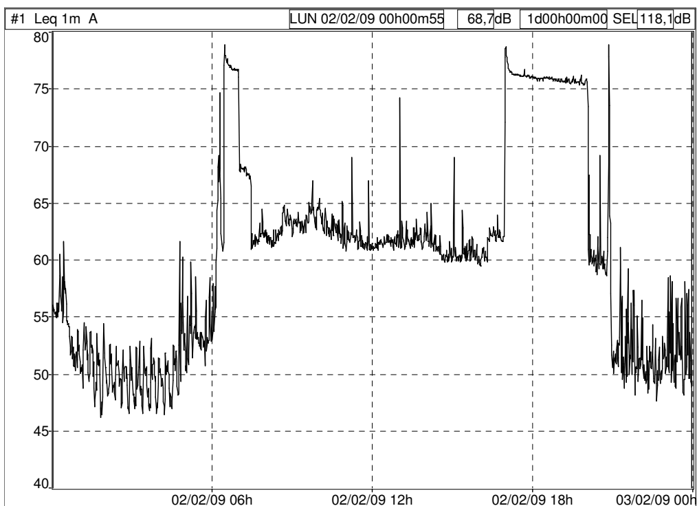
Storia temporale giornaliera sito Stazione Marittima (Fonte: dB TRAIT).
