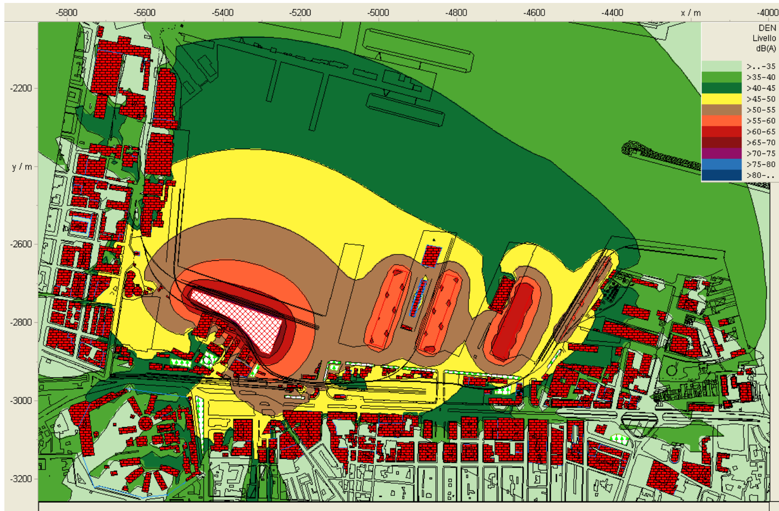
Mapa L_{DEN} simulazione “ Rumore portuale ” (Fonte: IMMI).
