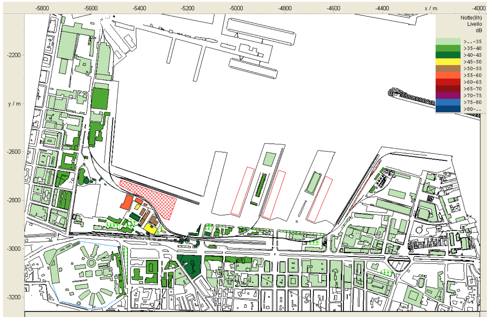
Mapa L night , livelli di facciata, simulazione “Rumore portuale” (Fonte: IMMI).
