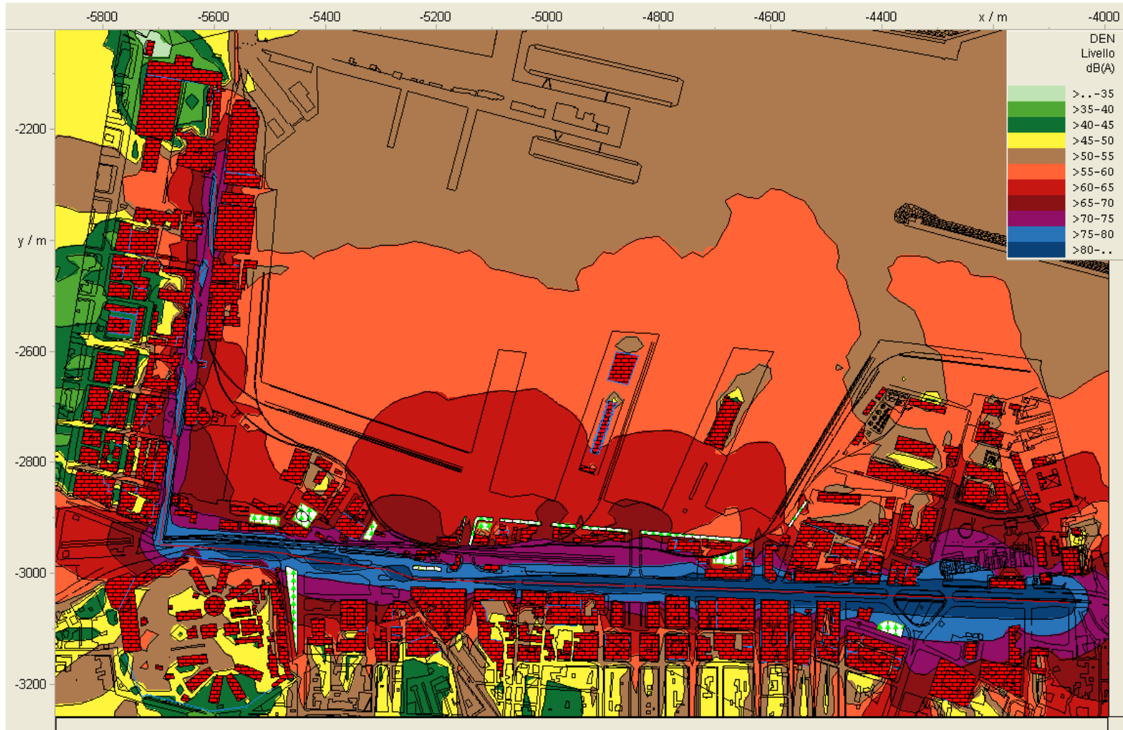
Mappa L DEN , simulazione “ Traffico stradale ” (Fonte: IMMI).
