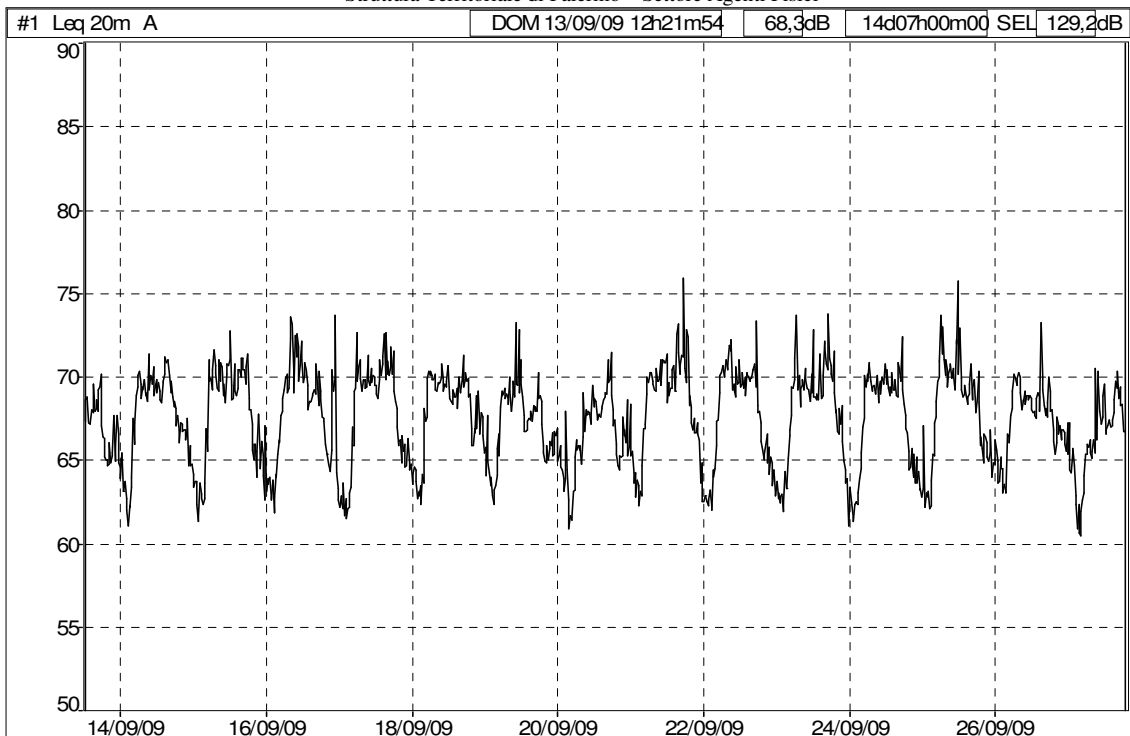
Storia temporale dal 13/09/09 al 28/09/09, sito Parking Amari (Fonte: dB TRAIT).
