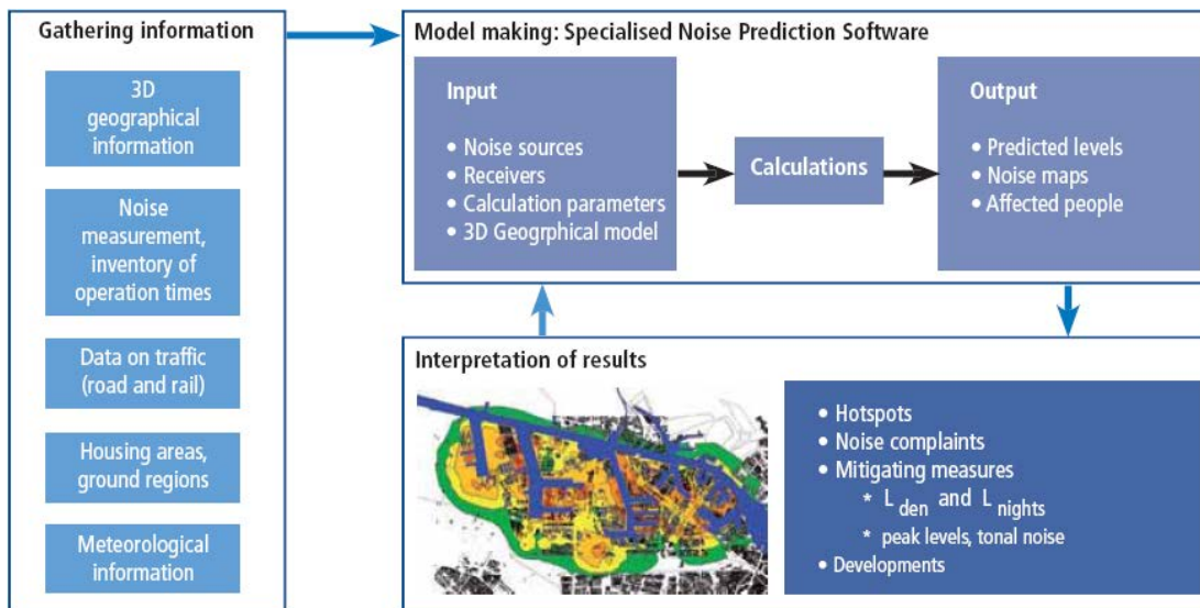
Schema di funzionamento di un software per l'analisi acustica previsionale
