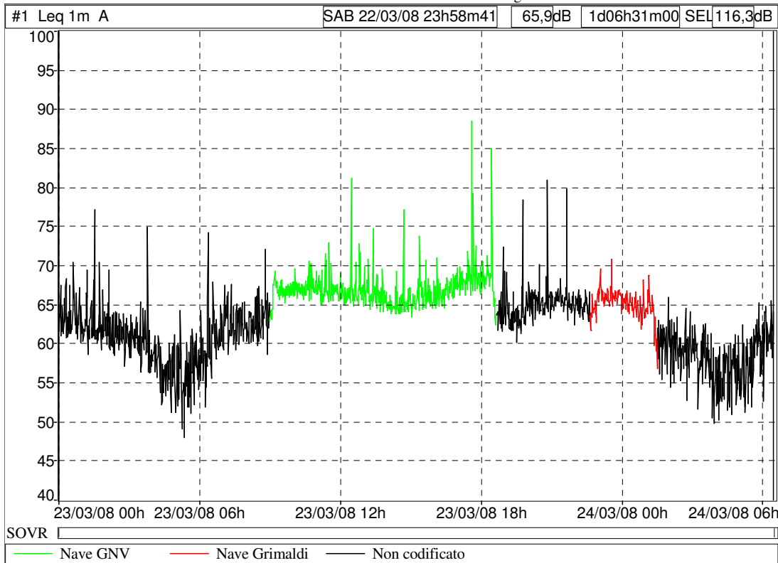
Storia temporale domenica sito Parcheggio (Fonte: dB TRAIT).
