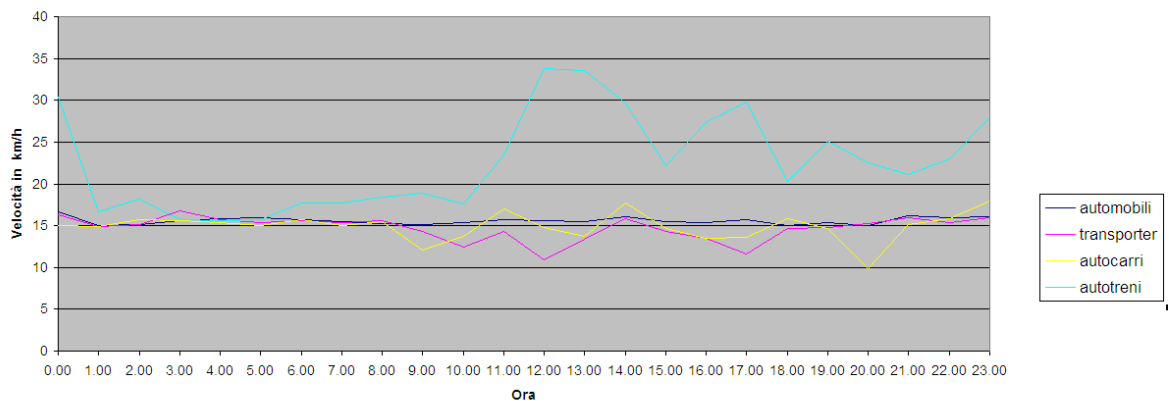
Andamento velocità minima
