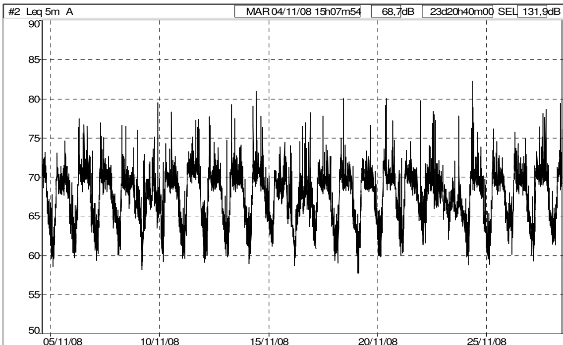
Storia temporale dal 04/11/08 al 28/11/08, sito Parking Amari (Fonte: dB TRAIT).
