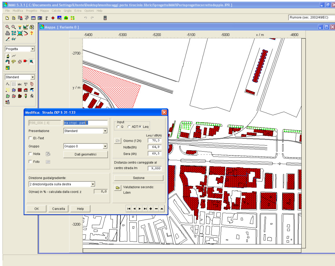
Schermata sorgente da traffico stradale (Fonte: IMMI).
