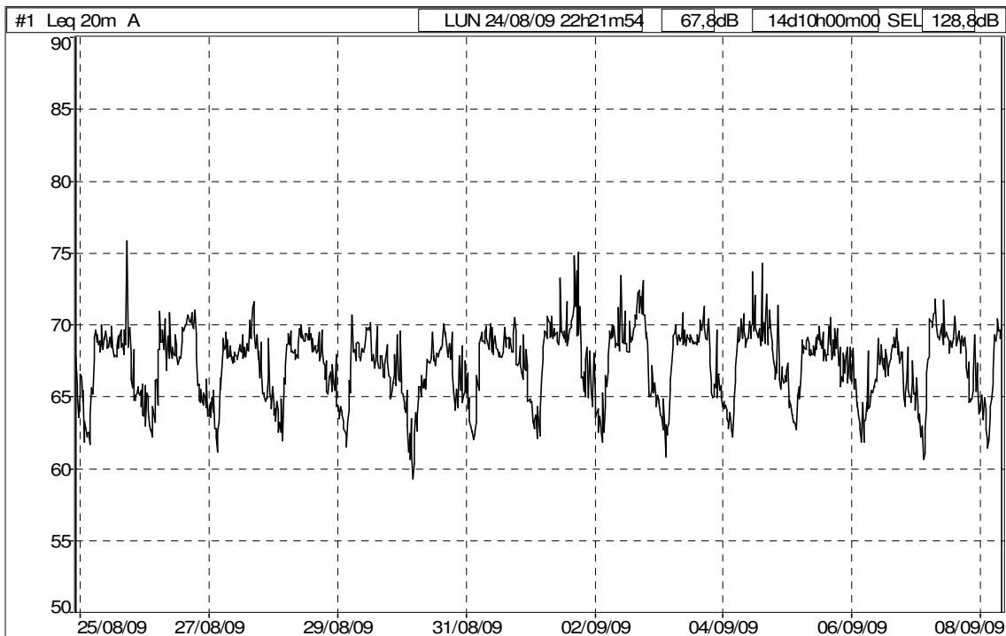
Storia temporale dal 24/08/09 al 08/09/09, sito Parking Amari (Fonte: dB TRAIT).
