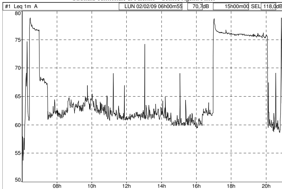
Storia temporale con nave in rada, sito Stazione Marittima (Fonte: dB TRAIT).
