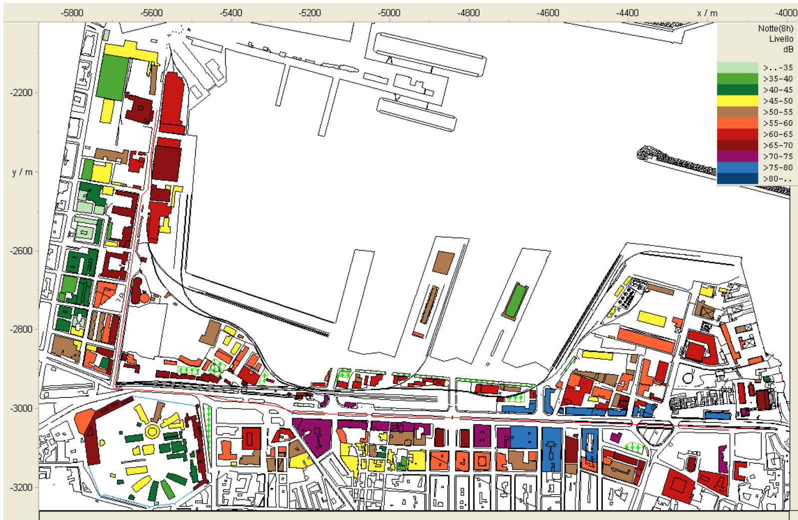
Mappa L night , livelli di facciata, simulazione "Traffico stradale" (Fonte: IMMI).
