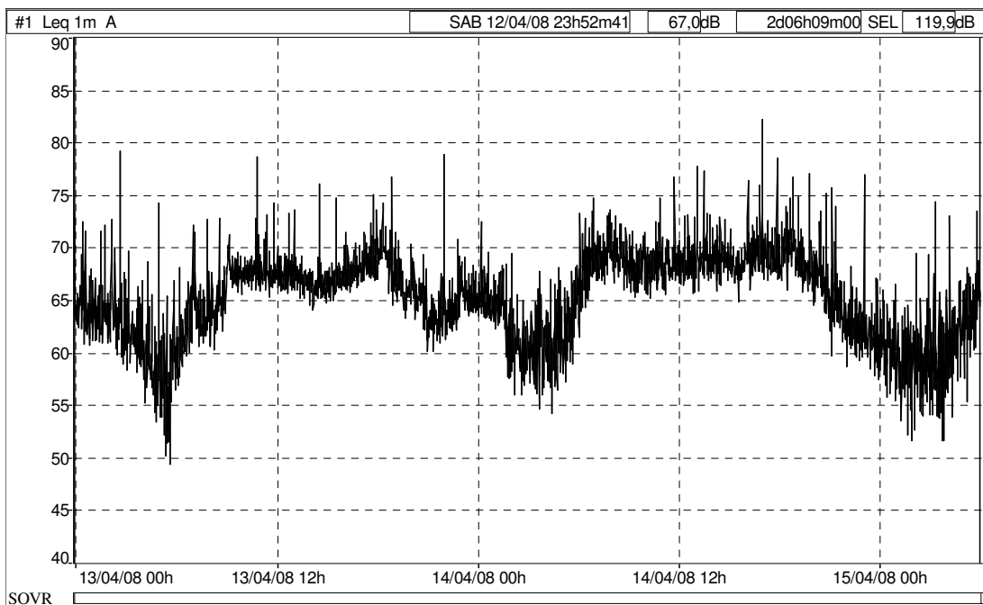
Storia temporale domenica e lunedì, sito Parcheggio (Fonte: dB TRAIT).
