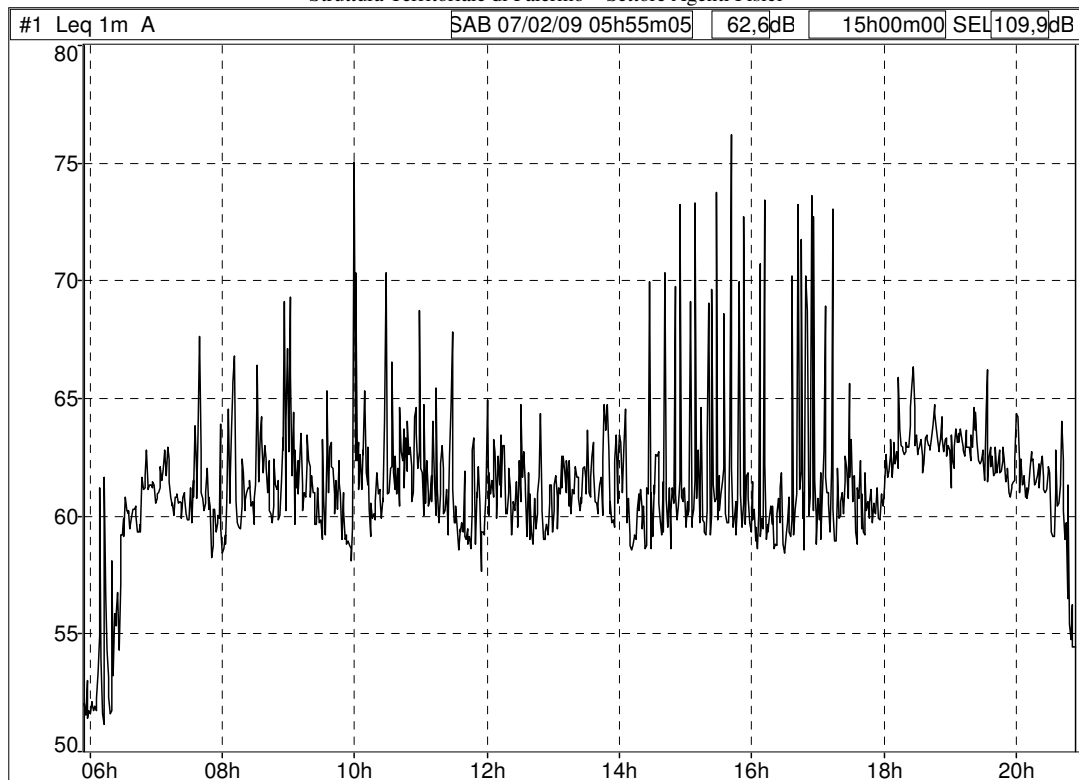
Storia temporale giornaliera sito molo Sammuzzo (Fonte: dB TRAIT).
