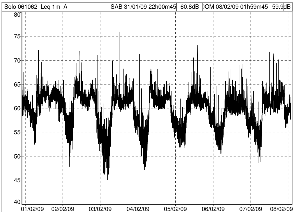
Storia temporale settimanale, sito Capitaneria di Porto (Fonte: dB TRAIT).
