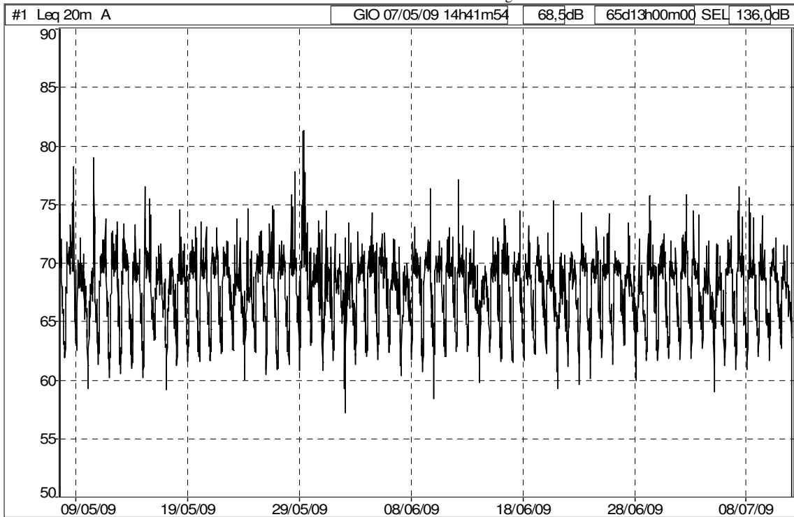
Storia temporale dal 07/05/09 al 11/07/09, sito Parking Amari (Fonte: dB TRAIT).
