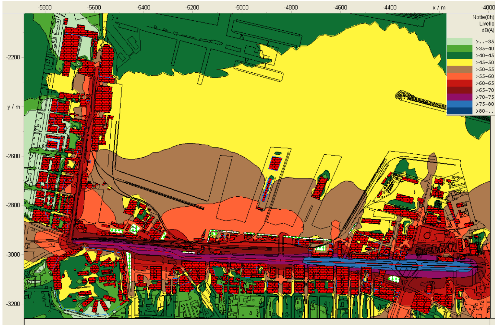
Mappa L_{night} , simulazione “ Traffico stradale ” (Fonte: IMMI).
