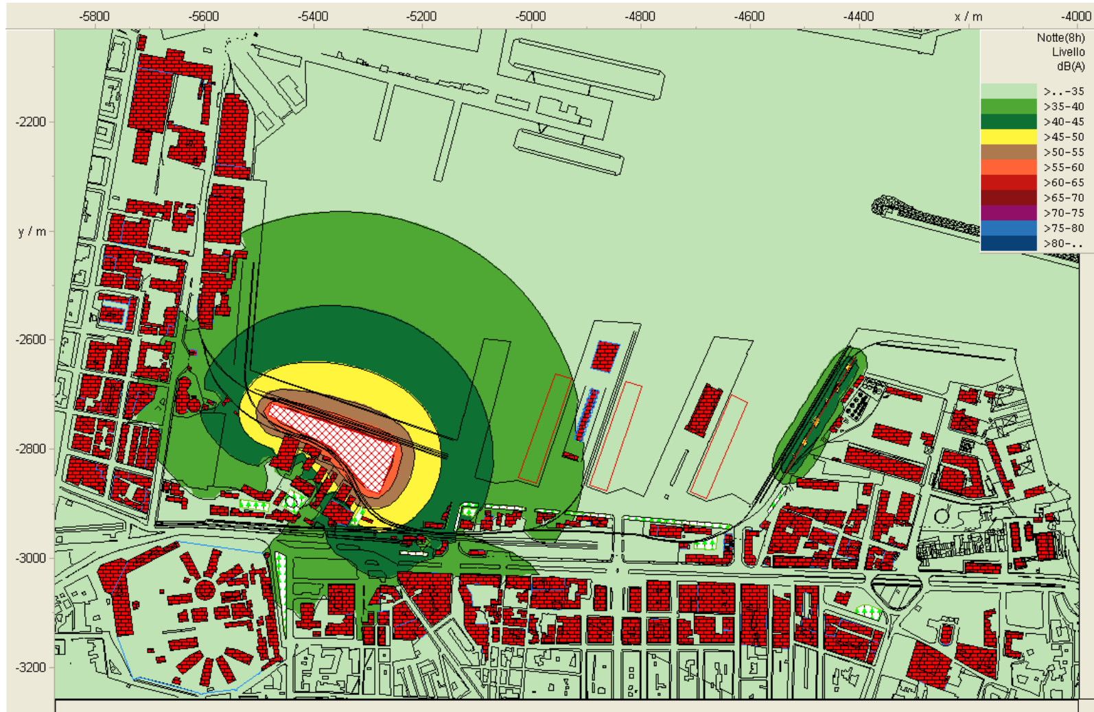
Mappa L_{night} simulazione “ Rumore portuale ” (Fonte: IMMI).
