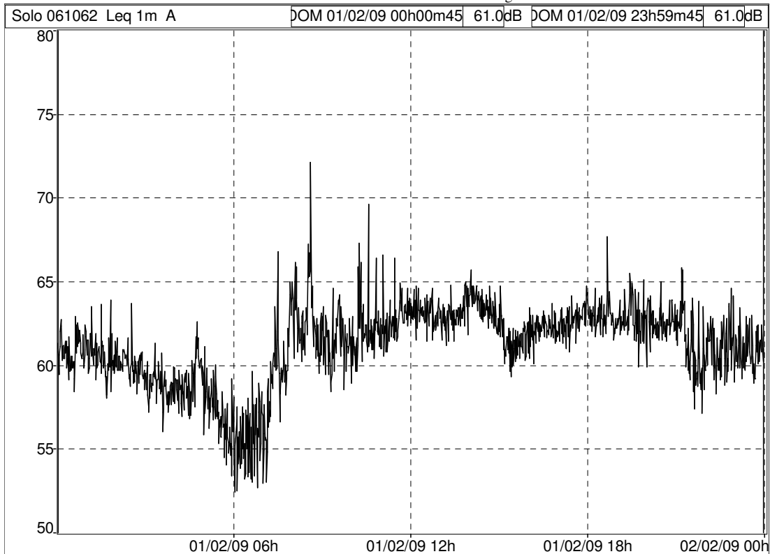
Storia temporale domenica 01/02/2009, sito Stazione Marittima (Fonte: dB TRAIT).
