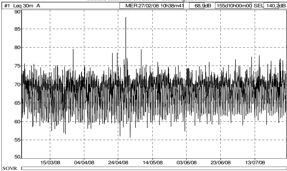
Storia temporale dal 27/02/08 al 04/11/08, sito Parking Amari (Fonte: dB TRAIT).
