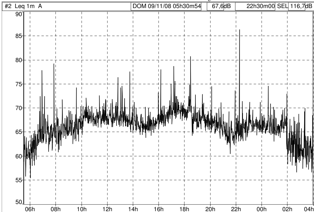
Storia temporale domenica, sito Parcheggio (Fonte: dB TRAIT).
