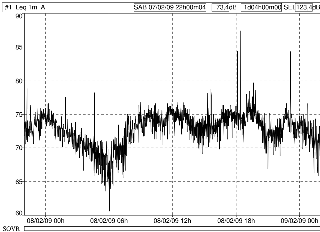
Storia temporale giornaliera domenica, sito via Crispi 120 (Fonte: dB TRAIT).
