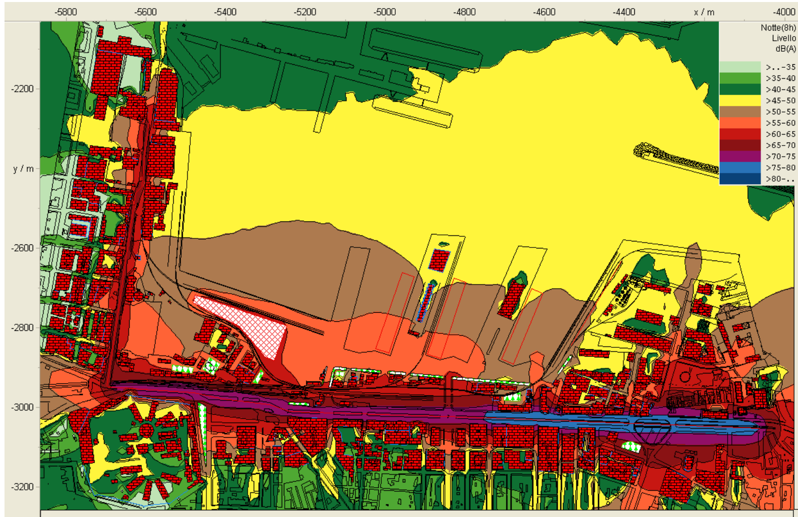
Mappa L_{\text{night}} simulazione “ Stato acustico reale ” (Fonte: IMMI).
