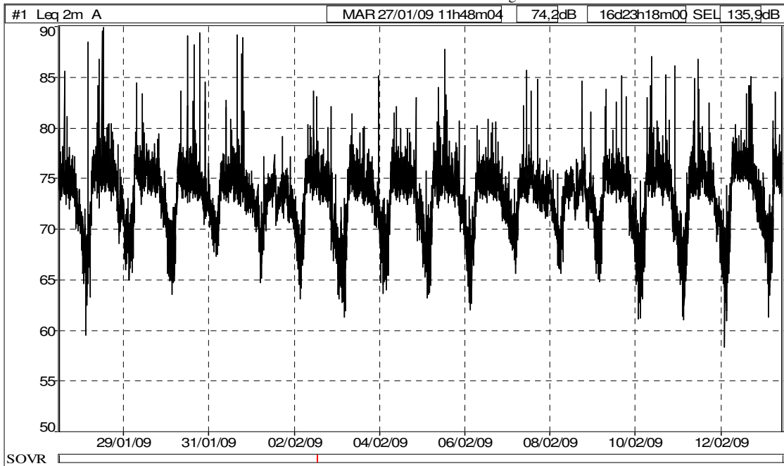
Storia temporale sito via Crispi 120 (Fonte: dB TRAIT).
