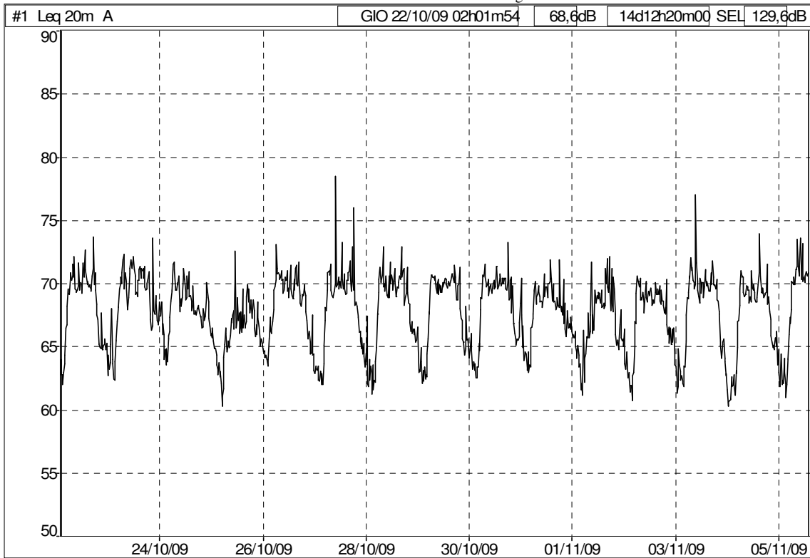
Storia temporale dal 02/10/09 al 17/10/09, sito Parking Amari (Fonte: dB TRAIT).
