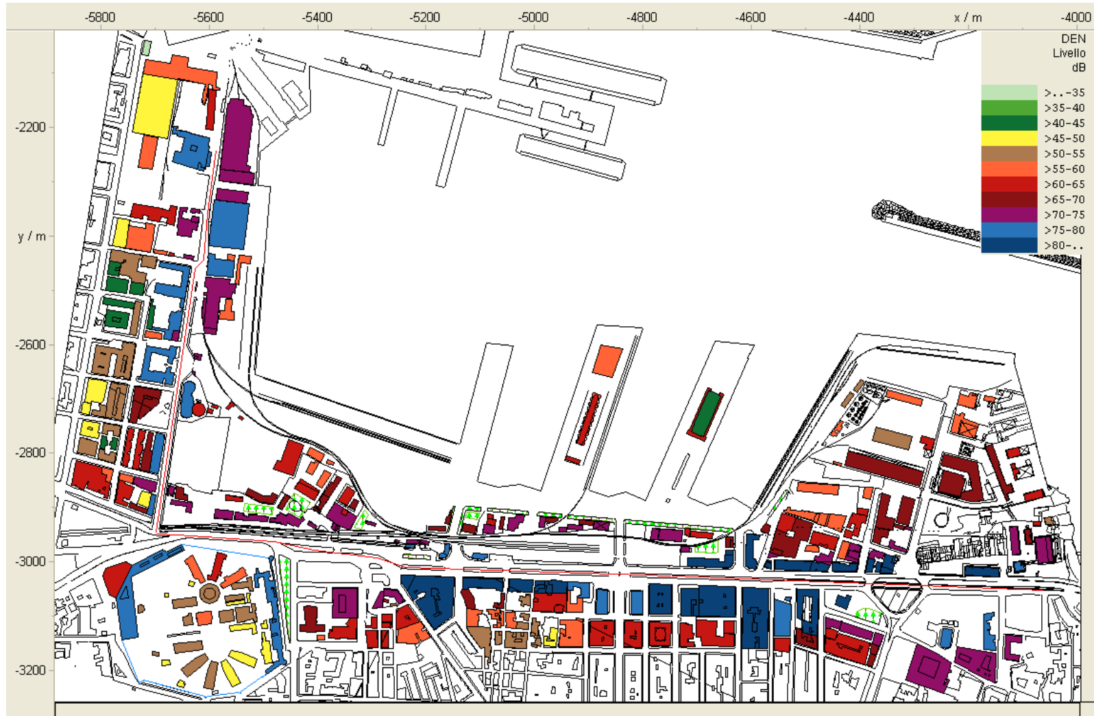
Mappa L DEN , livelli di facciata, simulazione "Traffico stradale" (Fonte: IMMI).
