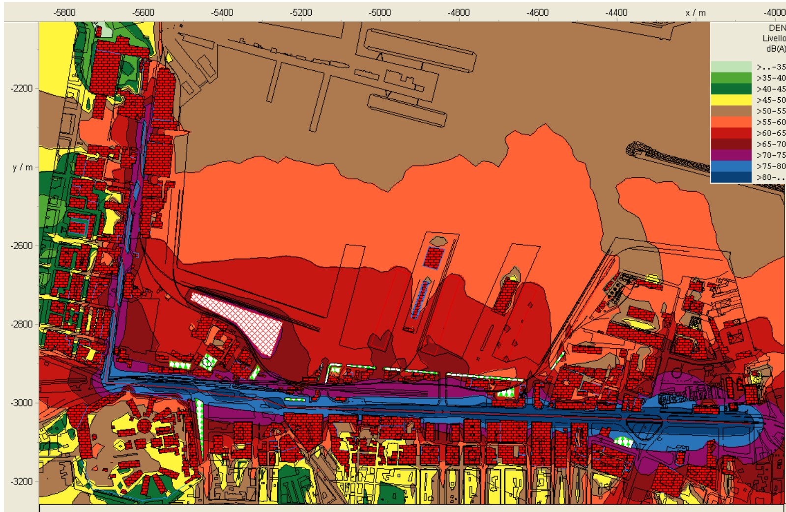
Mappa L den simulazione “ Stato acustico reale ” (Fonte: IMMI).
