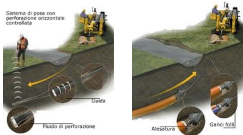
Figura 20 - Esempio tipo della tecnologia TOC-Trivellazione Orizzontale Controllata
