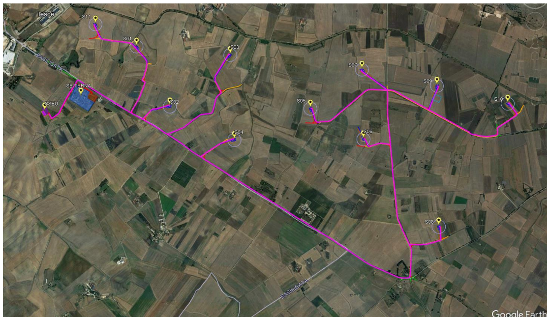
Figura 1 - Individuazione del layout di impianto su Ortofoto
