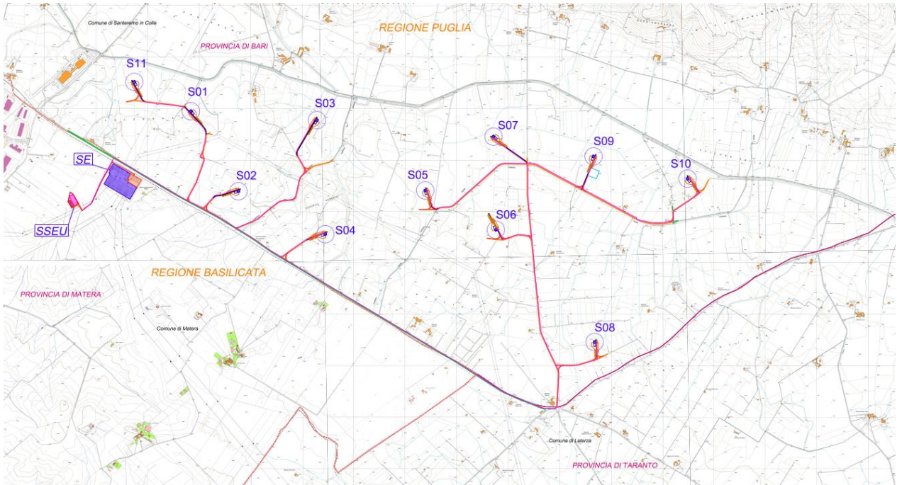
Figura 3 - Inquadramento impianto eolico su CTR
