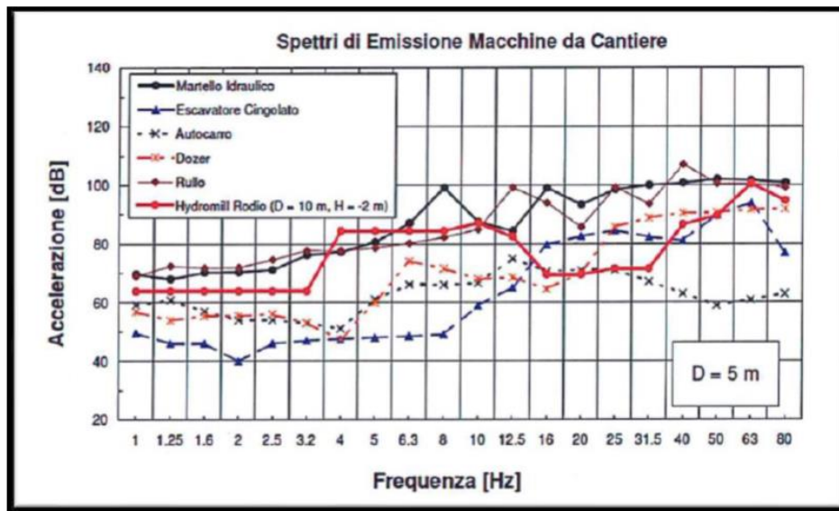
Figura 29 - Spettro emissioni tipo delle macchine da cantiere
