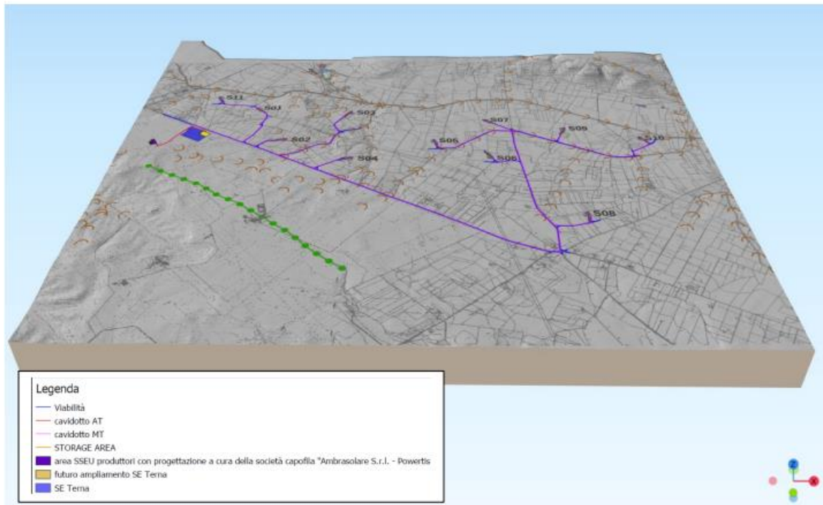
Figura 21 – Immagina rappresentativa delle strutture geomorfologiche presenti su base DEM
