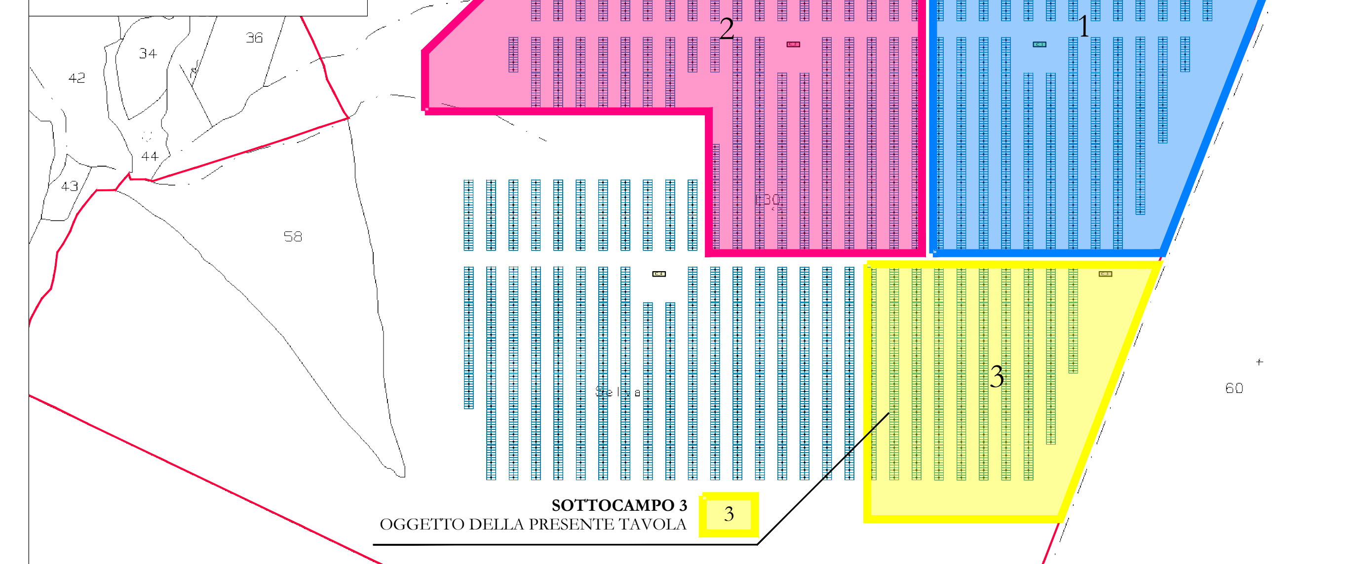
Planimetria generale con indicazione delle sezioni elettriche AREA 1 - scala 1:2.000
