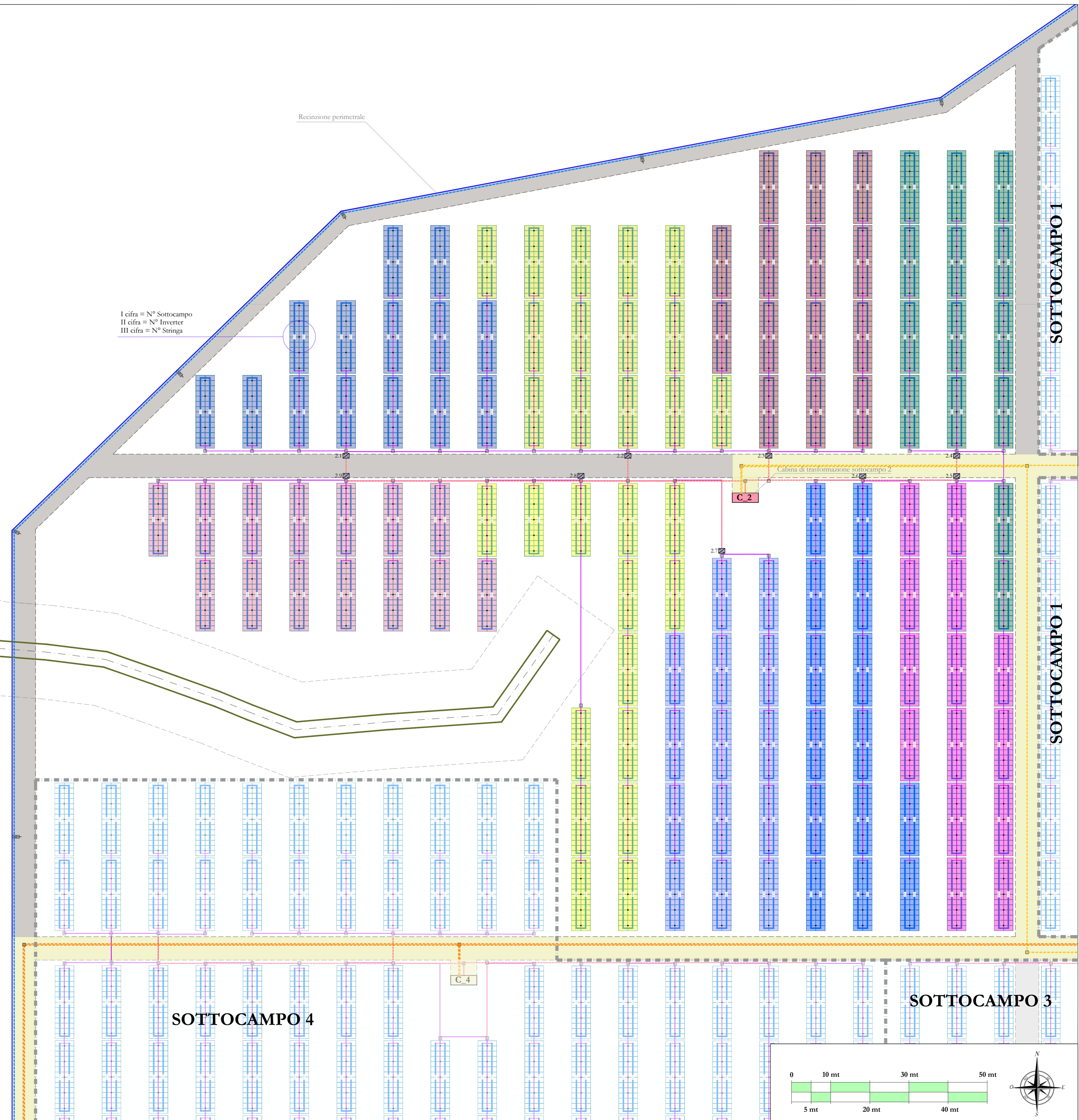
Planimetrica generale con indicazione delle sezioni elettriche AREA 1 - scala 1:2000
