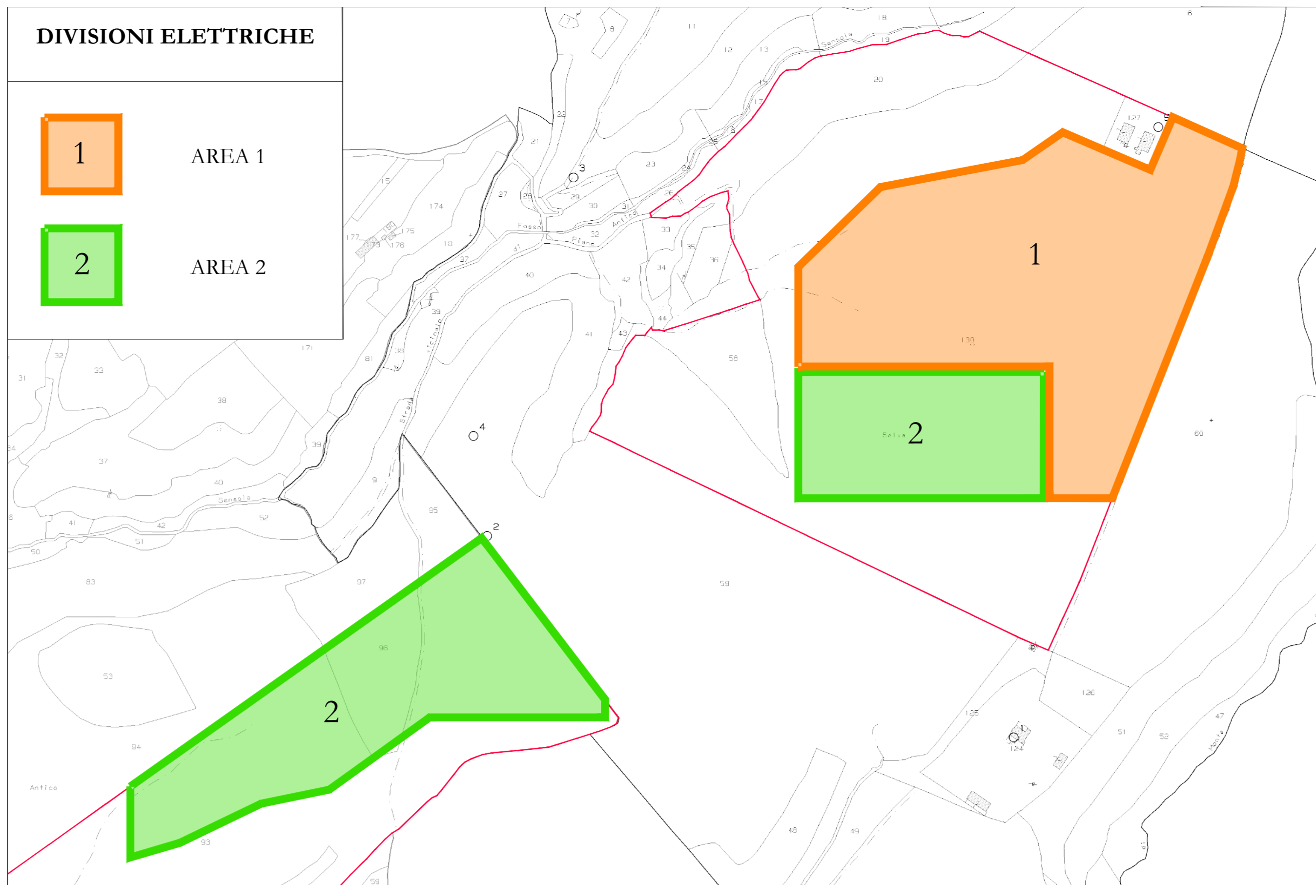
Planimetrica generale con indicazione delle sezioni elettriche - scala 1:4000
