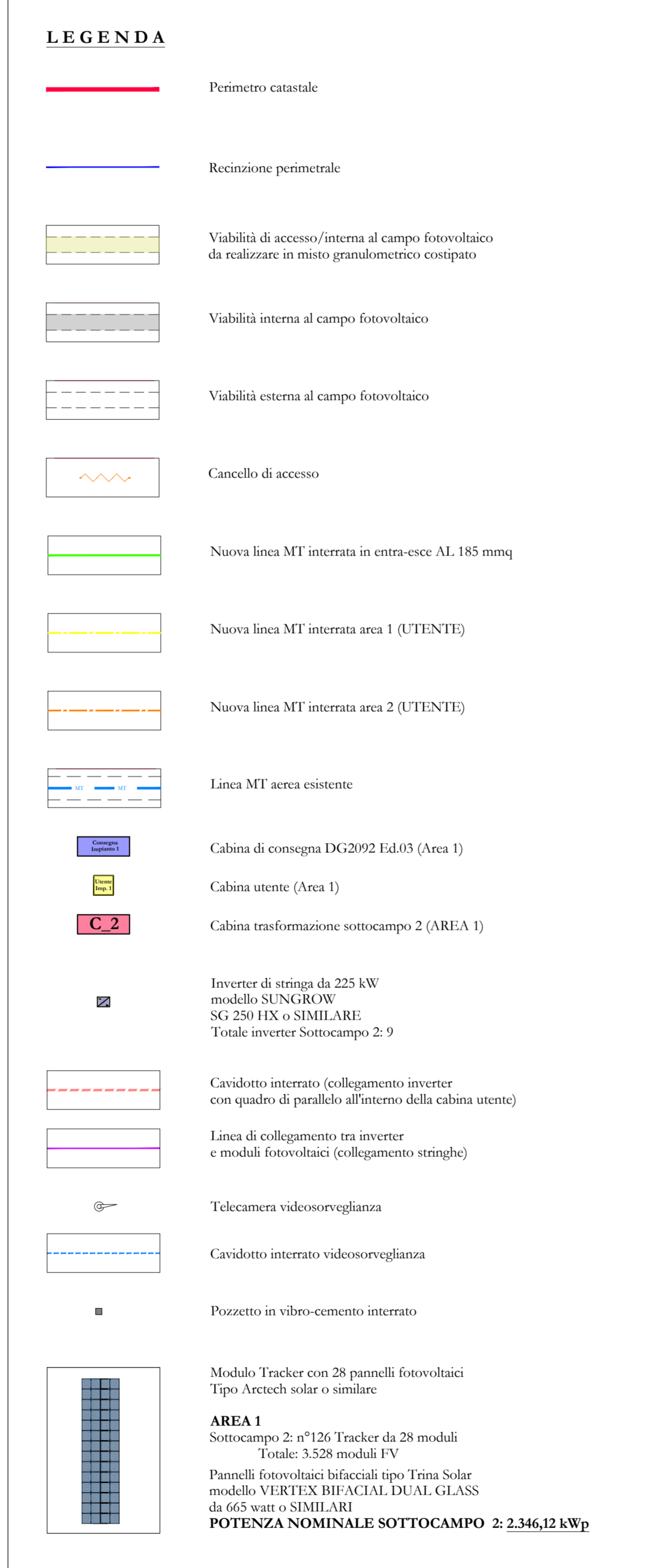
Planimetrica generale con indicazione delle sezioni elettriche - scala 1:4000
