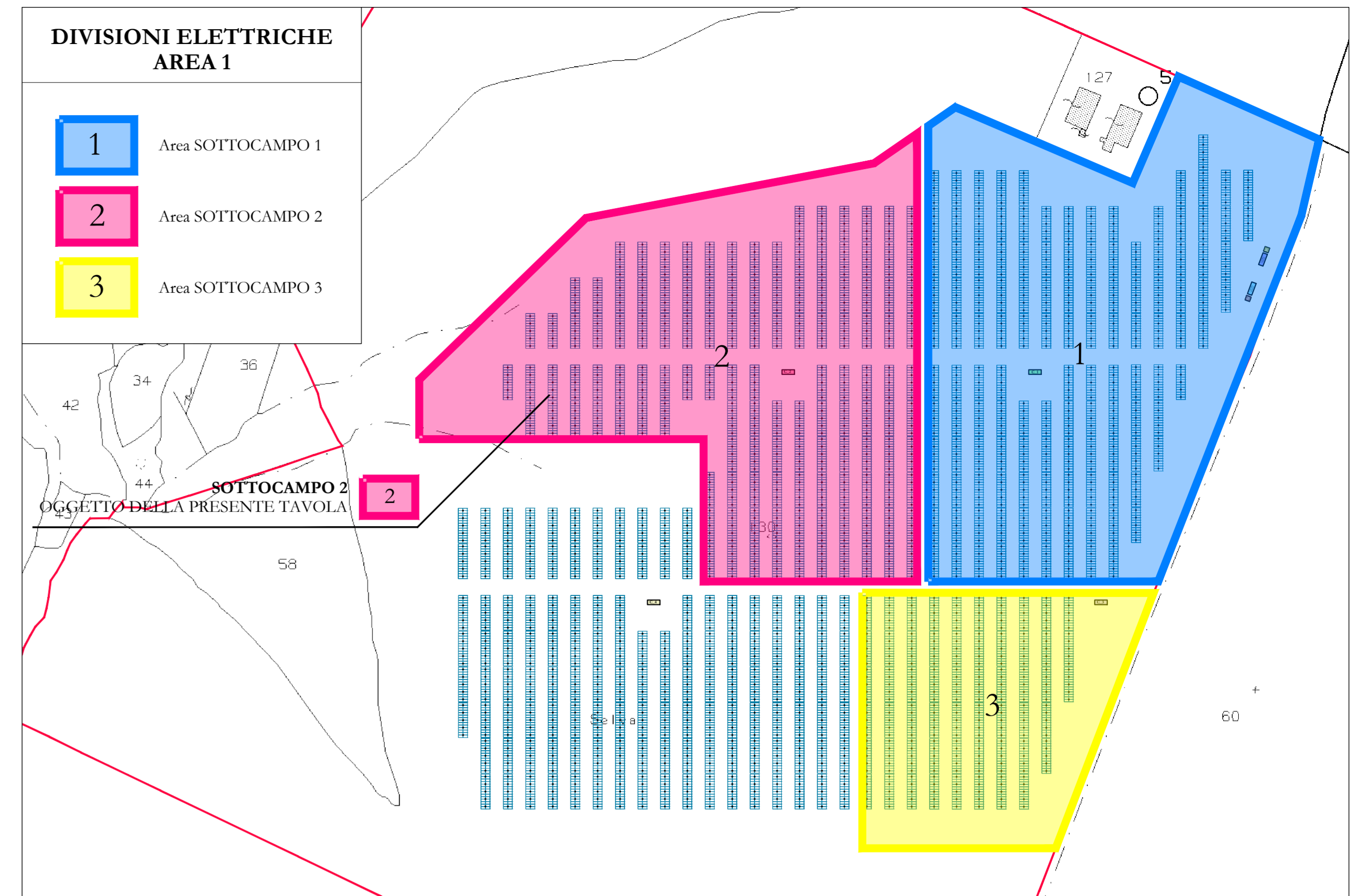
Planimetrica generale con indicazione delle sezioni elettriche AREA 1 - scala 1:2000
