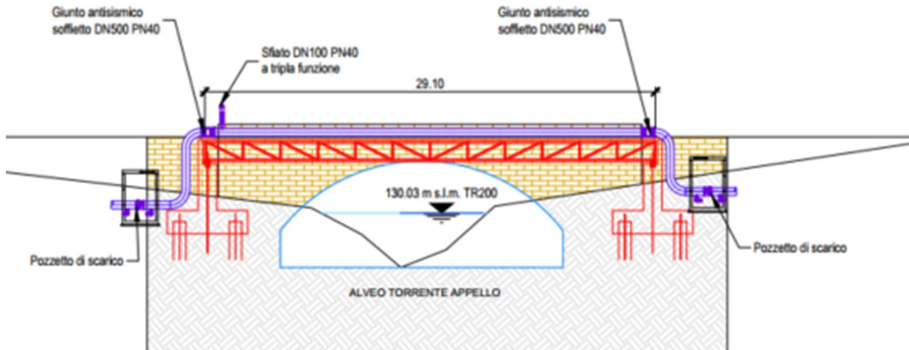
Figura 2 – Prospetto opera di attraversamento sull' Appello in progetto.
