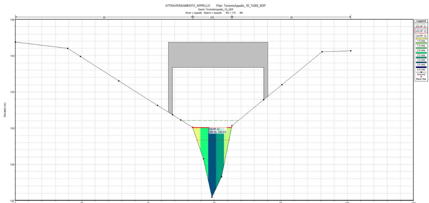
Figura 11 : Sezione 175 BR U – Modello 1D stato di progetto
