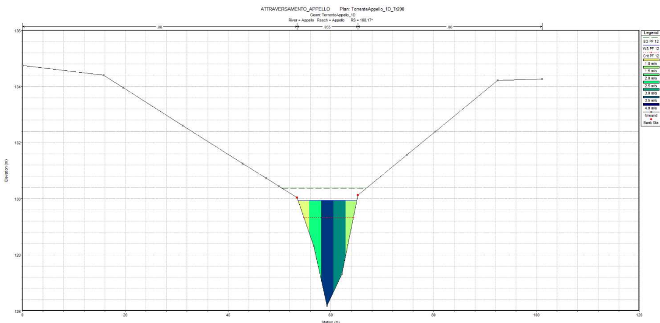
Figura 10 – Sezione 178 di attraversamento – Modello 1D stato di fatto.
