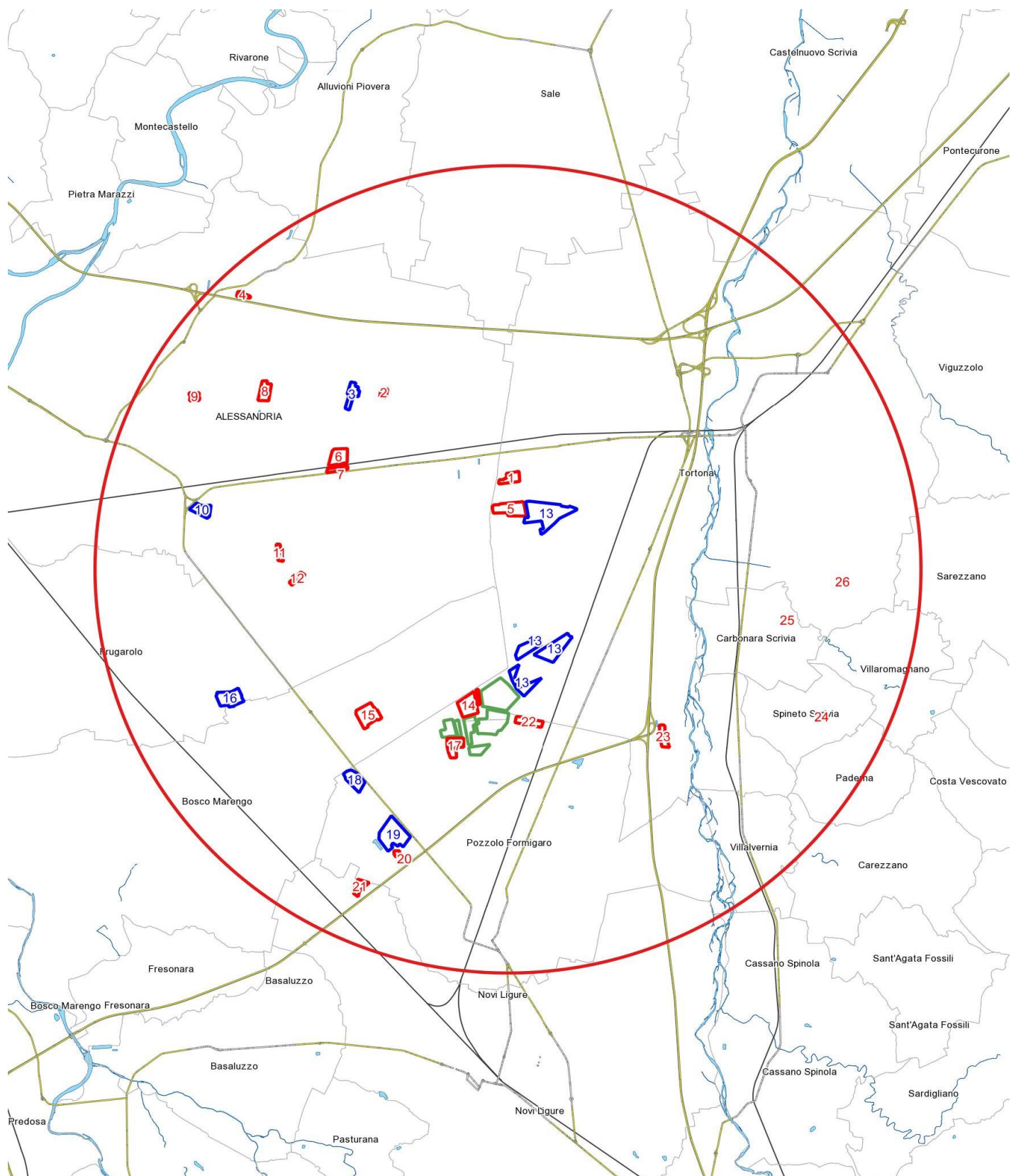
Figura 19: Inquadramento degli impianti fotovoltaici presenti nel raggio di 10 km dall'impianto agrovoltaico Margisolar
