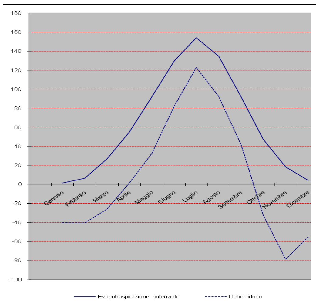
Figura 11: Evapotraspirazione e deficit idrico
