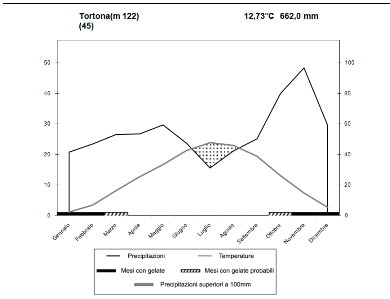
Figura 10: Climodiagramma secondo Walters e Lieth
