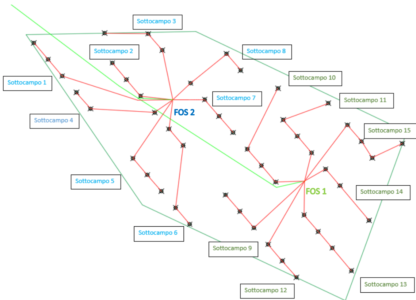
Figura 4 - Struttura del parco eolico con indicazione dei sottocampi e delle stazioni Off-Shore
