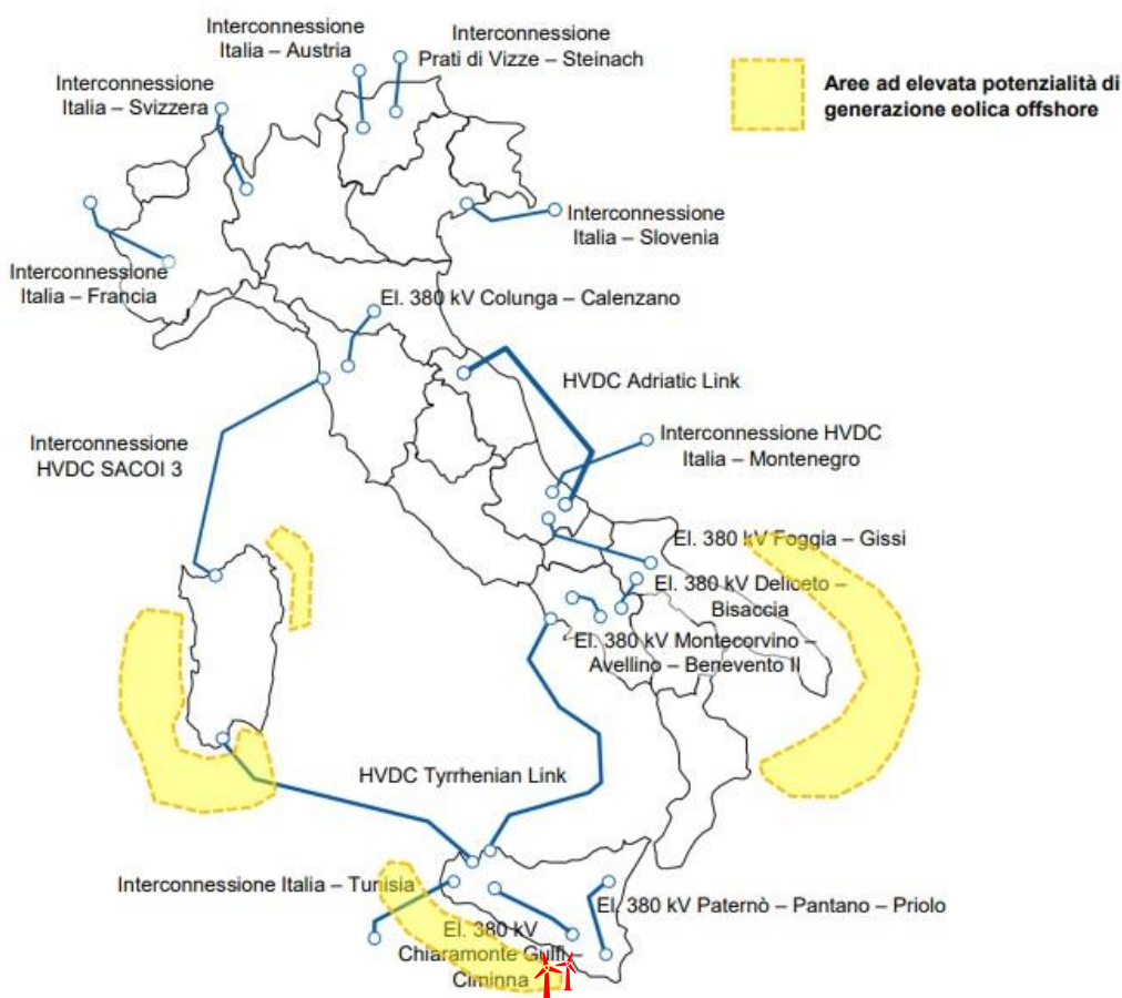
Figura 1 - Aree ad elevata potenzialità di generazione eolica off-shore, fonte Terna Spa
