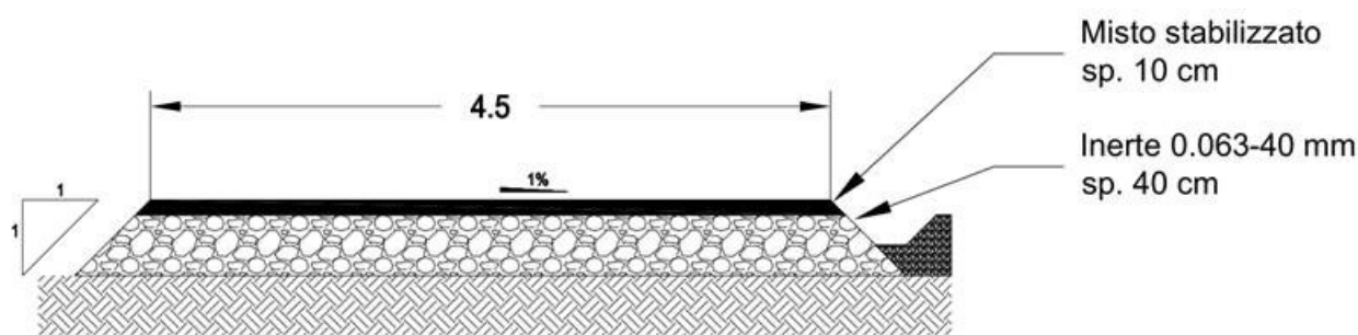
Figura 2: sezione tipo
