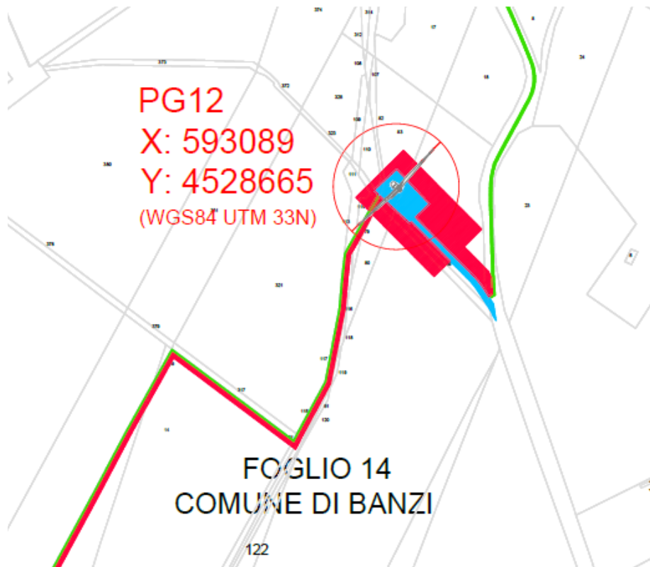
Figura 5 – Dettaglio strade di accesso-aree provvisorie e definitive
