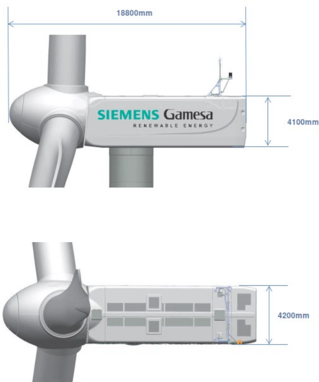
Figura 8 – Rappresentazione navicella Siemens Gamesa SG 4.7 – 155
