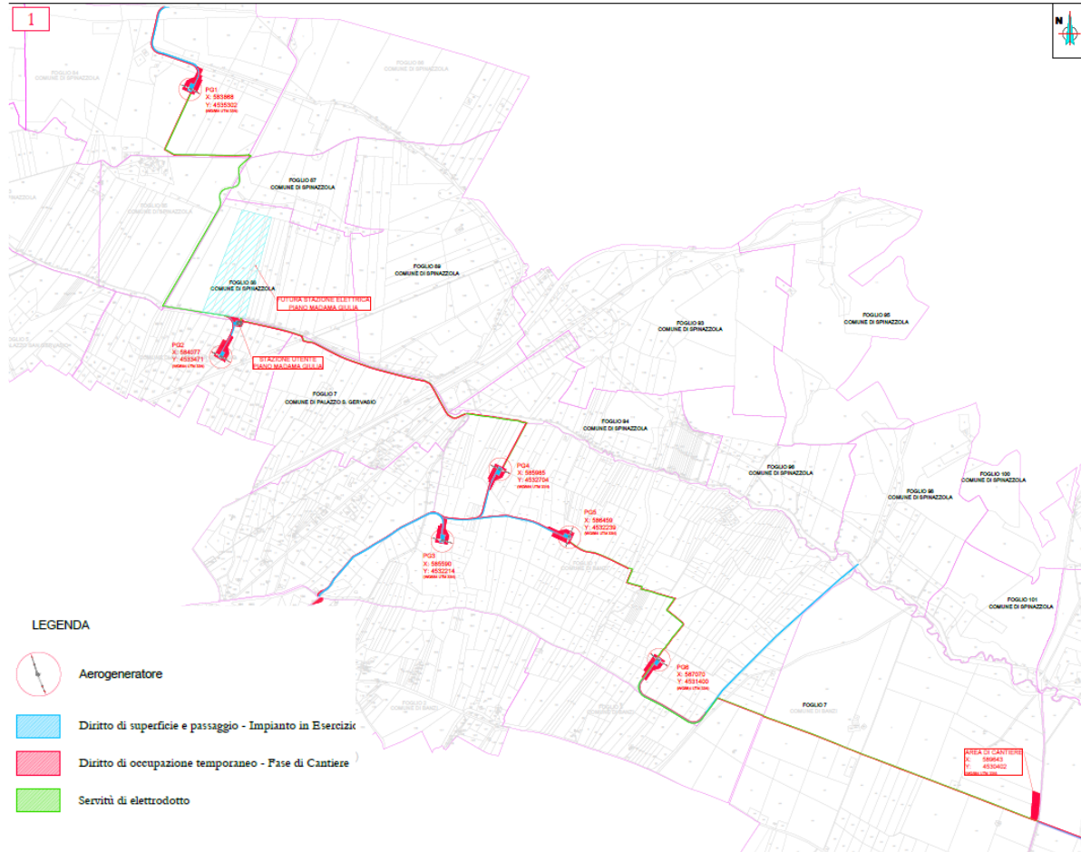
Figura 3 - Rappresentazione grafica generale aree di occupazione e servitù (1/2)
