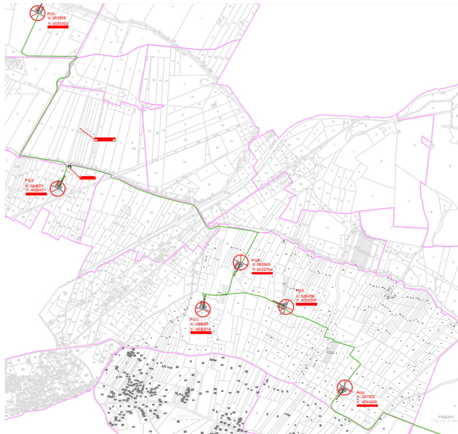
Figura 10 – Rappresentazione grafica generale del cavidotto (2/2)
