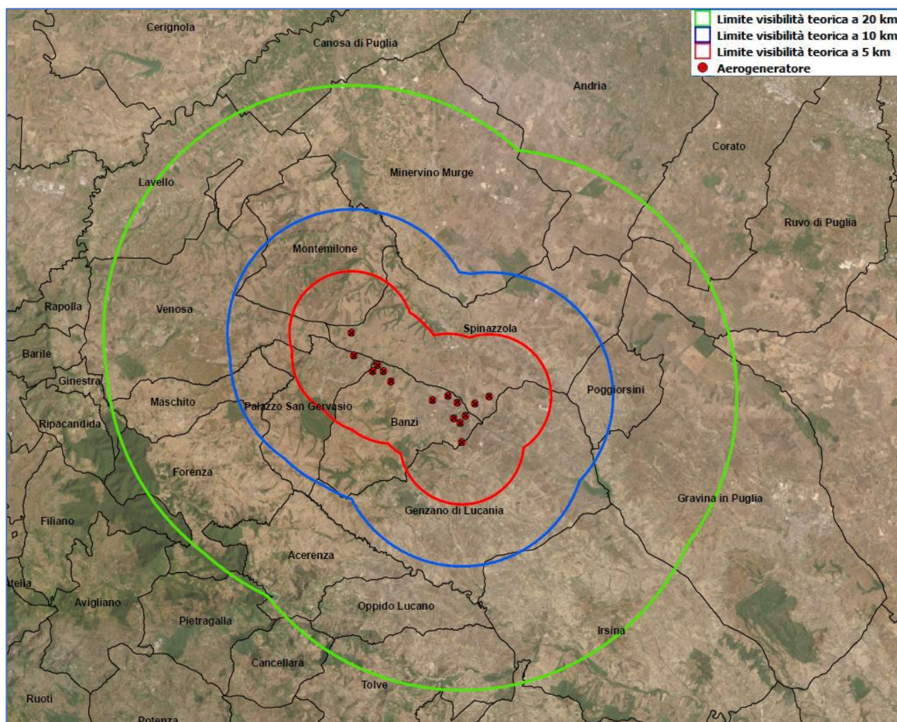
Figura 1 - Inquadramento area di impianto con aree di visibilità teorica a 20km, 10km e 5 km
