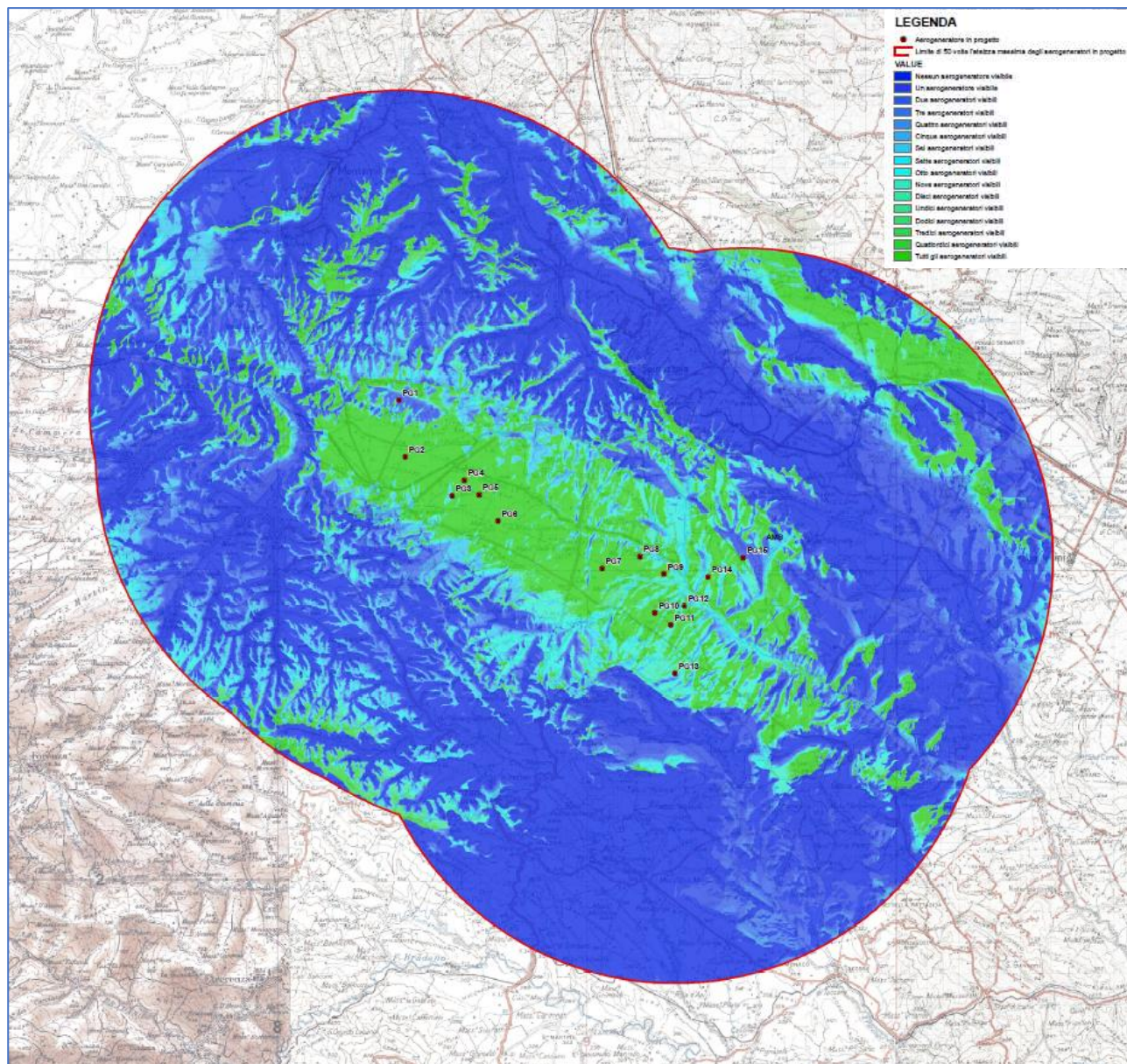
Figura 3 - Mappa dell'intervisibilità degli aerogeneratori - metodo 1
