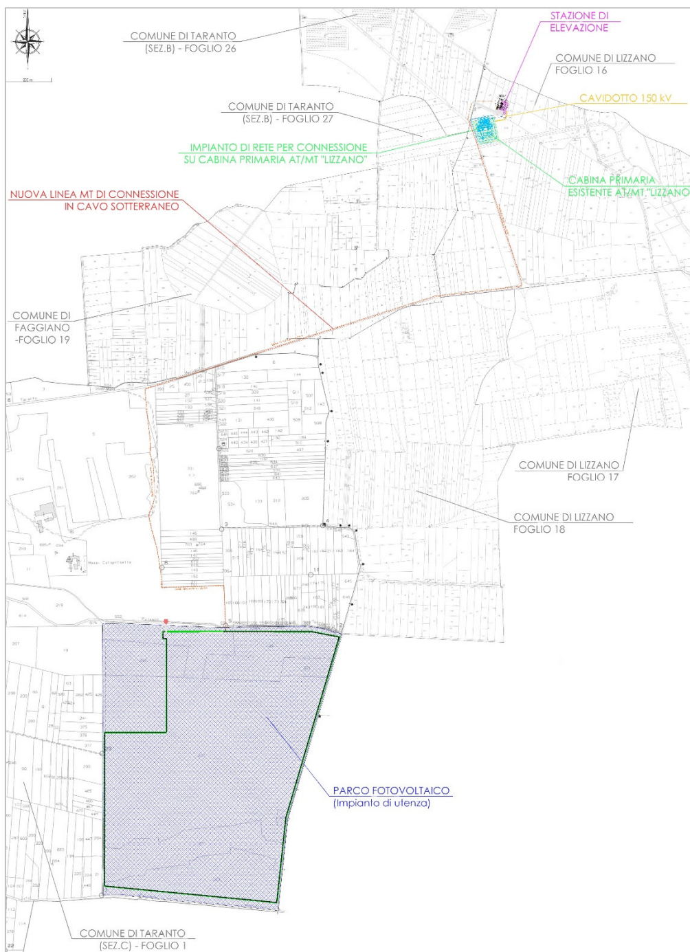
Figura 14: Tracciato del cavidotto a 30 kV (in arancio) da "Calapricello" a Stazione di Elevazione
