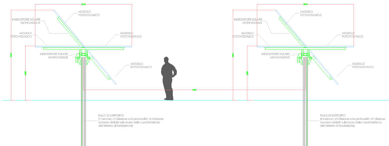
Figura 9: Sezione trasversale inseguitori monoassiali
