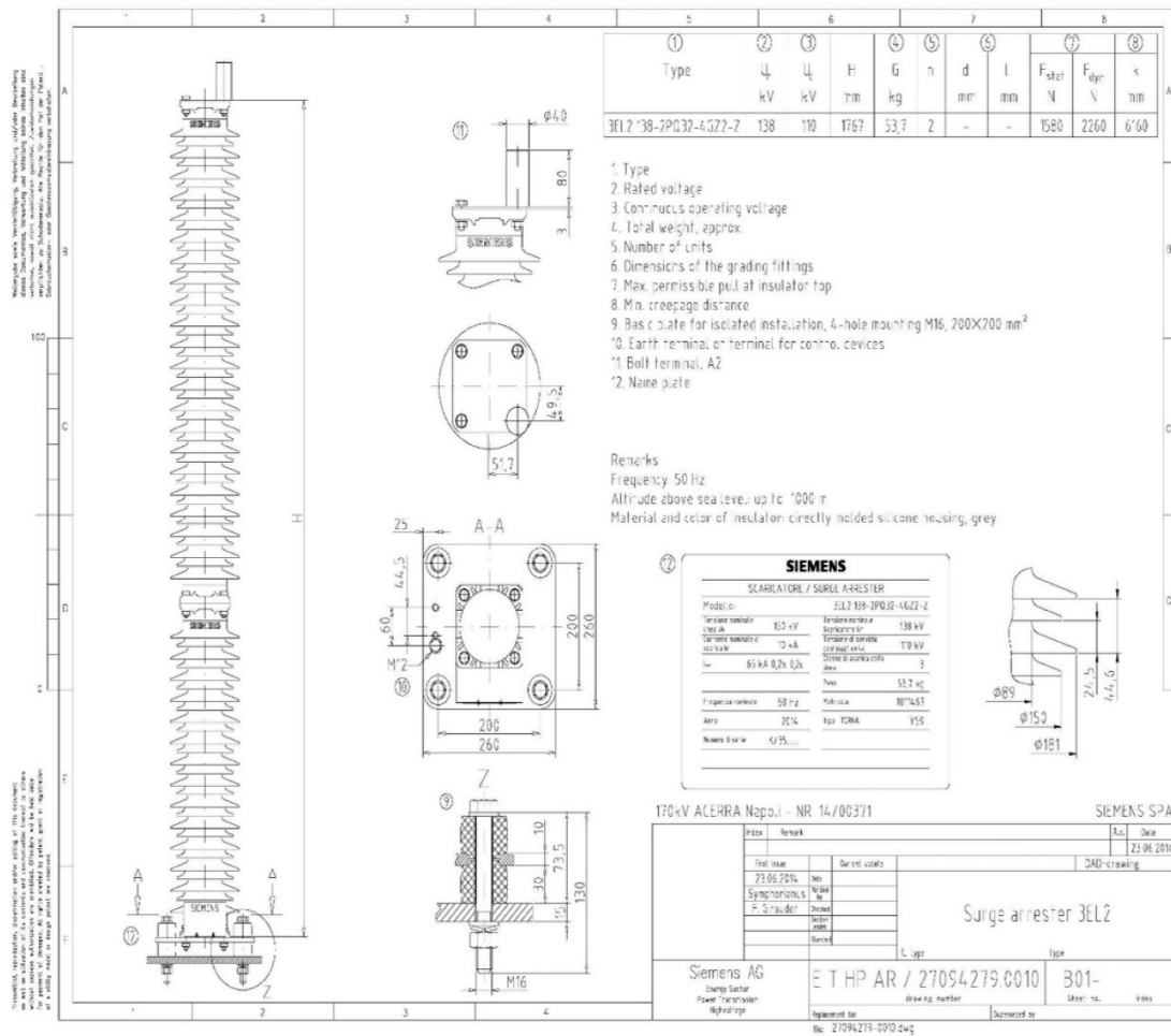
Figura 20: Scaricatori
