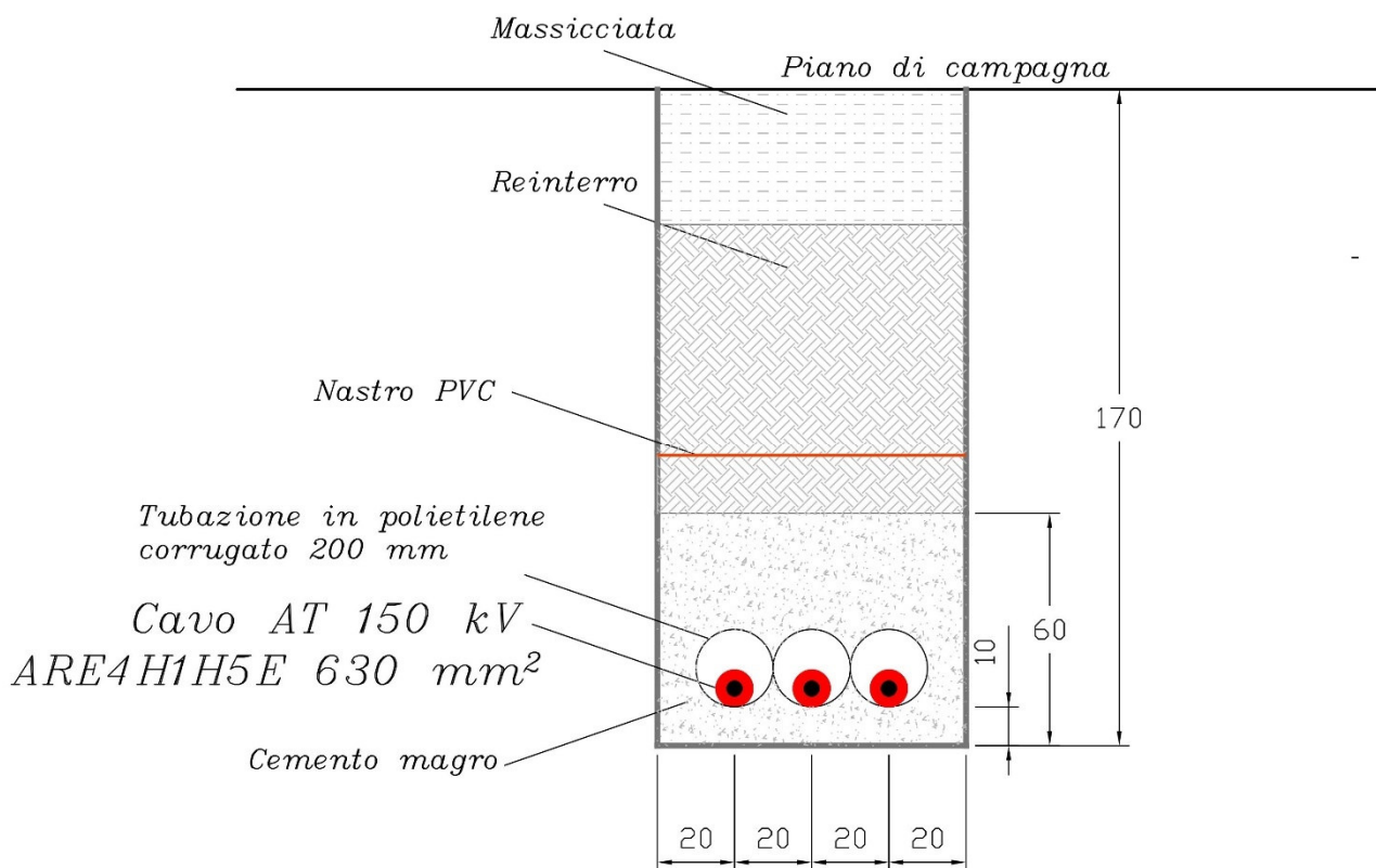
Figura 21: Tipico modalità di posa cavo 150 kV
