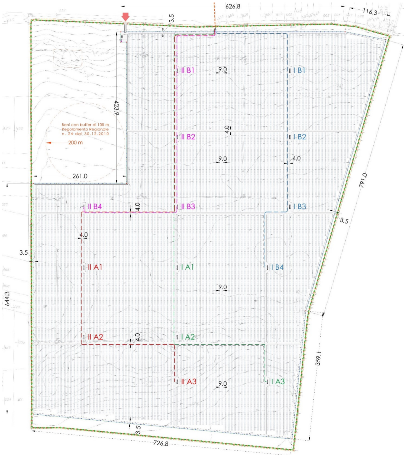
Figura 3: Layout dell'impianto di generazione fotovoltaica
