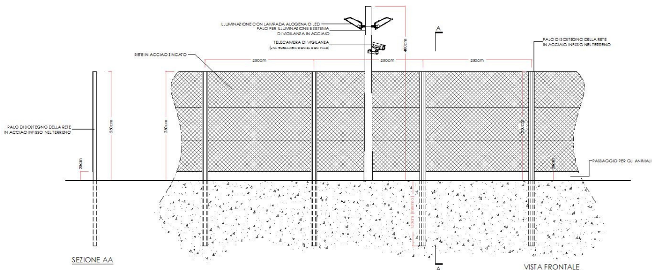
Figura 10: Dettaglio frontale della recinzione perimetrale.
