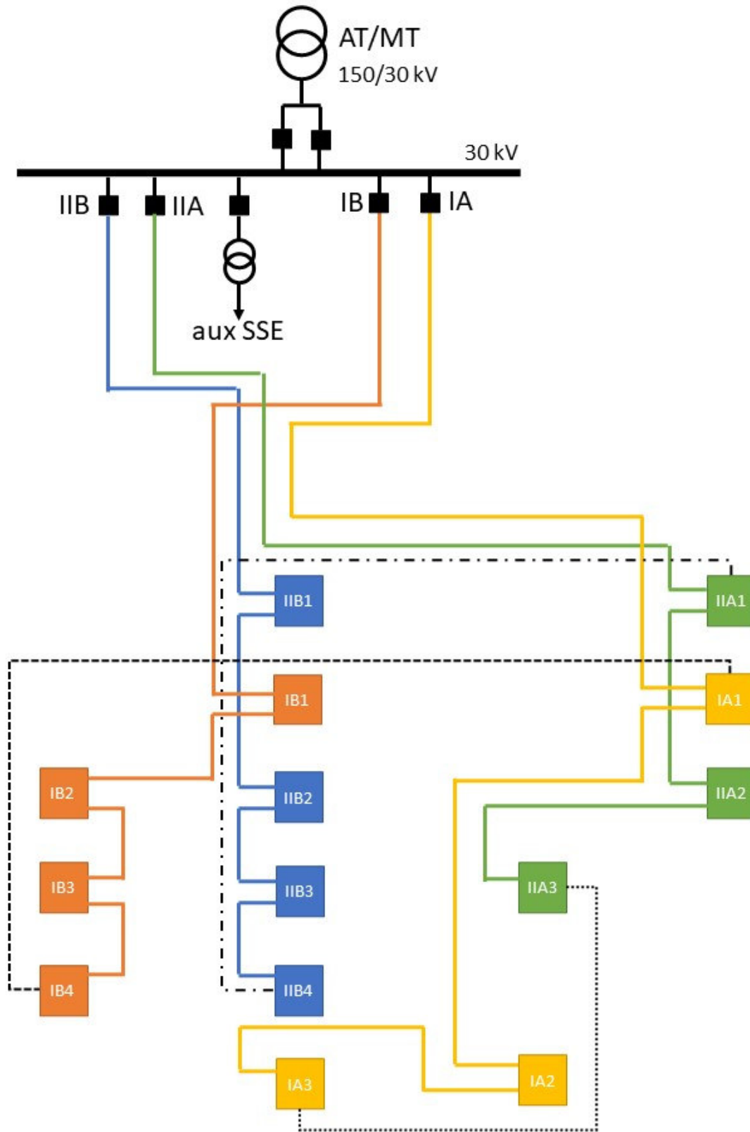
Figura 4: Sistema di distribuzione MT
