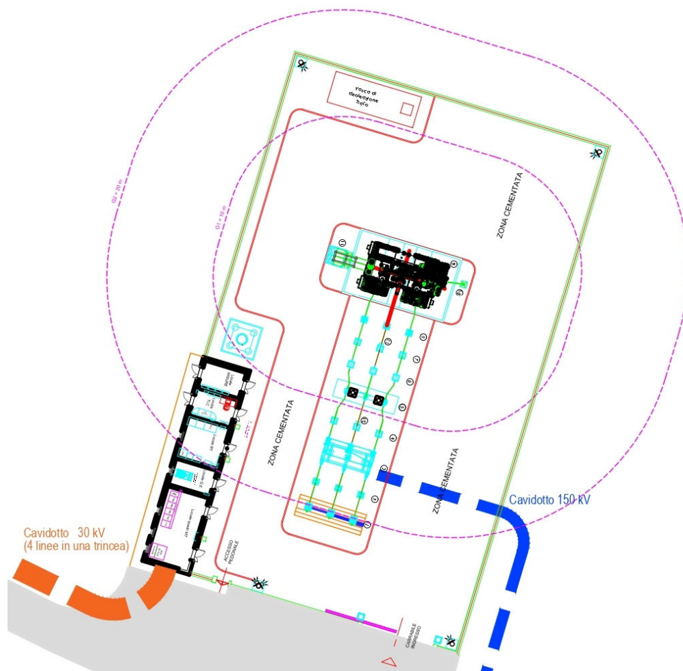
Figura 15: Disposizione elettromeccanica Stazione di Trasformazione Step-Up 150/30 kV
