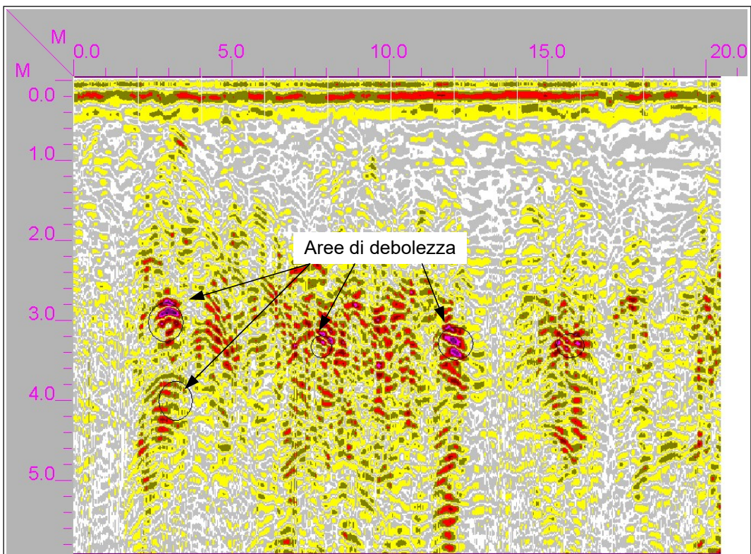
Figura 19 - Sezione 10
