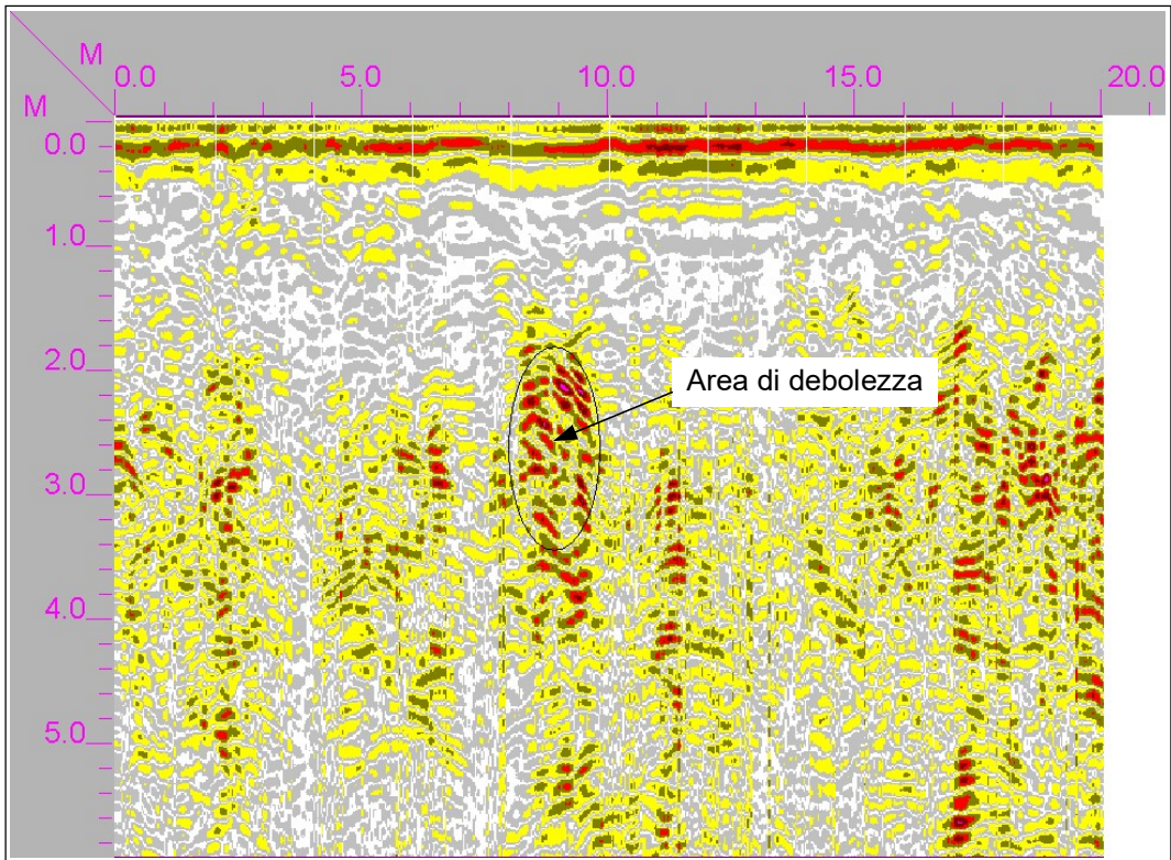
Figura 18 - Sezione 9
