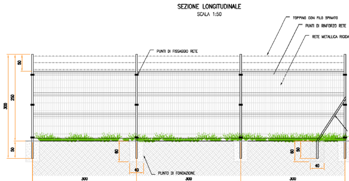
Figura 4.5: Particolare recinzione
