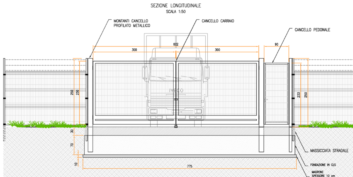
Figura 4.7: Particolare accesso
