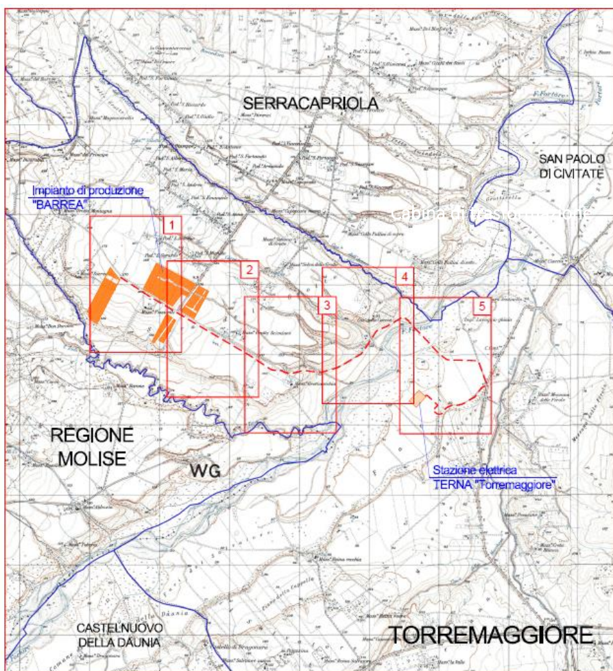
Figura 4.8: In rosso il percorso di connessione dal campo FV alla stazione elettrica.
