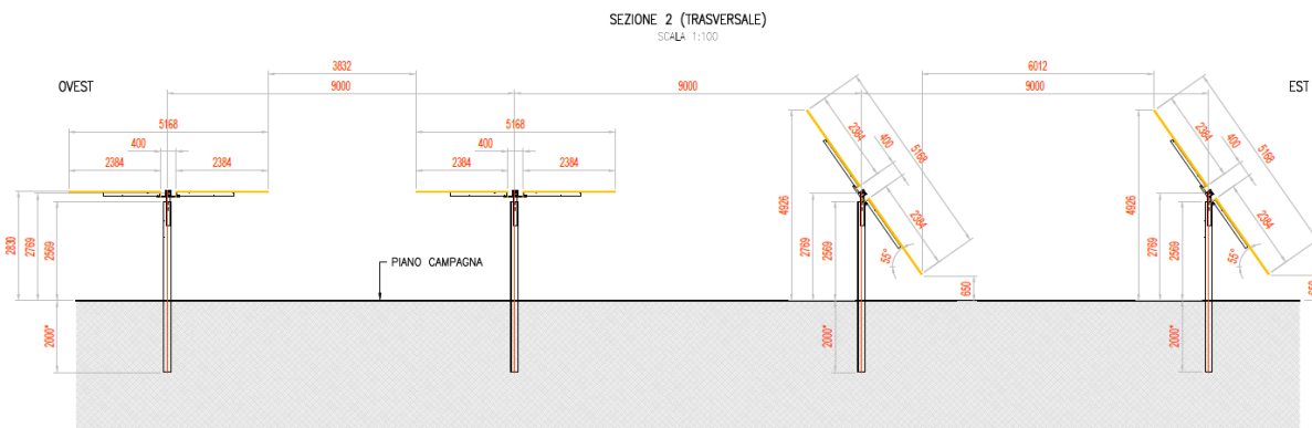
Figura 4.4: Particolare strutture di sostegno moduli
