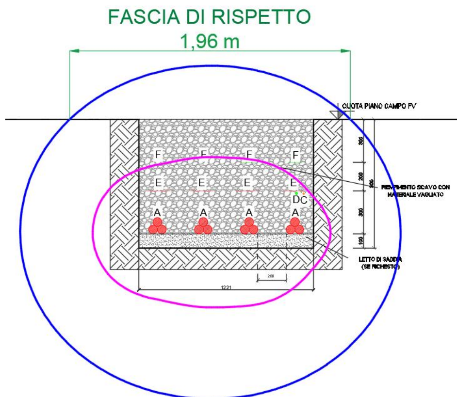
Figura 8: Curve Equicampo - 4 Terne di cavi MT su strada sterrata - Interno Impianto FV
