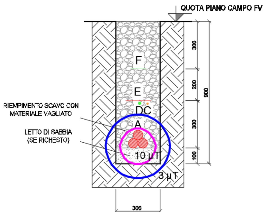
Figura 4: Curve Equicampo - 1 Terna di cavi MT su strada sterrata - Interno Impianto FV
