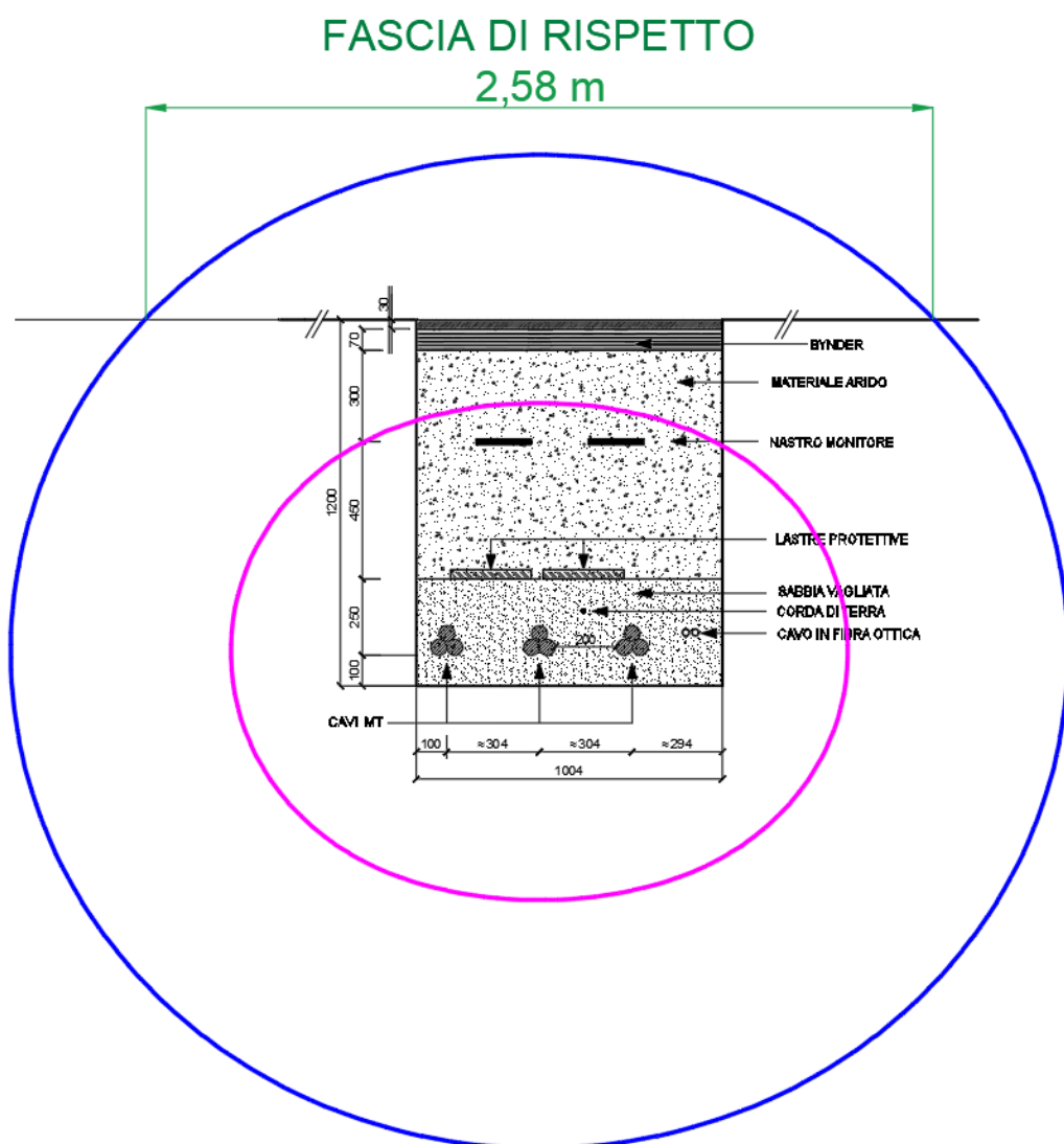
Figura 9: Curve Equicampo - 3 Terne di cavi MT su strada asfaltata – Interconnessione Impianto FV con SSU
