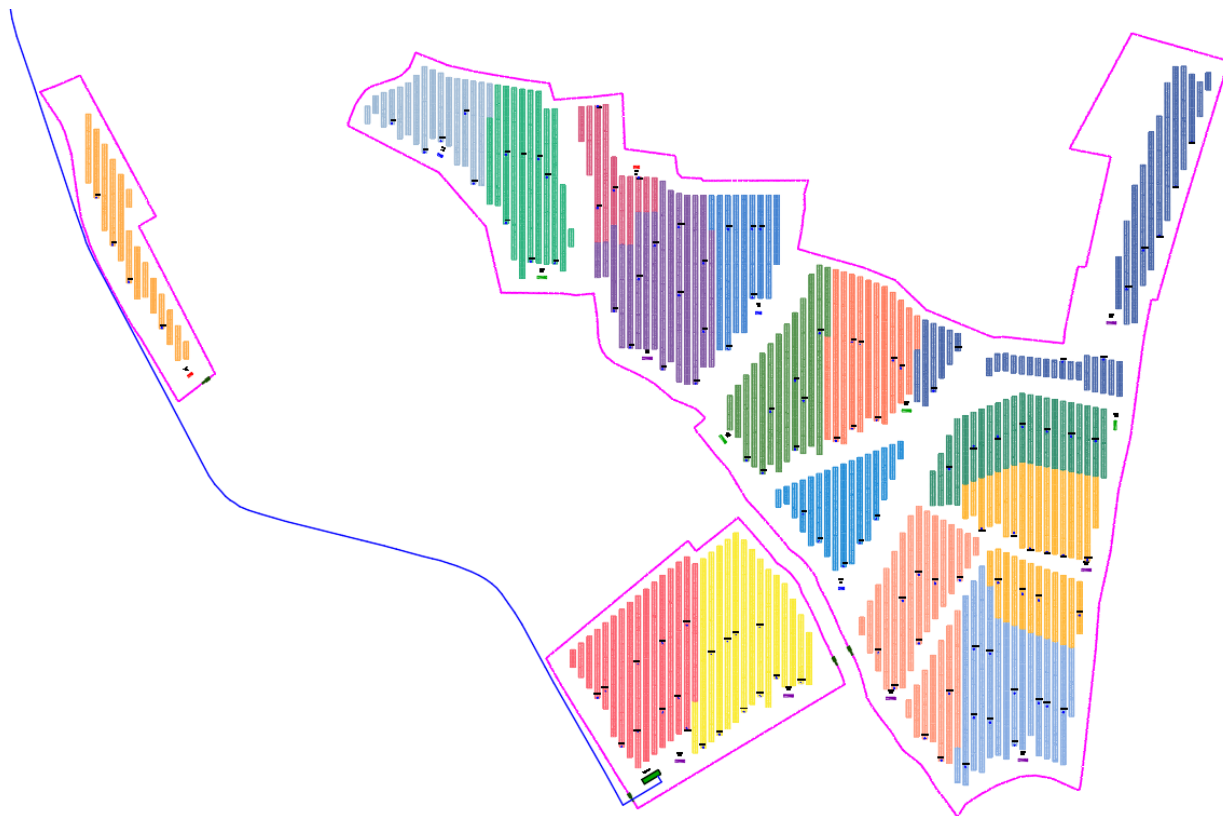
Figura 2 Layout d'impianto
