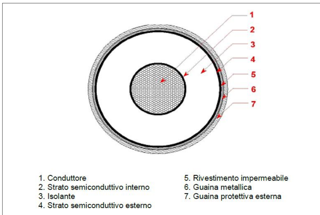
Figura 18 - Sezione tipo cavo AT.
