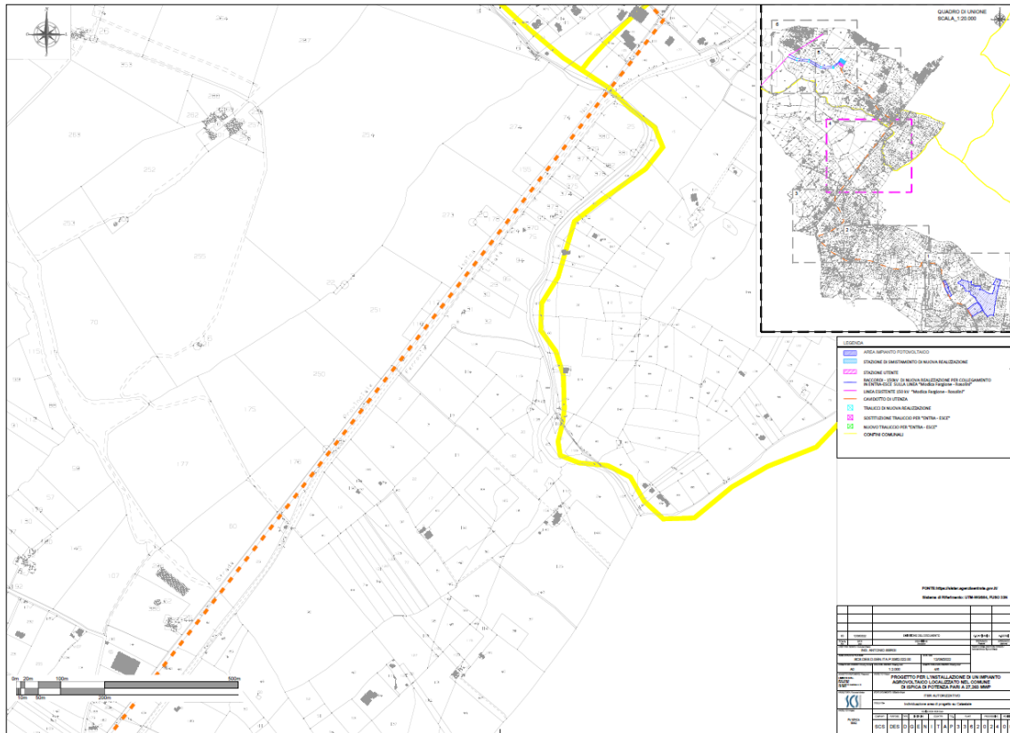
Figura 6: Stralcio 4 da planimetria catastale - percorso cavidotto MT
