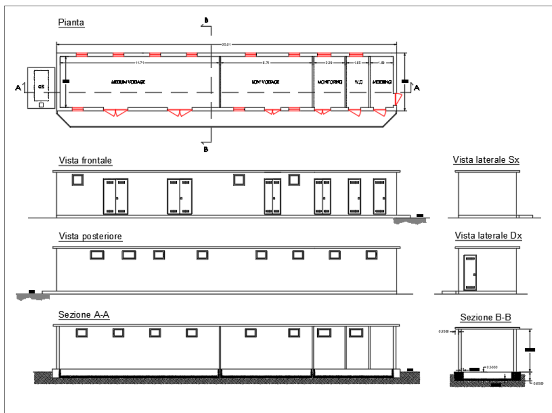
Figura 15 - Edificio interno alla SSU.
