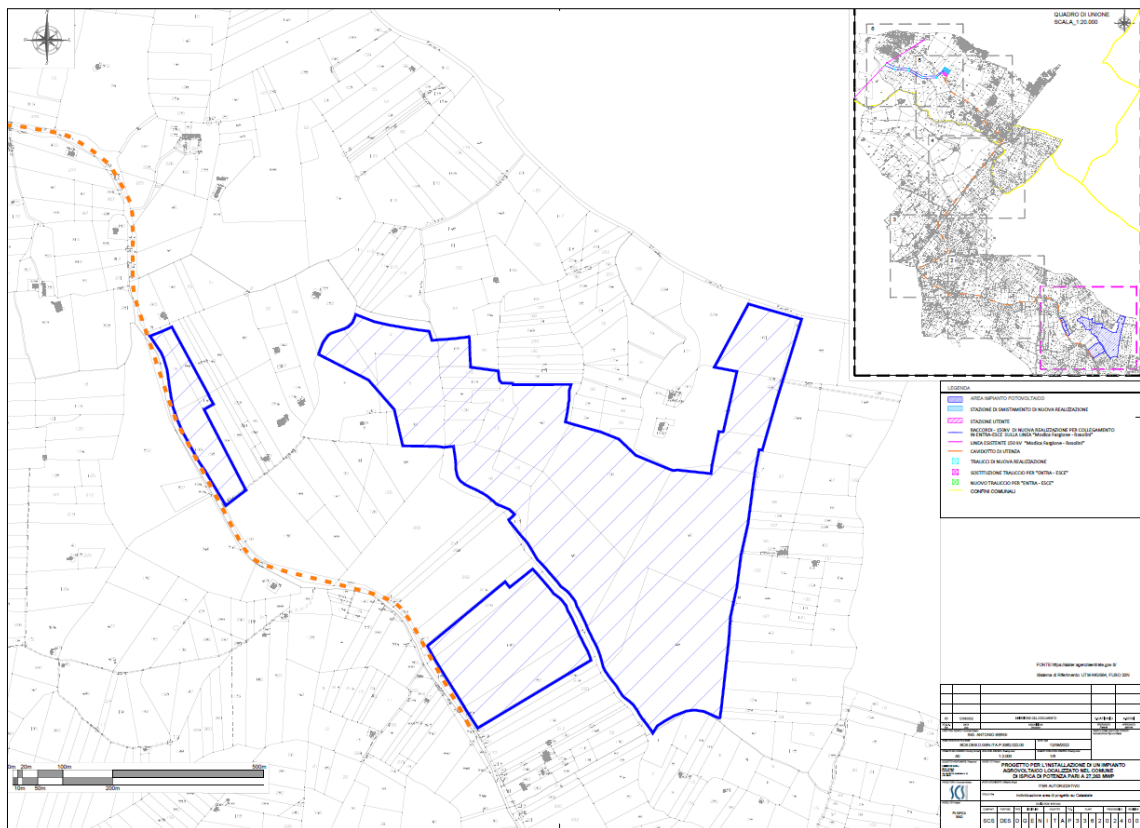
Figura 3: Stralcio 1 da planimetria catastale - percorso cavidotto MT
