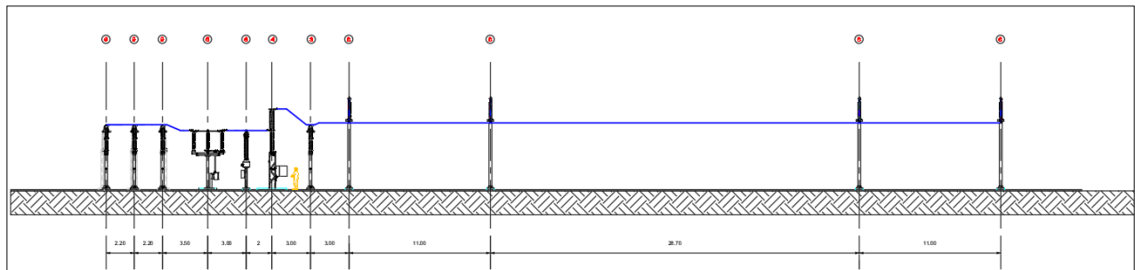
Figura 12 - Stallo di trasformazione LIMES 28 S.r.l.
