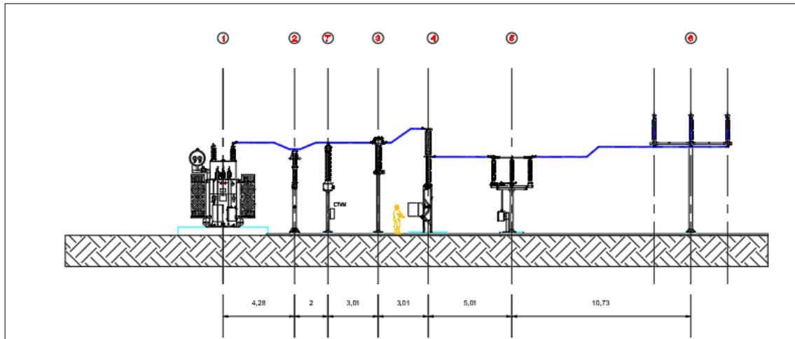
Figura 12 - Stallo di trasformazione LIMES 28 S.r.l.
