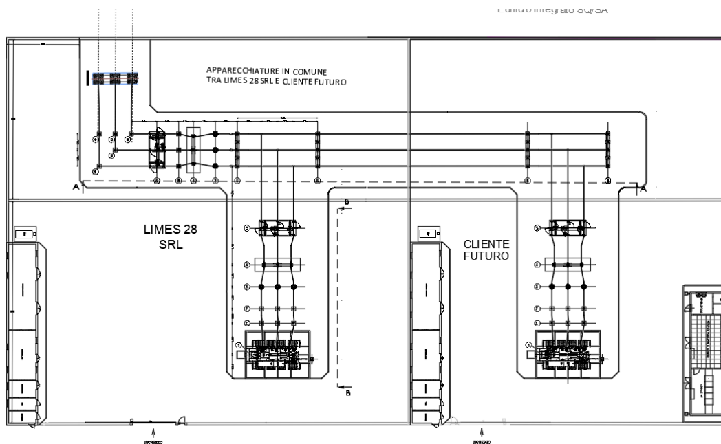
Figura 11 - Area sottostazione LIMES 28 S.r.l.
