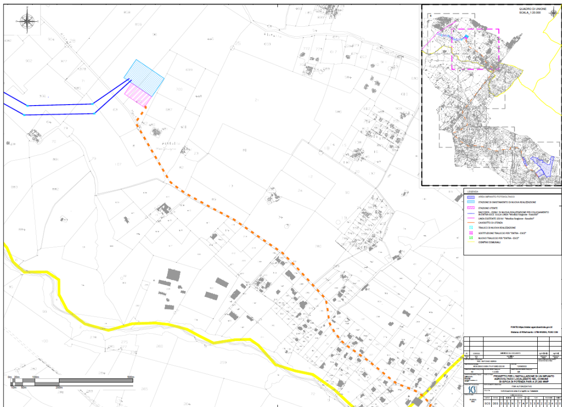
Figura 7: Stralcio 4 da planimetria catastale - percorso cavidotto MT
