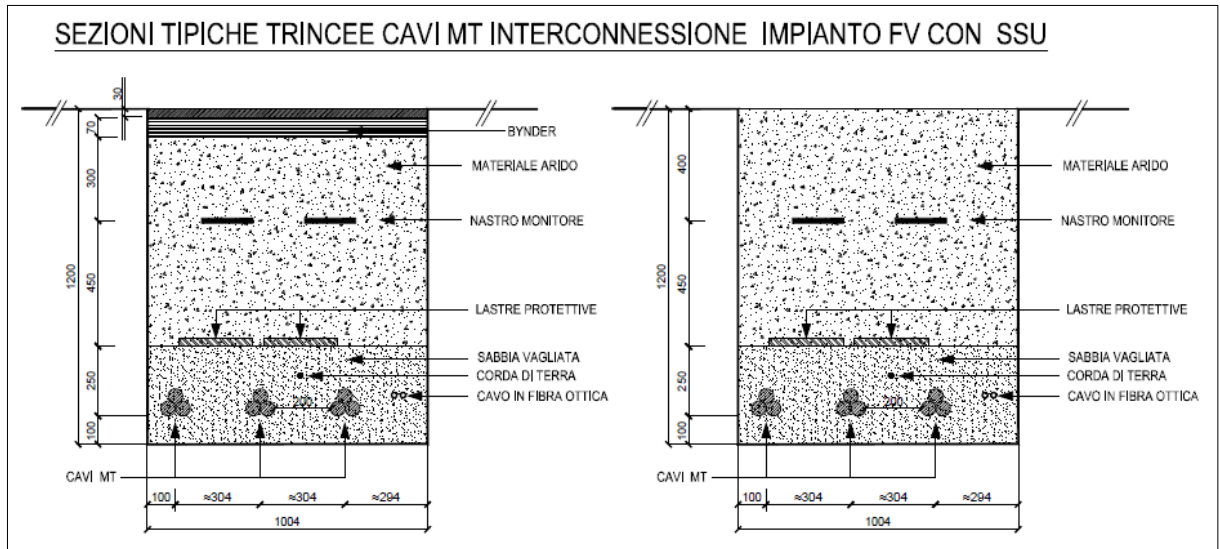
Figura 2: Tipo sezione su strada asfaltata e sterrata
