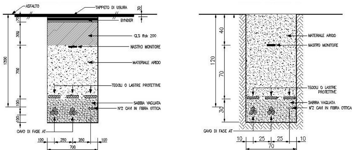
Figura 2: Tipici di posa cavi AT con n°1 e n°2 linee su viabilità asfaltata e terreno vegetale
