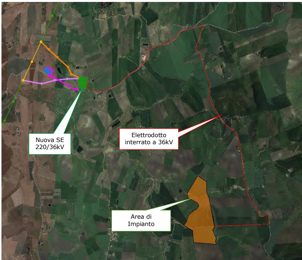
Figura 1: Tracciato degli elettrodotti AT
