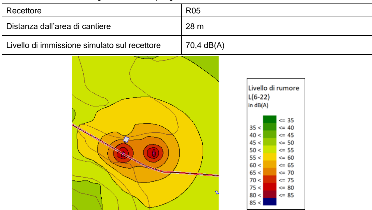
Figura 8.11 – Riepilogo simulazione – Ricettore R05
