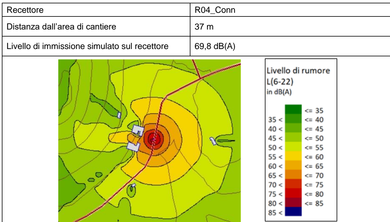
Figura 8.10 – Riepilogo simulazione – Ricettore R04_CONN
