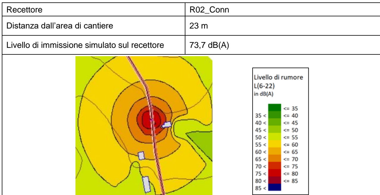
Figura 8.8 – Riepilogo simulazione – Ricettore R02_CONN
