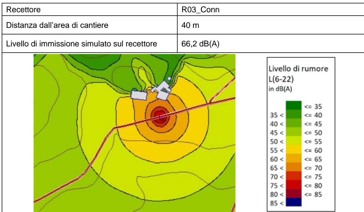
Figura 8.9 – Riepilogo simulazione – Ricettore R03_CONN
