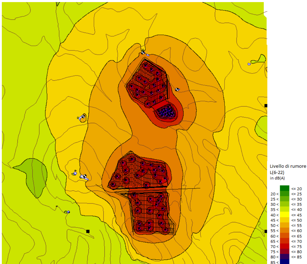
Figura 8.6 – Immagine rappresentante curve di isolivello
