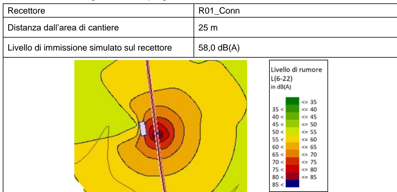
Figura 8.7 – Riepilogo simulazione – Ricettore R01_CONN
