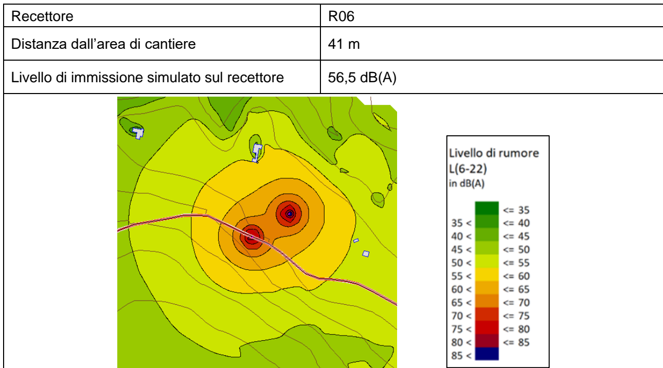
Figura 8.12 – Riepilogo simulazione – Ricettore R06
