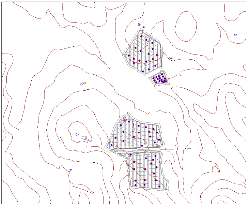
Figura 8.2 – Modello acustico dell'area di studio in SoundPlan
