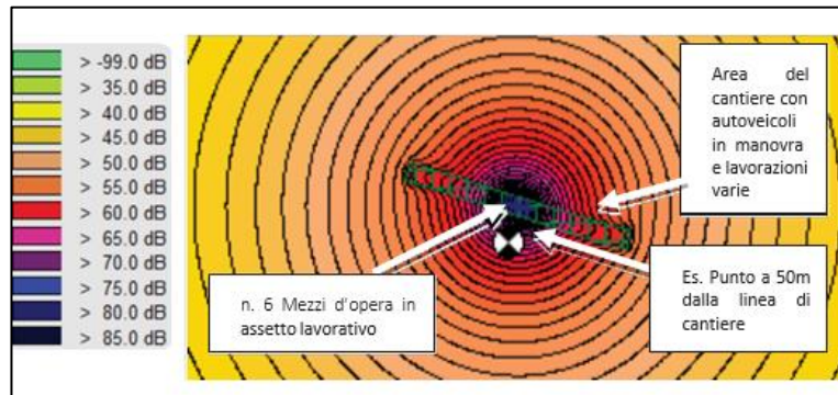
Figura 8.5 – Rappresentazione grafica dell'emissione del cantiere – Curve di ISOLIVELLO dB(A)
