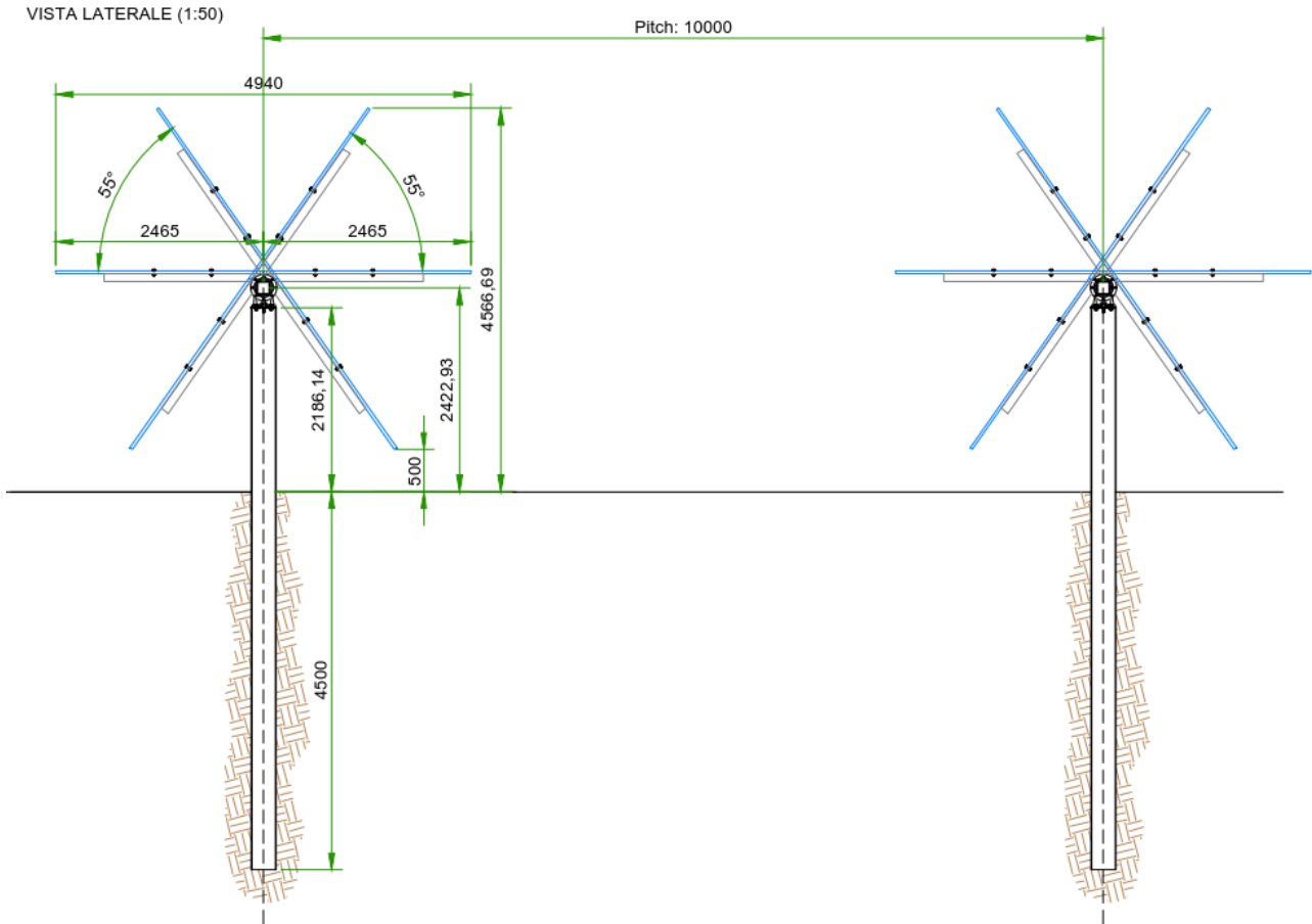
Figura 2.2: struttura di sostegno
