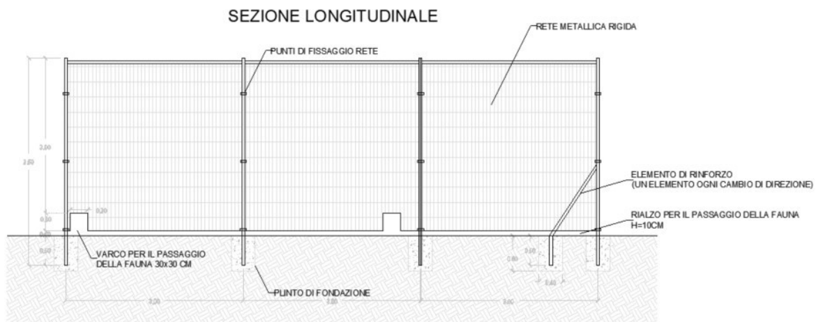
Figura 2.6: Particolare recinzione
