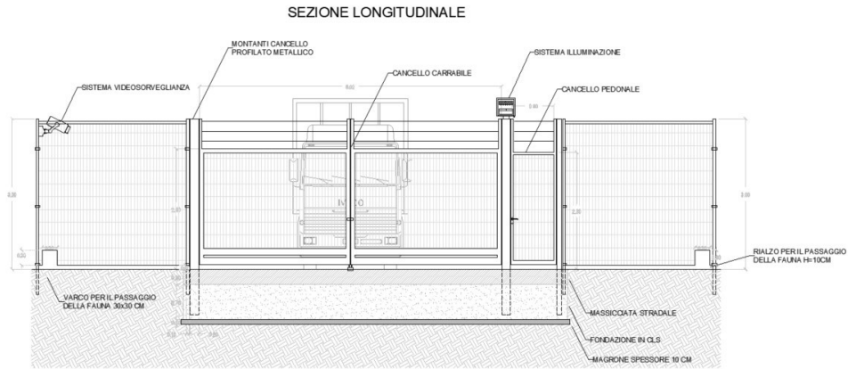
Figura 2.7: Particolare accesso
