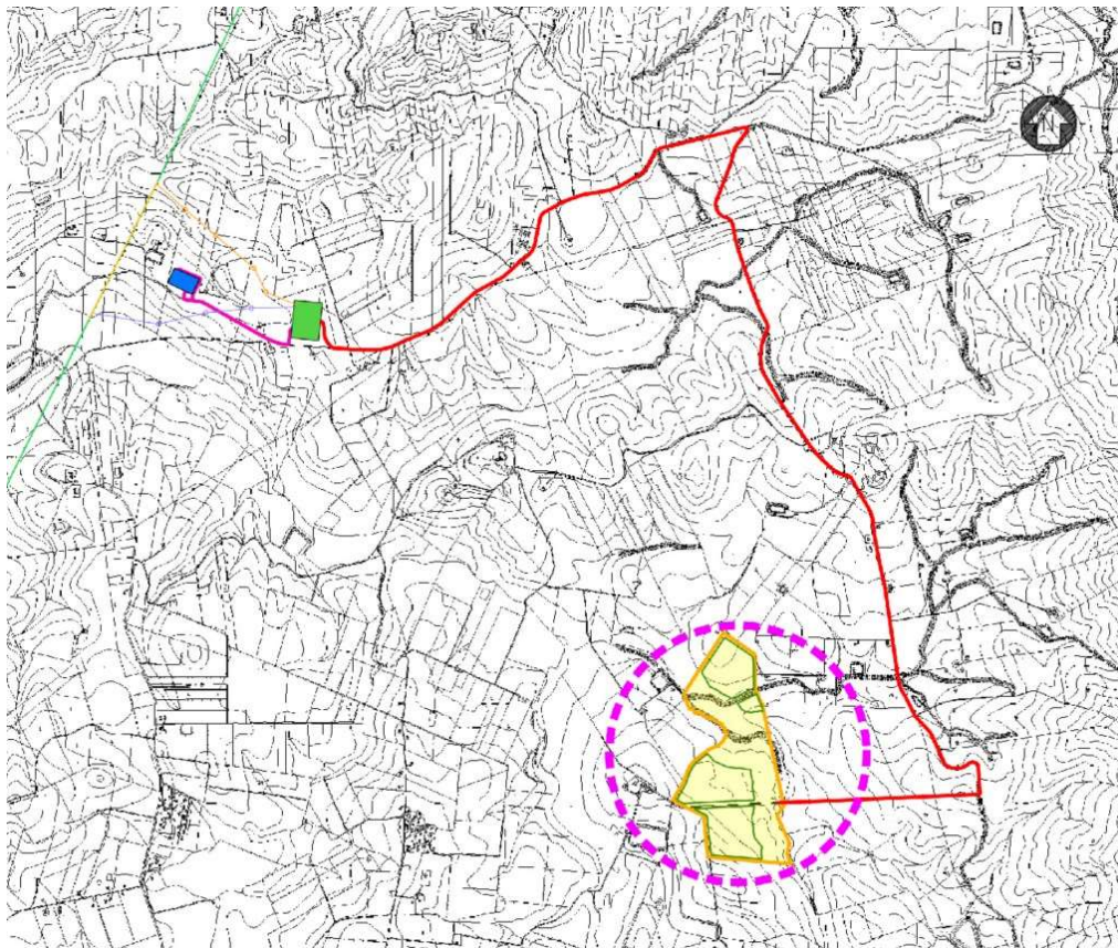
Figura 2.9: Collegamento AT alla Nuova SE 220/36 kV
