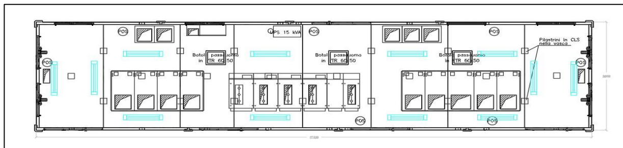
Figura 4.3 – Posizionamento plafoniere Cabina Power Station - cabina BT/MT
