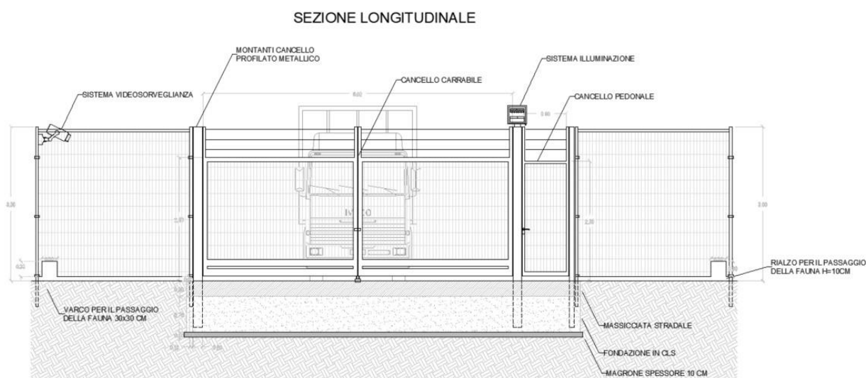
Figura 5.1: Tipico recinzione
