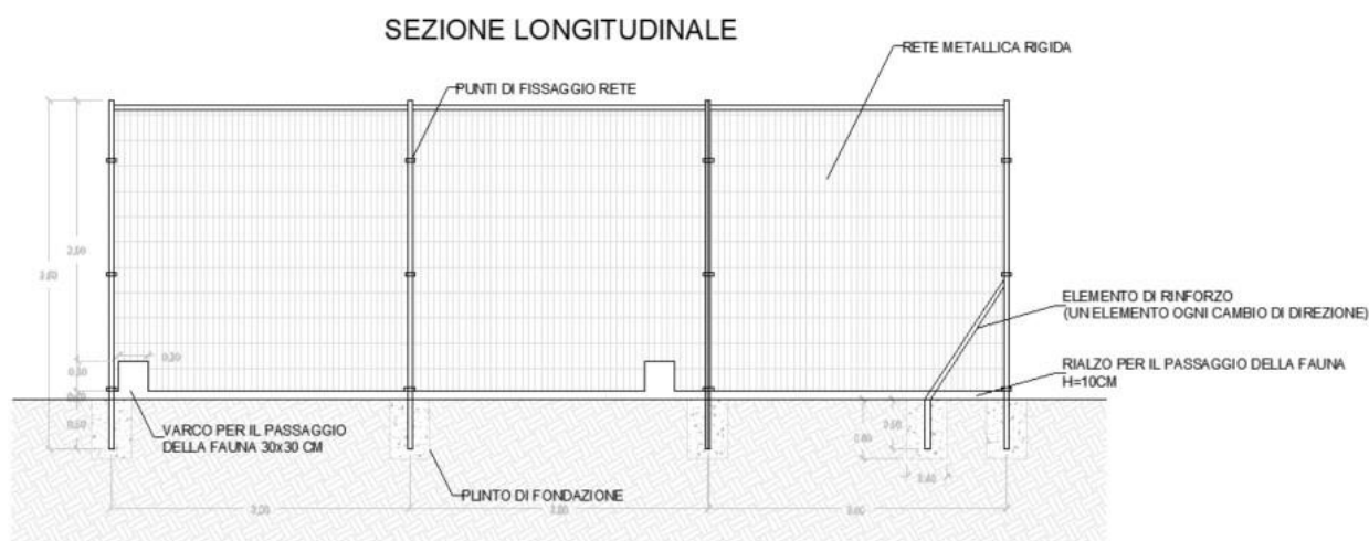
Figura 5.1: Tipico recinzione
