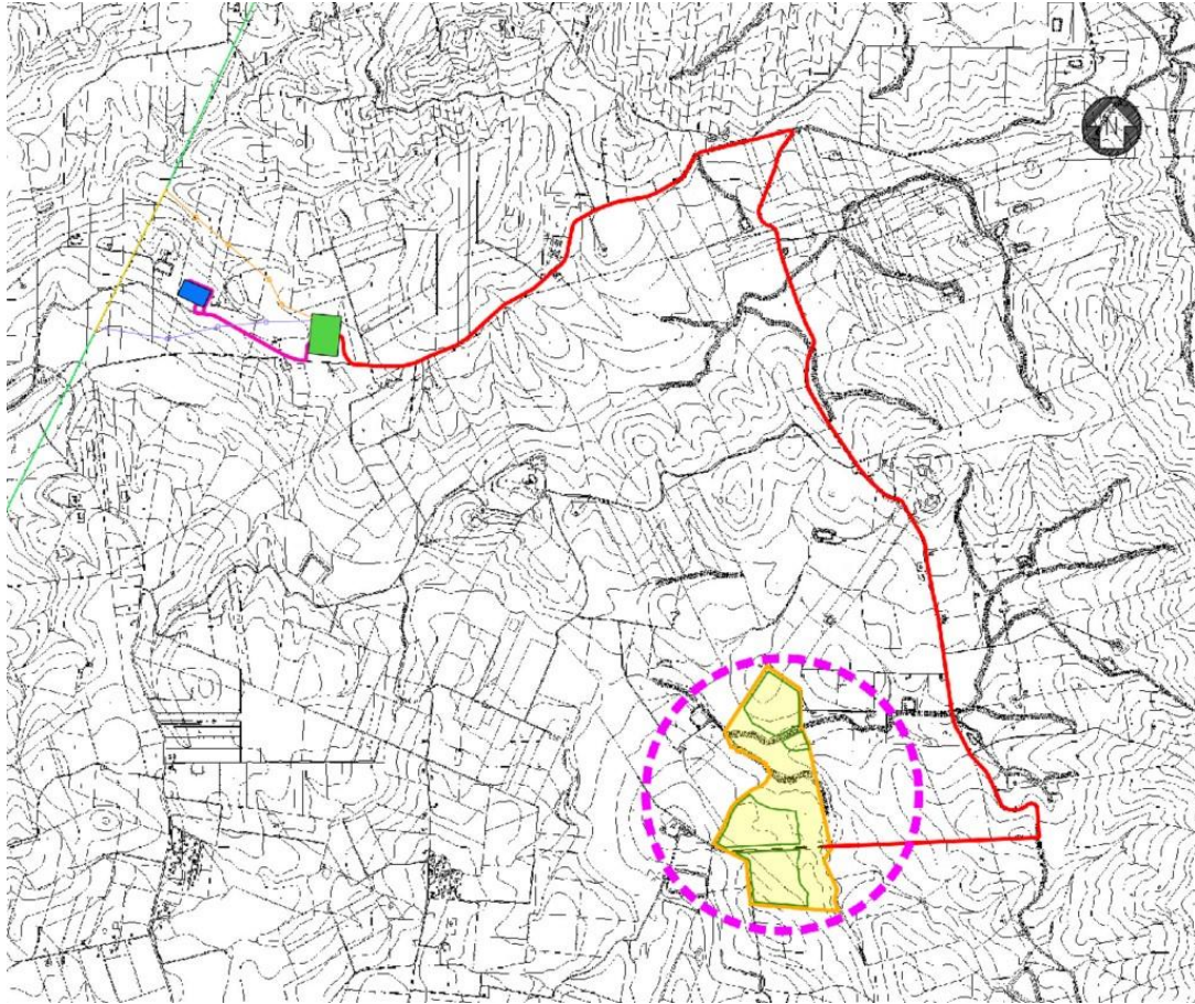
Figura 5.1: Collegamento AT alla Nuova SE 220/36 kV
