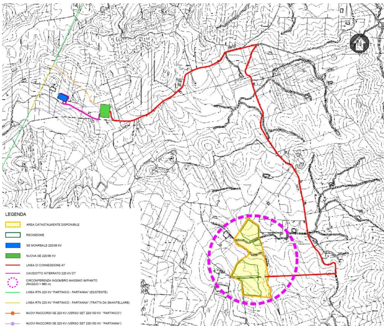
Figura 2.2: Localizzazione dell'area impianto e connessione
