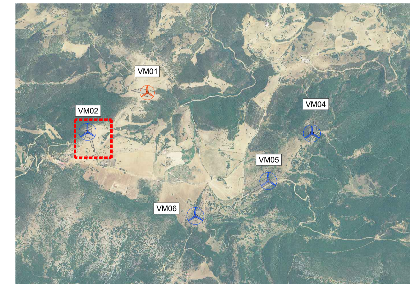
PLANIMETRIA GENERALE – 1:20.000
