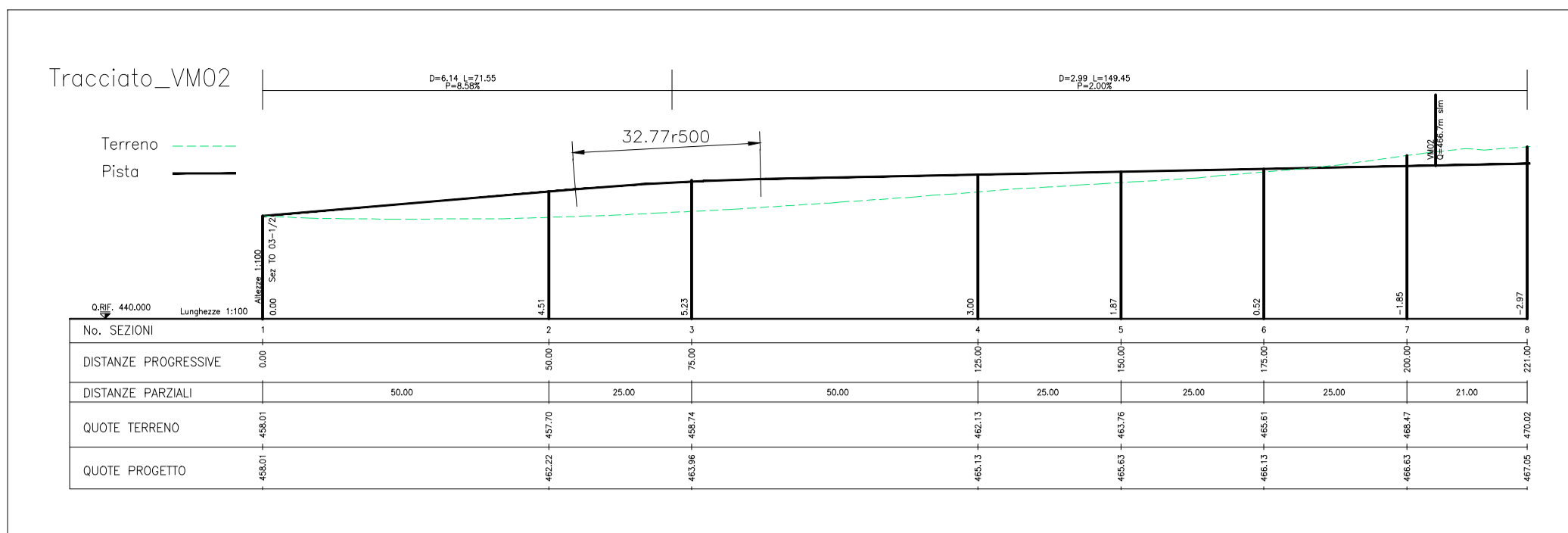
PROFilo LONGITUDINALE VM02 – SCALA 1:1000
