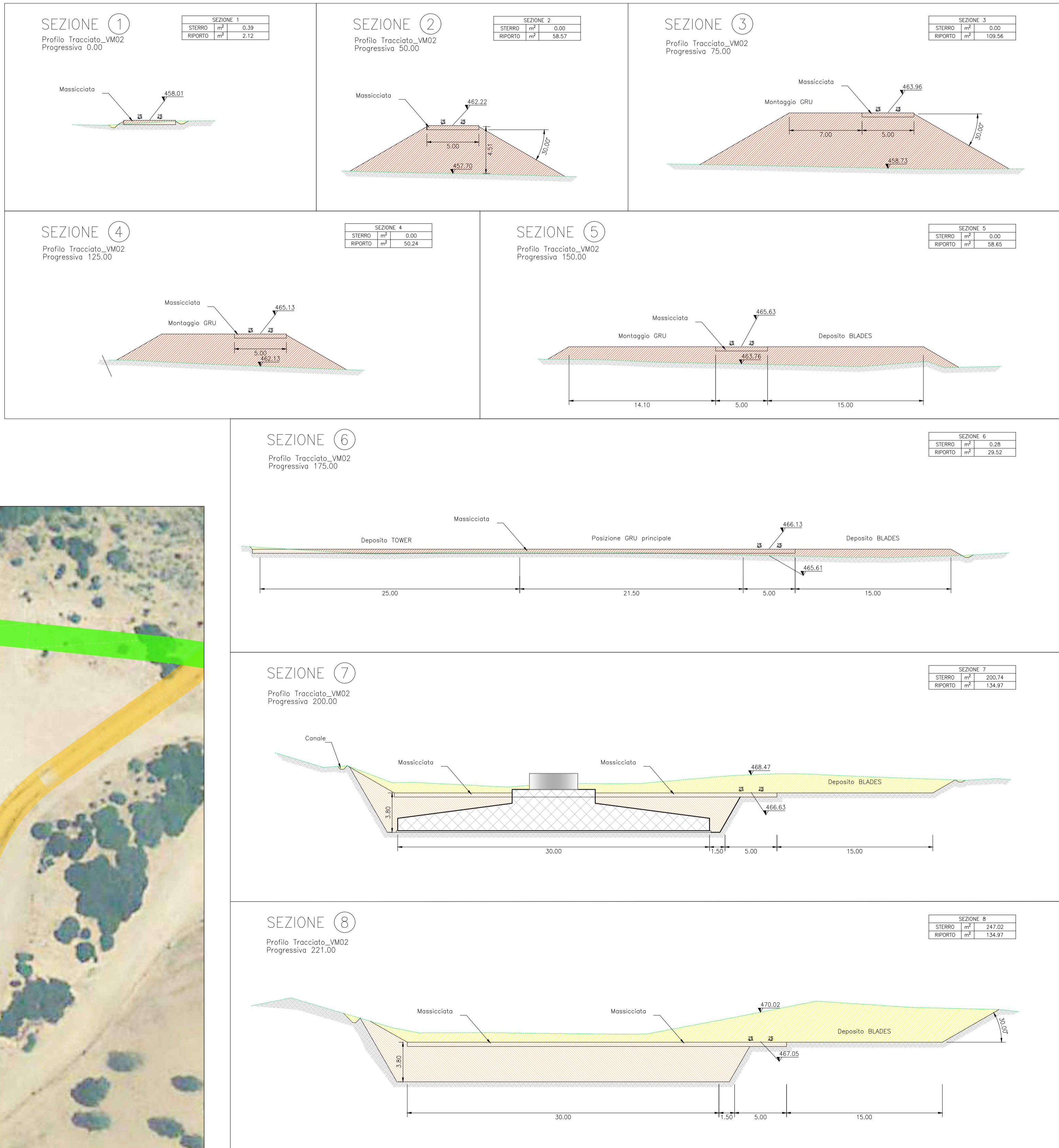
SEZIONI TRASVERSALI VM02 – SCALA 1:250
