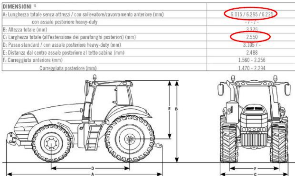
Figura 6: Dimensioni del più grande dei trattori gommati convenzionali prodotti dalla CNH
