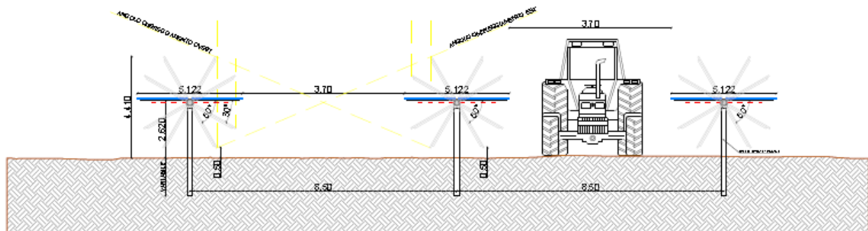
Figura 16: disposizione delle file di lavanda tra le file di moduli fotovoltaici - prospetto
