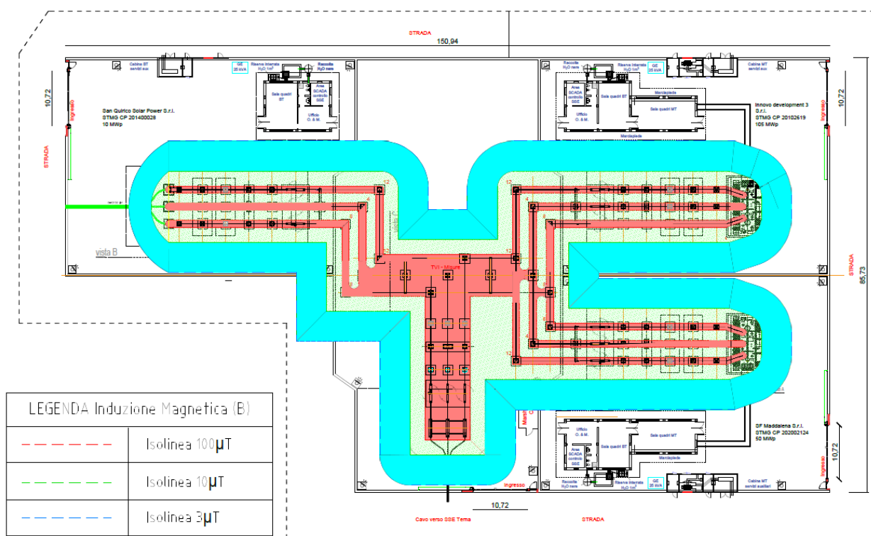
Figura 9 - Sbarre AT in aria - Zone induzione magnetica 3, 10 e 100 µT
