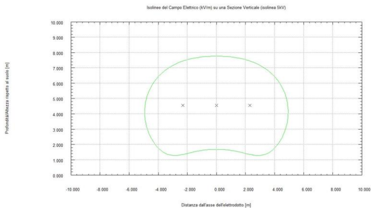
Figura 8 - Sbarre AT in aria - Isolinea campo elettrico 5 kV/m
