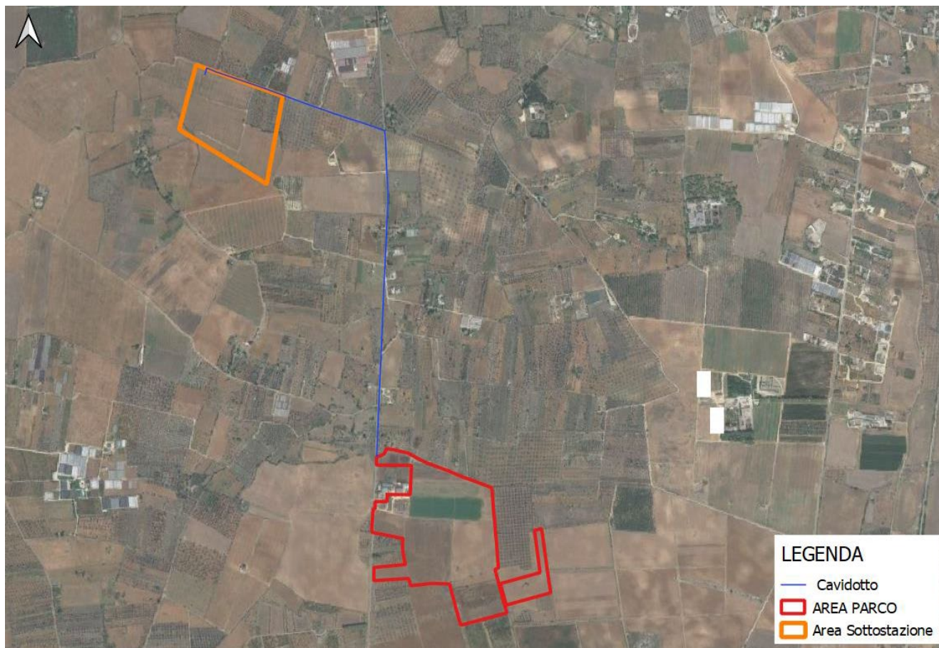
Figura 3 - Inquadramento generale dell'opera su ortofoto
