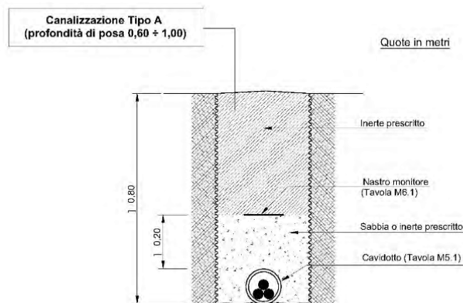
Figura 10 – Sezione di posa cavidotto interno
