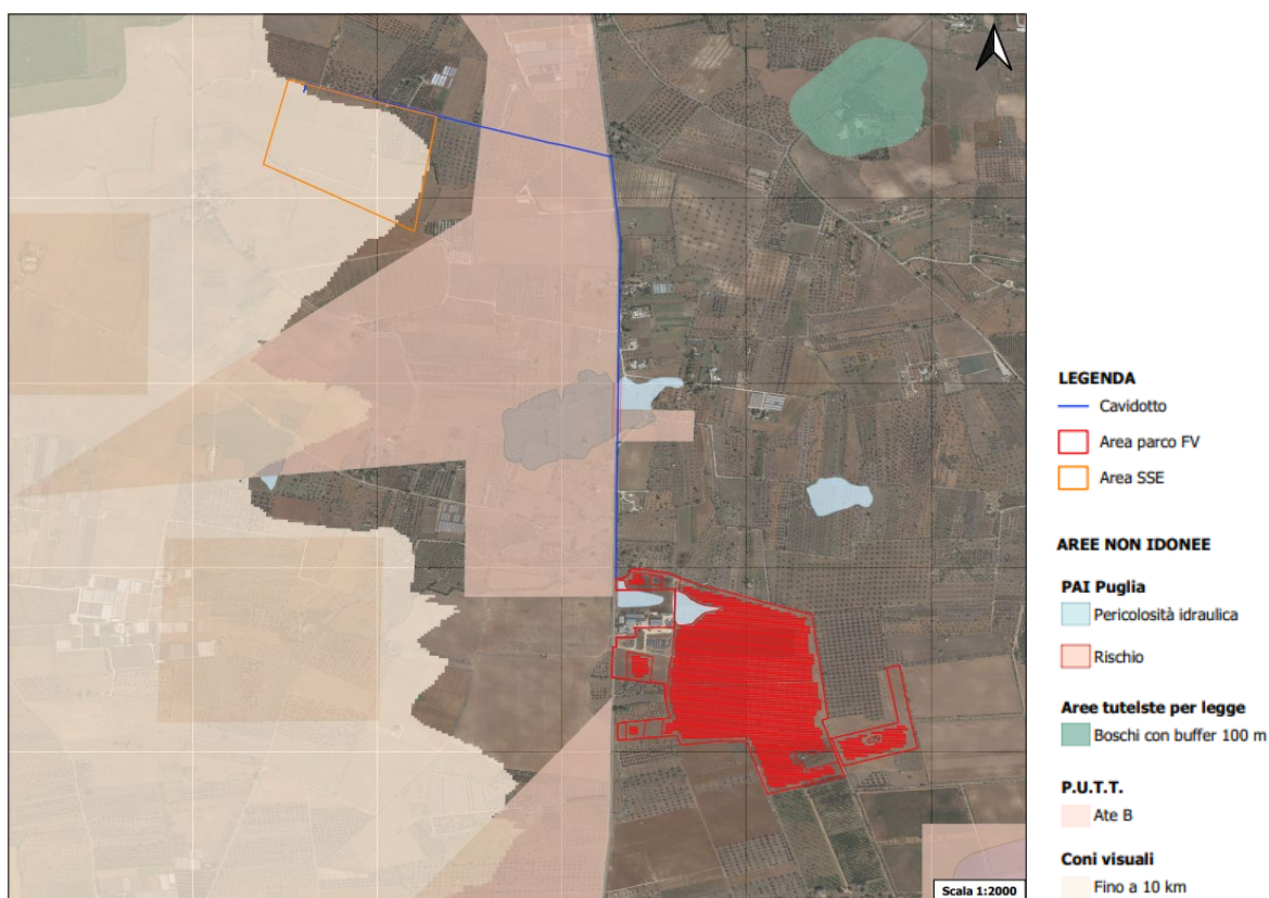
Figura 24 – Carta Aree non Idonee FER
