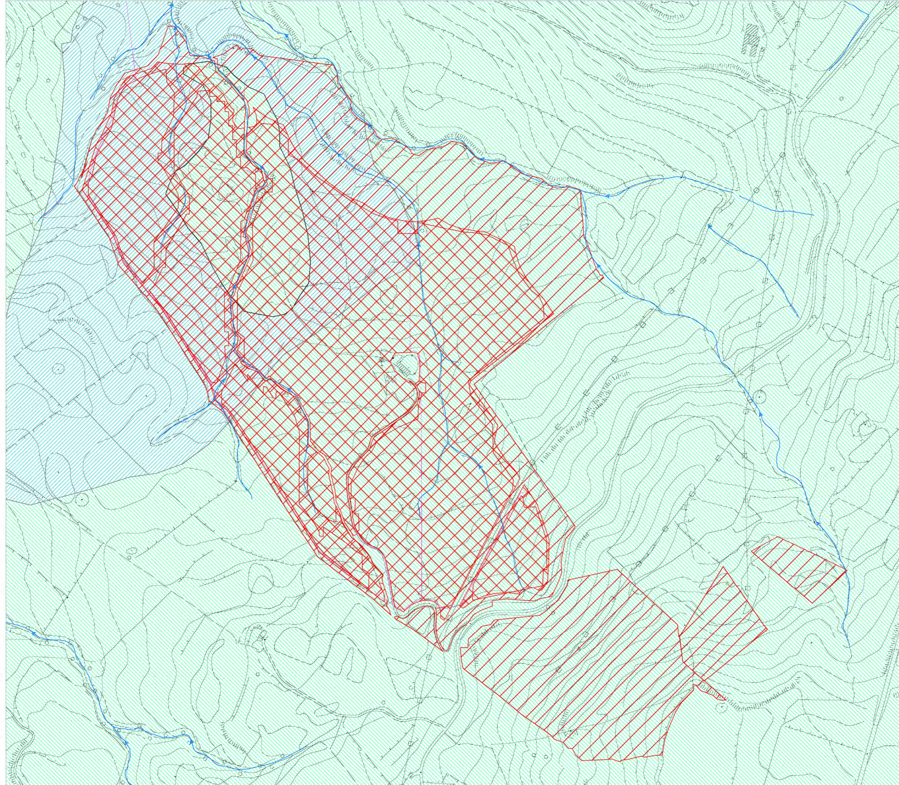
Tav.2: Carta Idrogeologica – Area Parco (1:5000)
