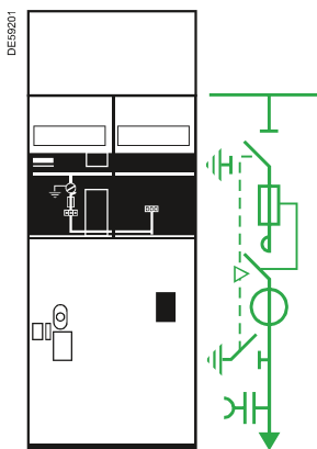
CRM Unità contattore con fusibili 24 kV: 750 mm
