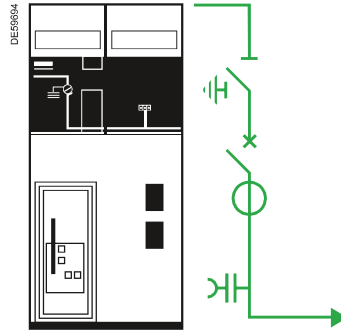
DMVL-D Unità interruttore con sezionatore e uscita sbarre 24 kV: 750 mm
