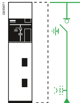
IM Unità arrivo/partenza 24 kV: 375 36 kV: 750 mm
