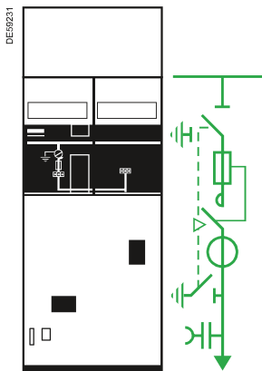
CVM Unità contattore con fusibili 24 kV: 750 mm
