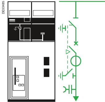
DMVL-A Unità interruttore con sezionatore e partenza cavo 24 kV: 750 mm
