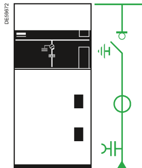
IMC Unità arrivo/partenza 36 kV: 750 mm
