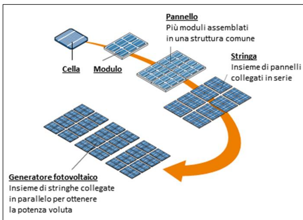
Figura 8: unità elementari del generatore fotovoltaico
