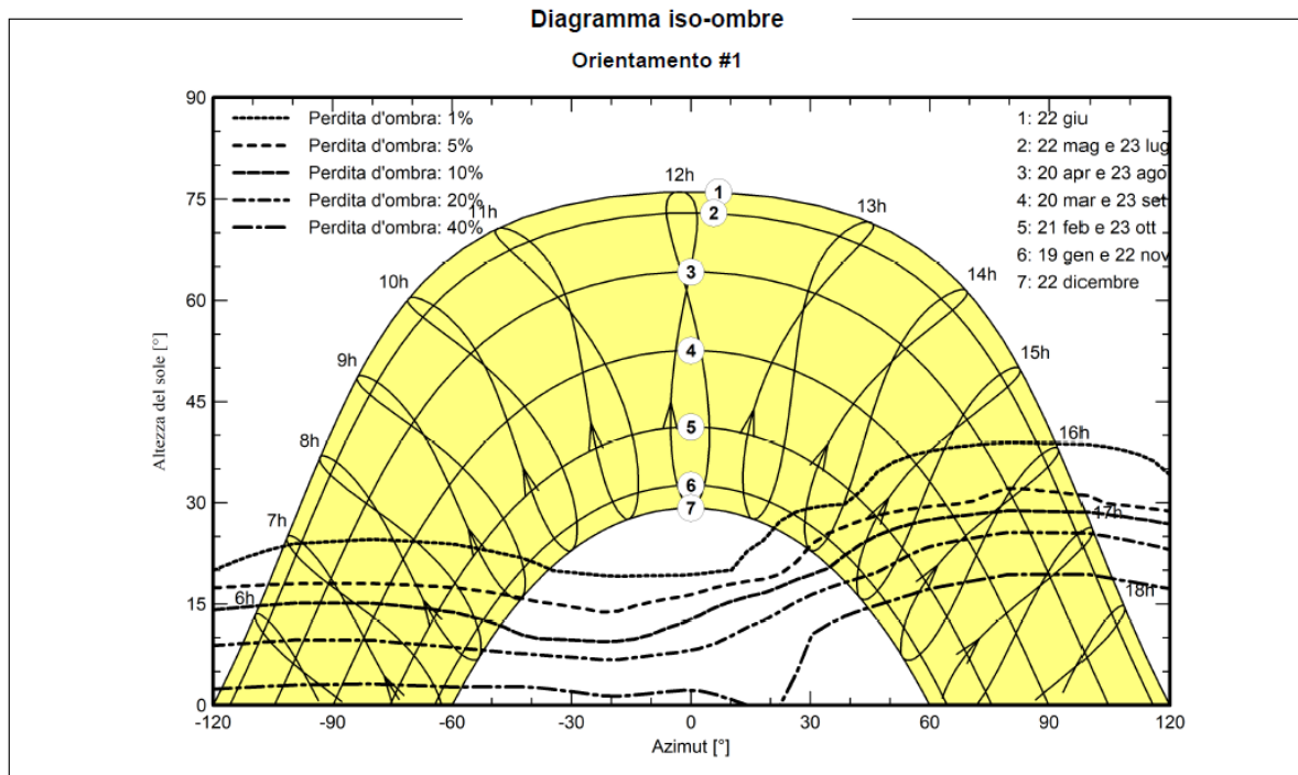
Figura 11: Diagramma iso-ombre
