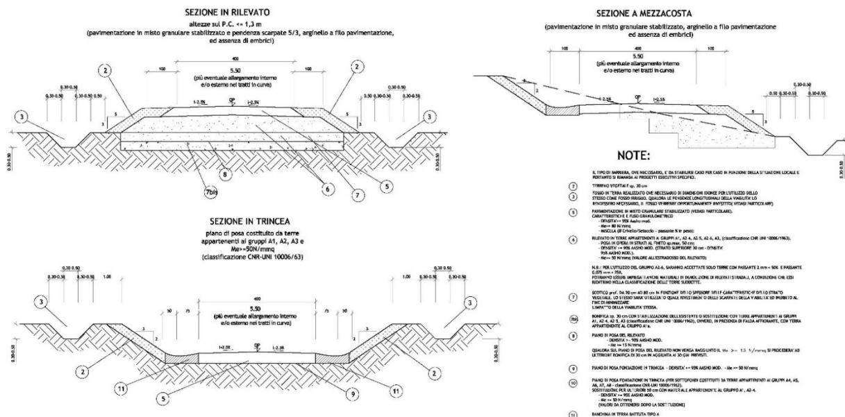
Figura 33: dettagli relativi alle caratteristiche costruttive della viabilità interna al parco
