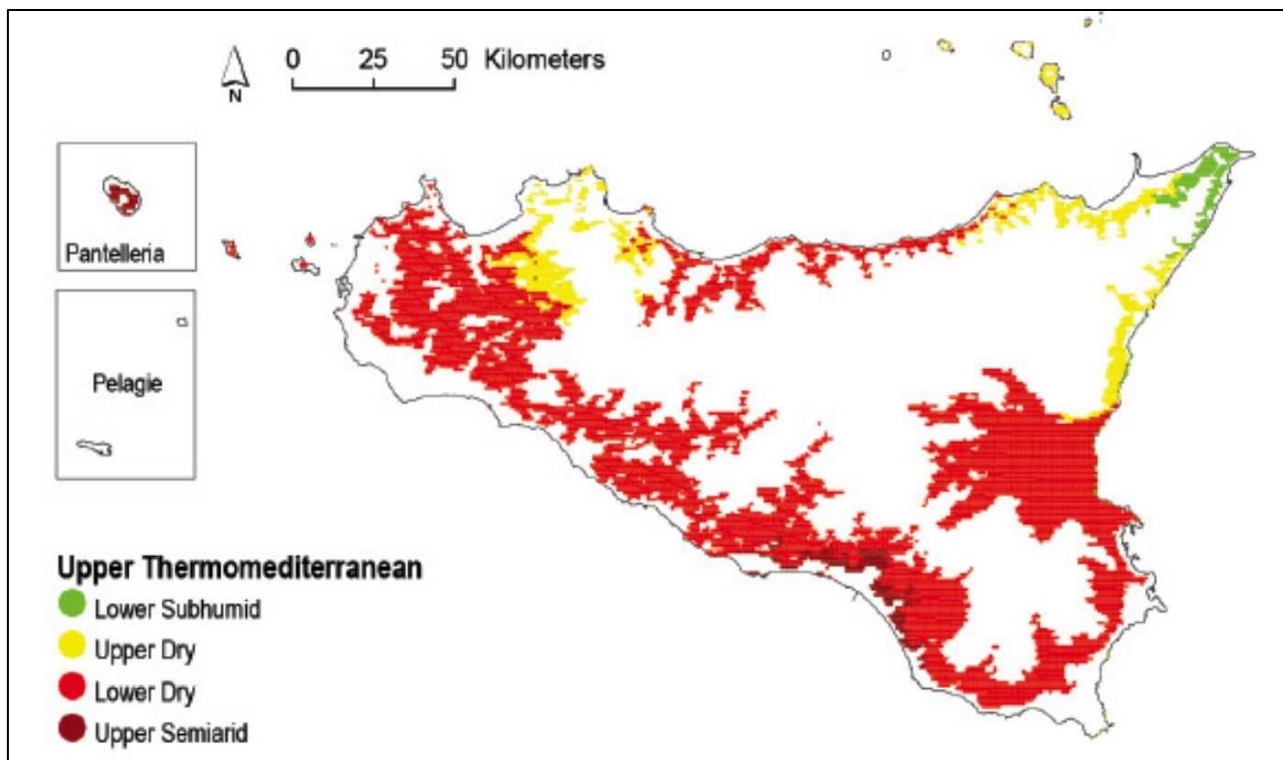
FIGURA 2 – Carta bioclimatica dell'area termomediterranea della Sicilia
