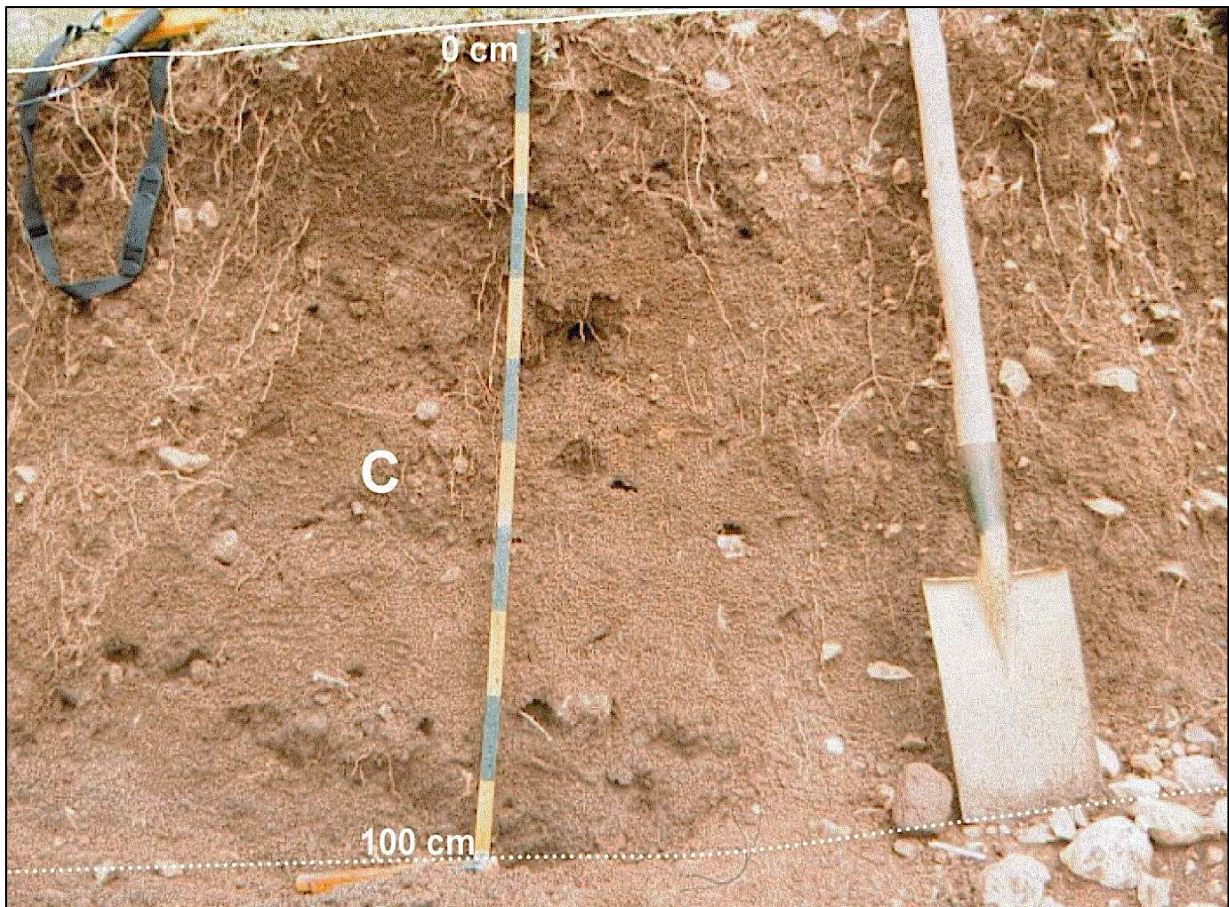
FIGURA 3 – Profilo tipo di regosuolo (WRB regosol)
