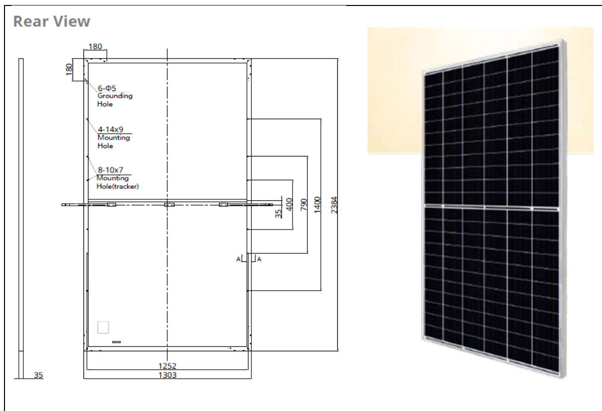
Figura 36: pannello FV fino a 665 Wp con dimensioni 2384 x 1303 x 35 mm
