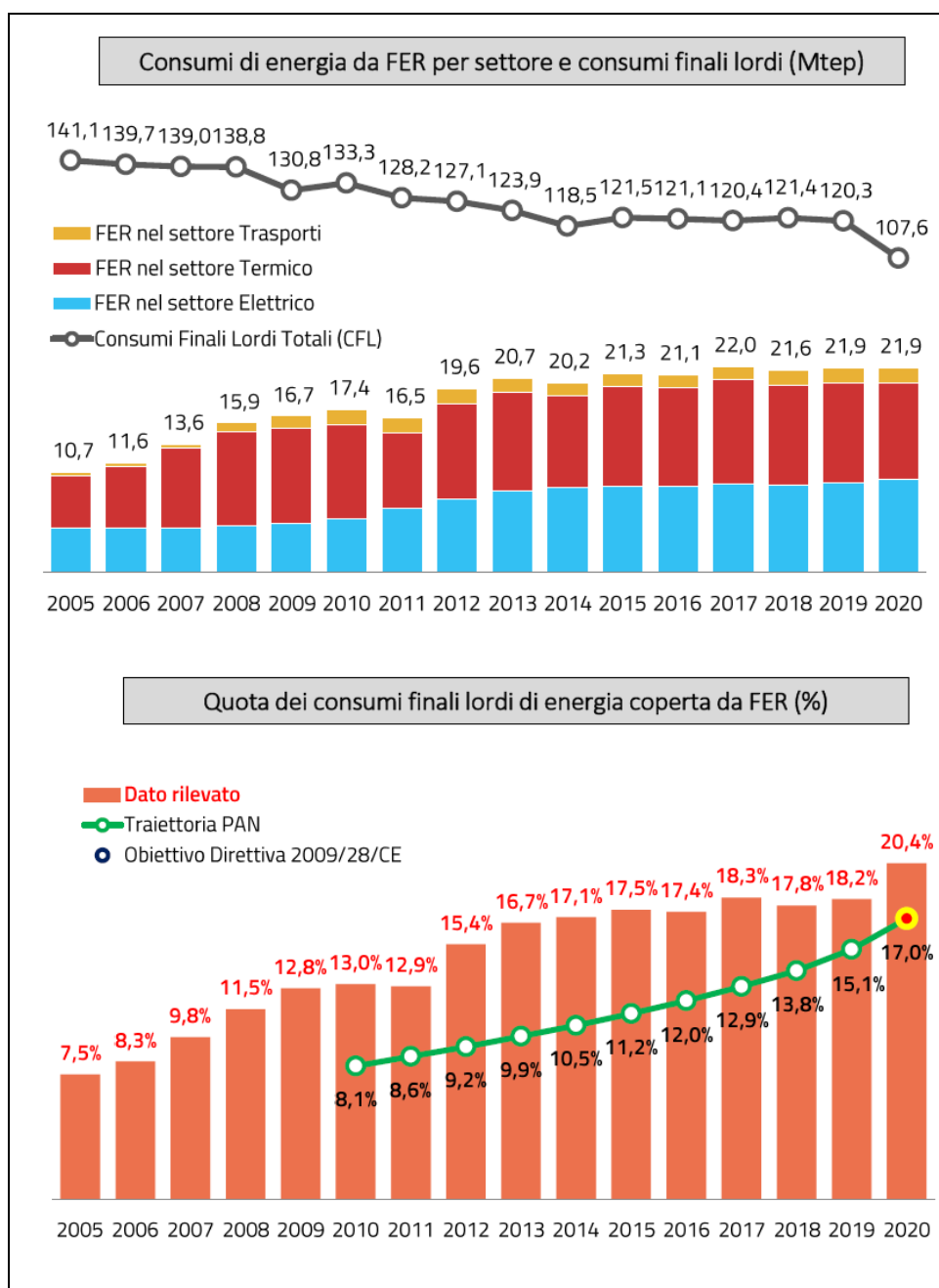
Figura 7: Fonte GSE "Sviluppo e Diffusione delle Fonti Rinnovabili di Energia in Italia e in Europa - anno 2020"
