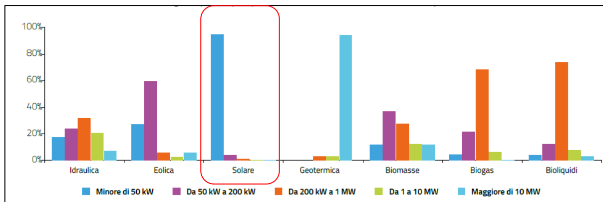
Figura 11: Distribuzione percentuale del numero di impianti per fonte rinnovabile, secondo classe di potenza - FONTE: GSE "Rapporto Statistico FER 2020"
