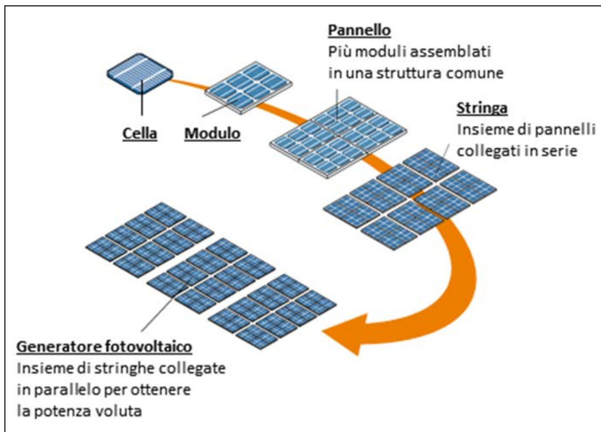
Figura 35: unità elementari del generatore fotovoltaico
