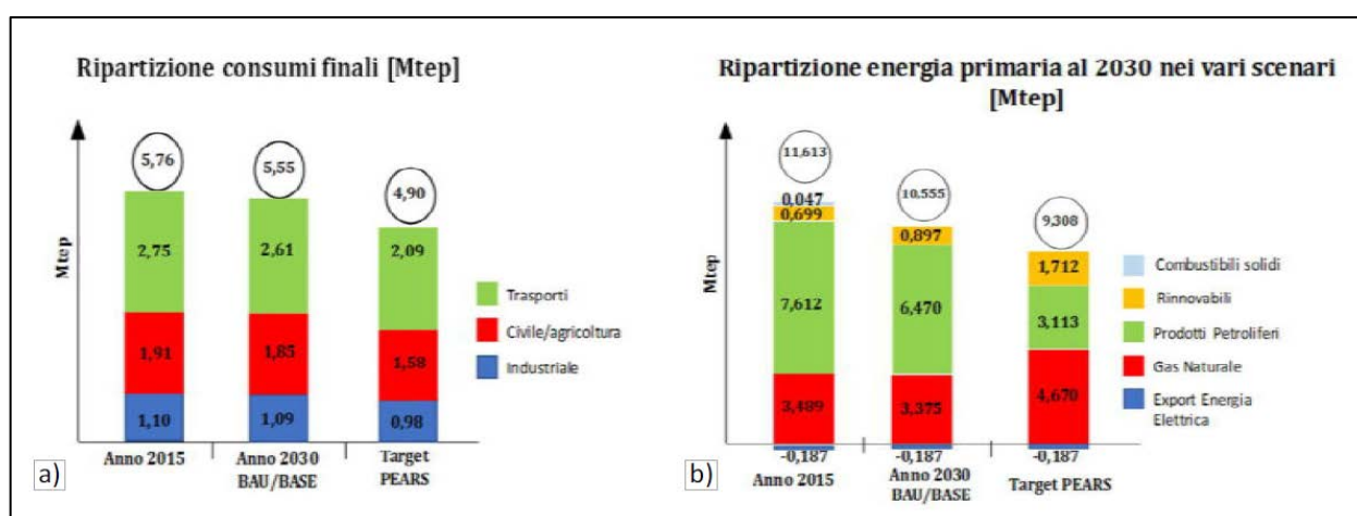
Figura 15: a) Ripartizione dei consumi finali e b) ripartizione energia primaria al 2030 - alternativa PEARS
