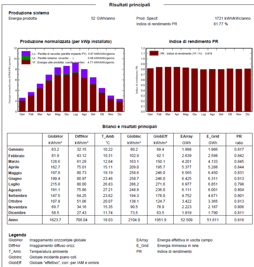
Figura 4: Risultati ottenuti con PVSyst
