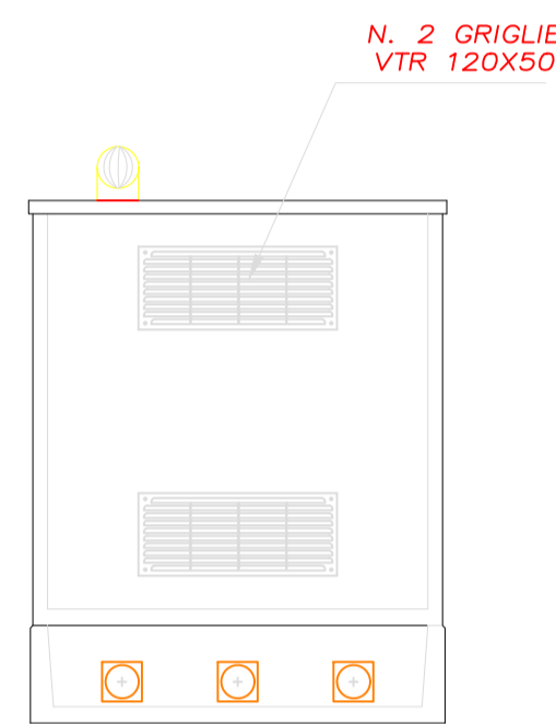
VISTA LATO B
