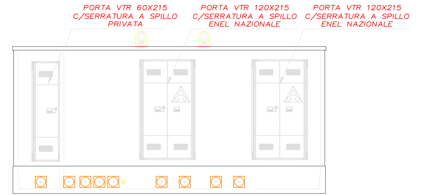
VISTA LATO A
