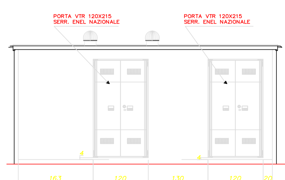
VISTA FRONTALE
