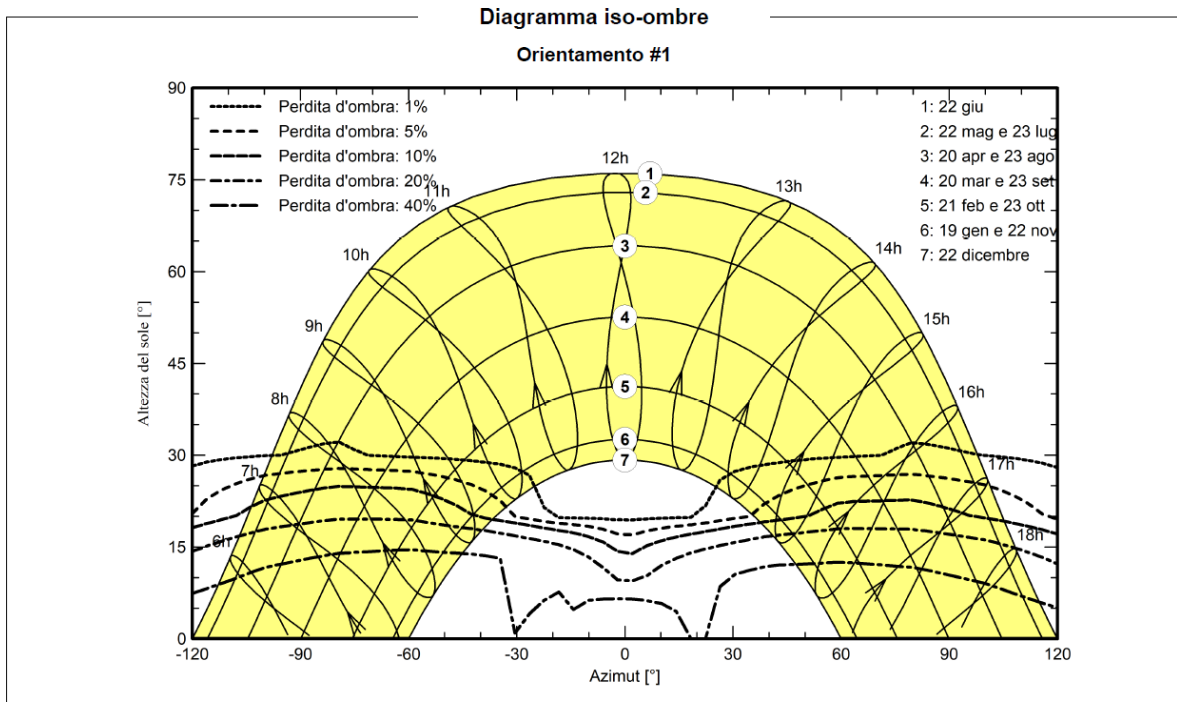
Figura 9: Diagramma iso-ombre
