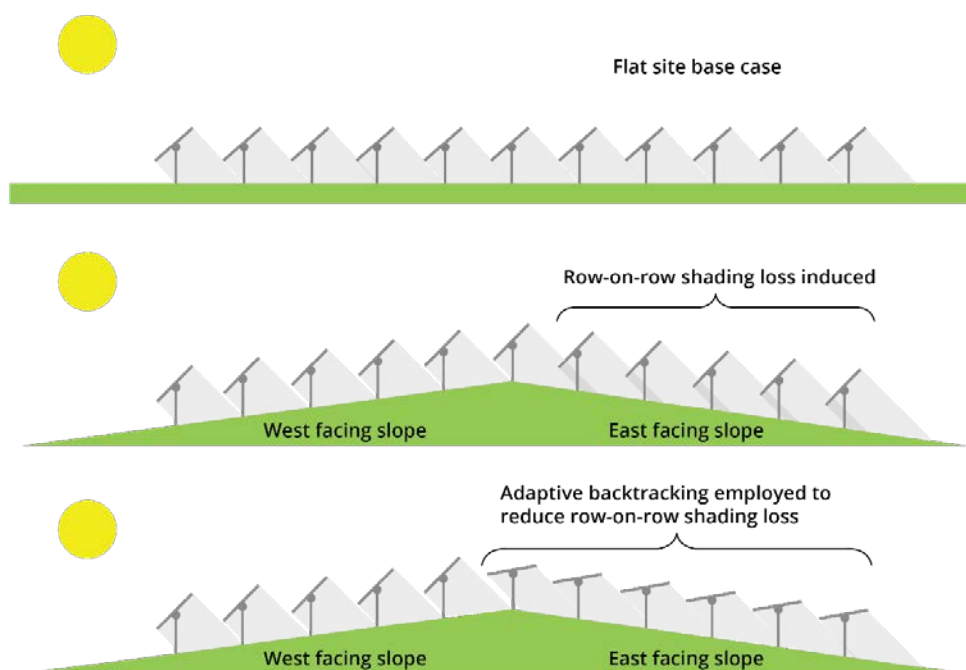
Figura 9: Schema funzionale del Backtracking
