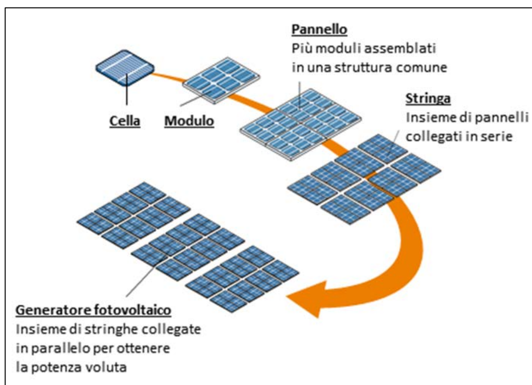
Figura 6: unità elementari del generatore fotovoltaico
