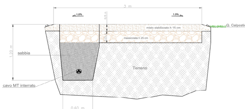
Figura10: Particolare della viabilità interna di servizio dei Campi fotovoltaici.
