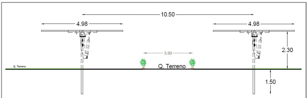
Figura 9: Rappresentazione in sezione di una fascia interfilare, con individuazione della superficie a cielo libero (circa 5 m).
