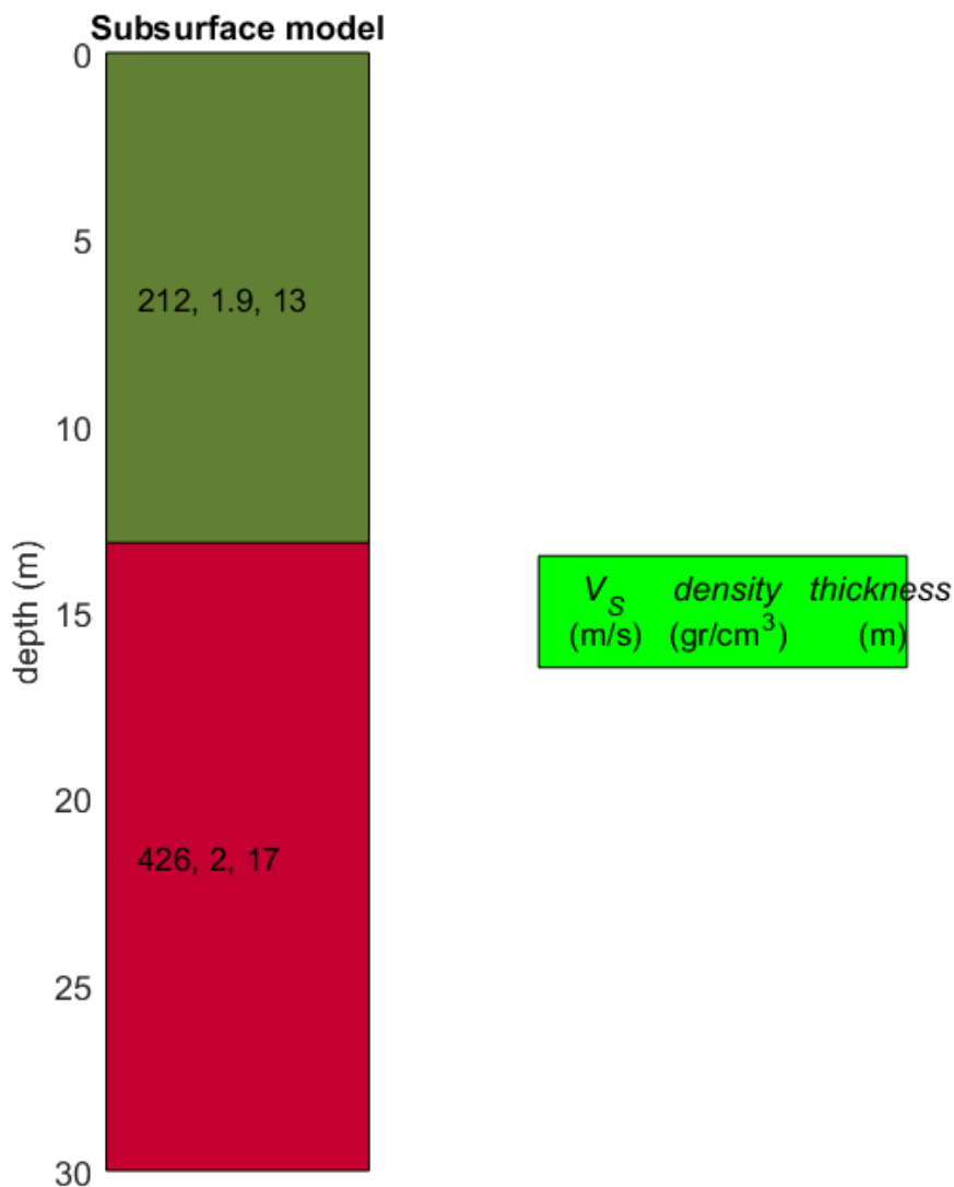
Modello stratigrafico su base sismica
