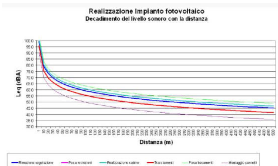
Figura 21.1 Abbattimento del rumore in funzione della distanza
