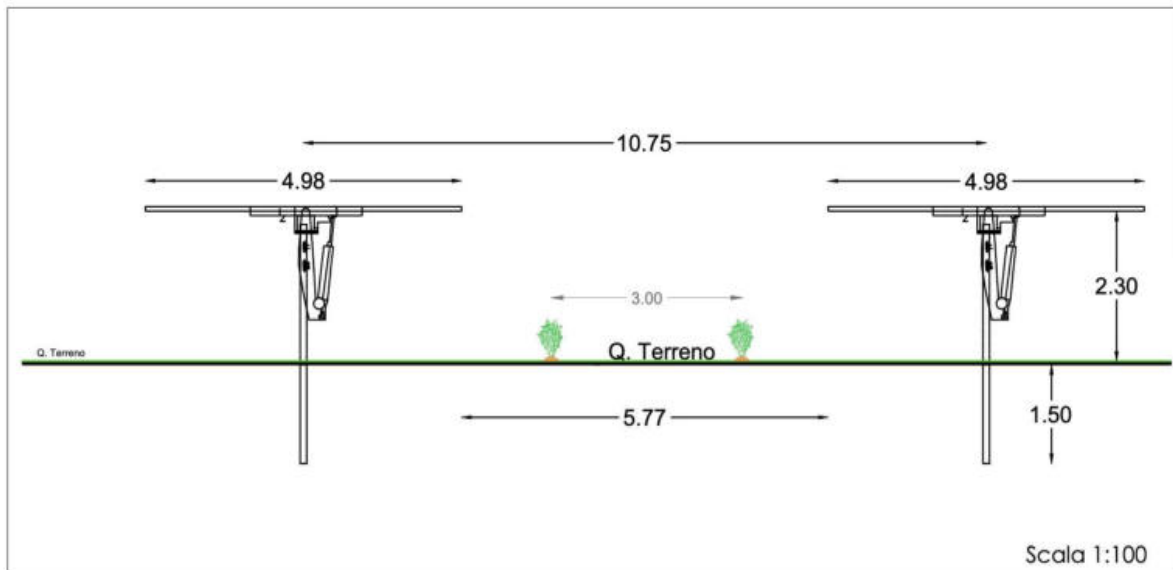
Figura 42-5 Opere di mitigazione Campo 2
