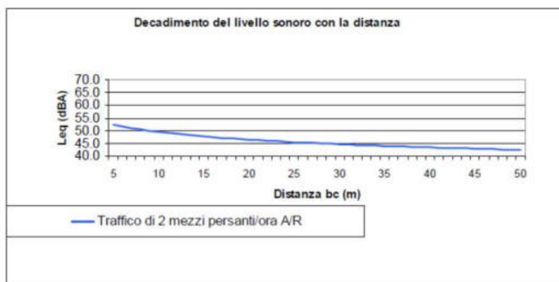
Figura 27-1 decadimento del rumore prodotto dalla circolazione dei mezzi pesanti
