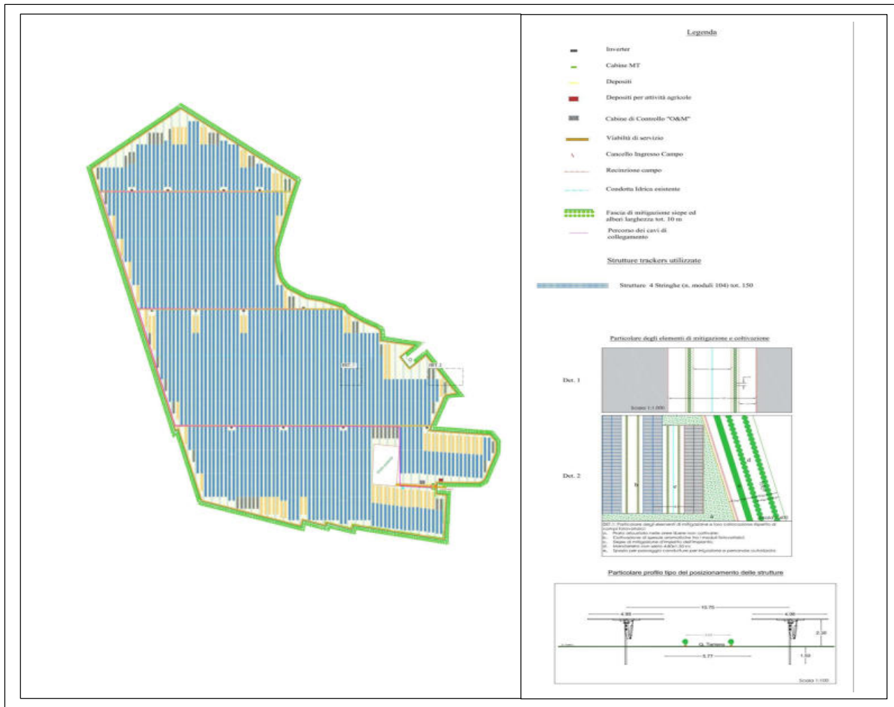
Figura 422-3 Opere di mitigazione Campo 1
