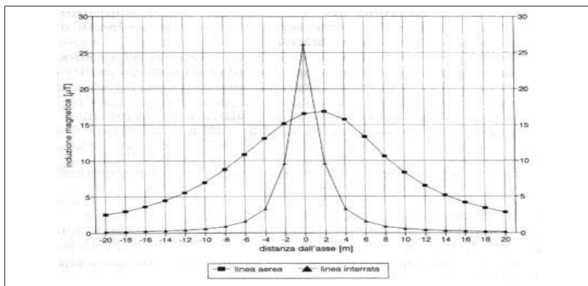
Figura 38-1_Rapporto tra campo di induzione magnetica generato da linea interrata e linea aerea
