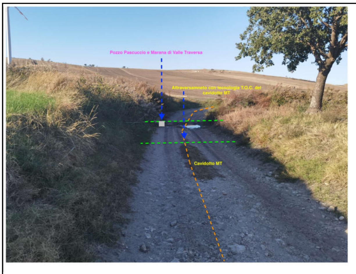
Figura 6-Punto 3 – Attraversamento cavidotto MT proveniente da Campi 1 e 2 con tecnologia T.O.C. del Pozzo Pascuccio-Marana di Valle Traversa
