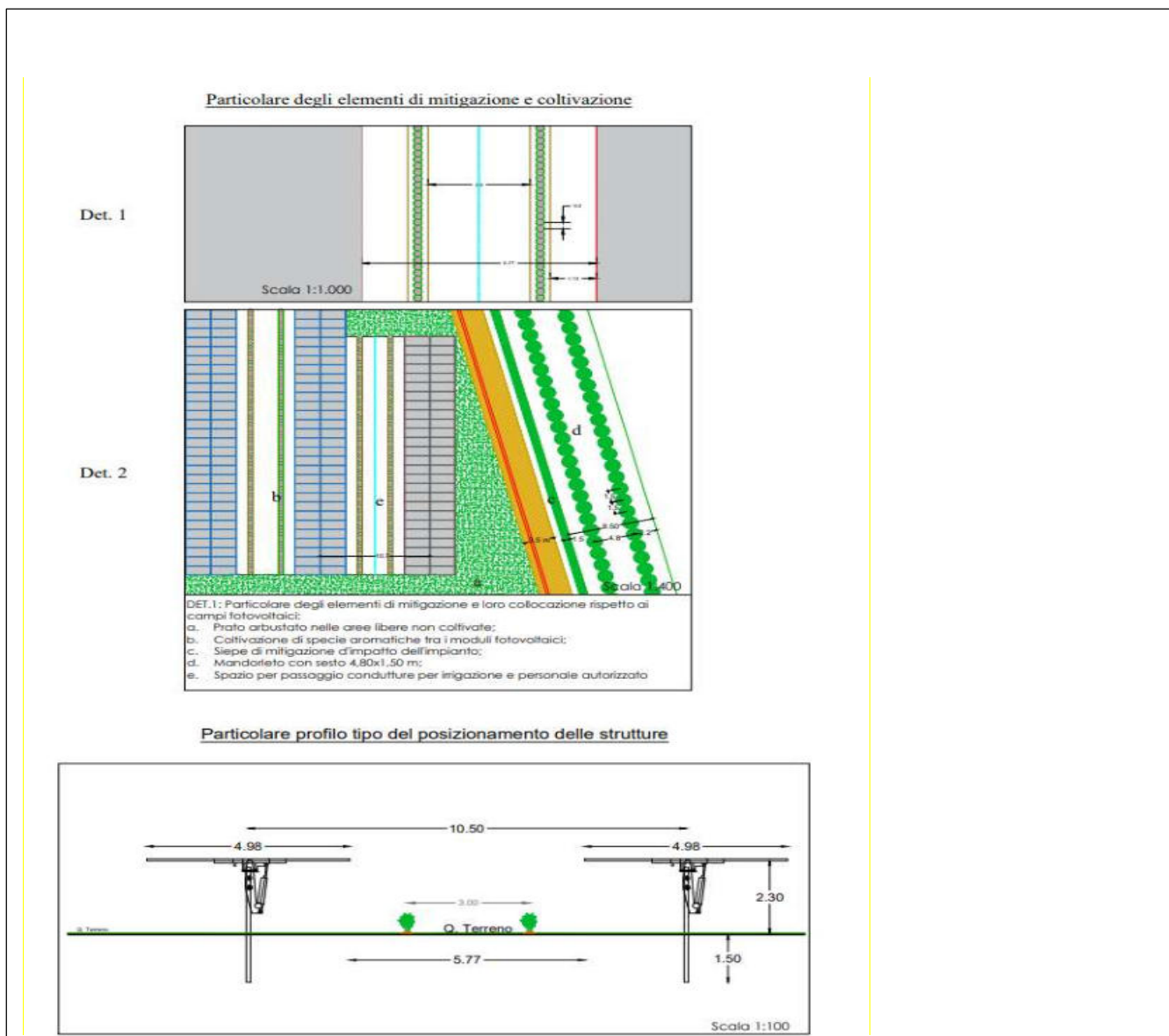
Figura 22-5 Particolare profilo tipo del posizionamento delle strutture
