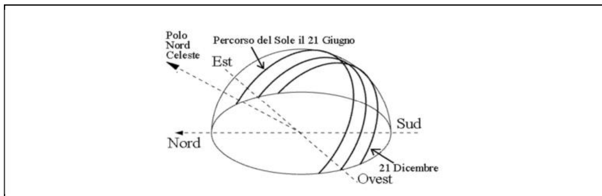
Figura 31-1 Movimento apparente del disco solare per un osservatore situata ad una latitudine nord attorno ai 45°. Per tutte le località situate tra il tropic del Cancro e il Polo Nord Geografico
