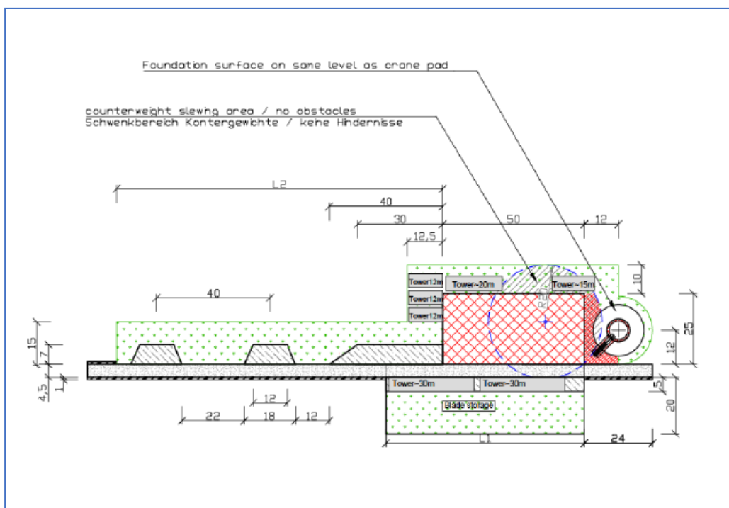
Figura 12 - Piazzola di montaggio
