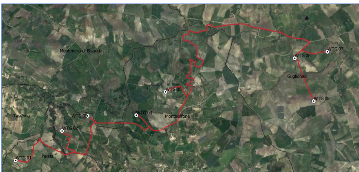
Figura 6 - layout impianto a n.8 aerogeneratori
