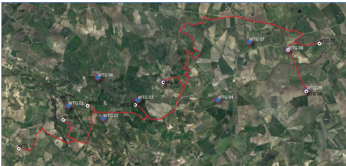
Figura 5 - Sovrapposizione schema layout di partenza a 10 WTG (in blu) e schema definitivo a 8 WTG (in rosso).
