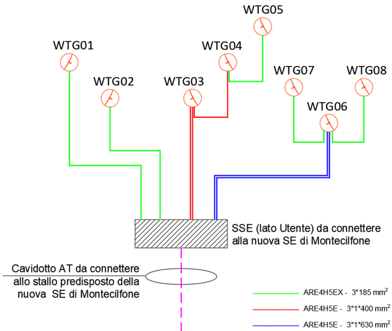
Figura 14 - collegamenti MT, sezione e materiale dei conduttori
