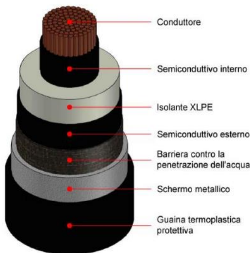
Figura 13 - Esempio di cavo
