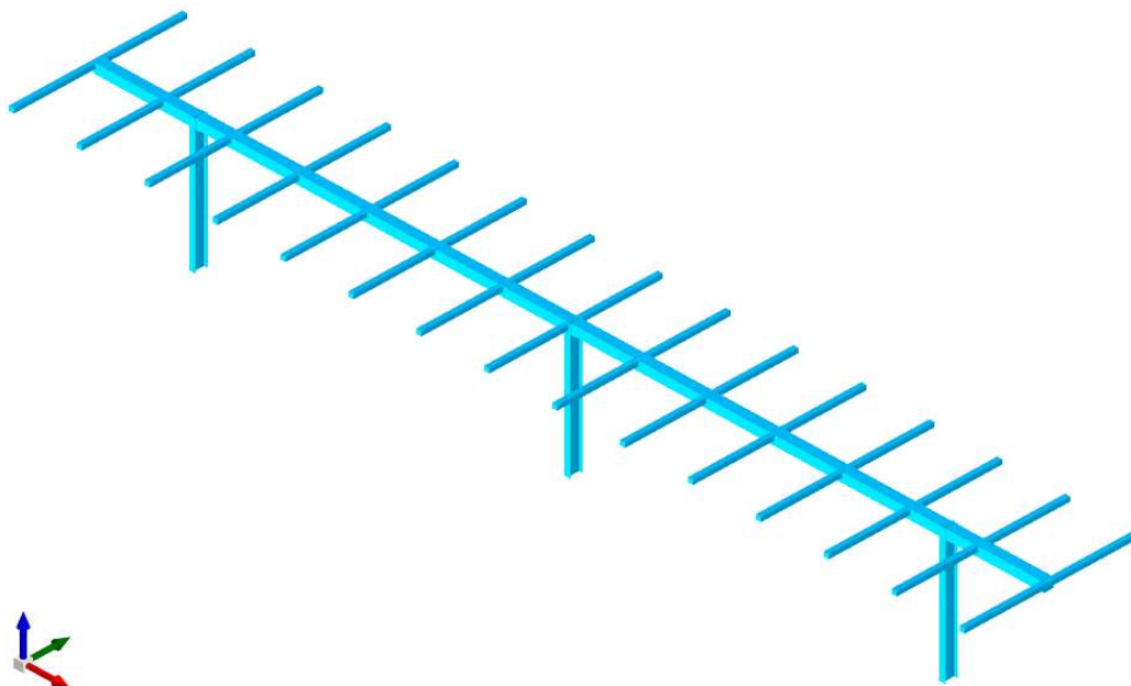
Figura 4.3: Vista assonometrica modello strutturale con posizione della “vela” orizzontale
