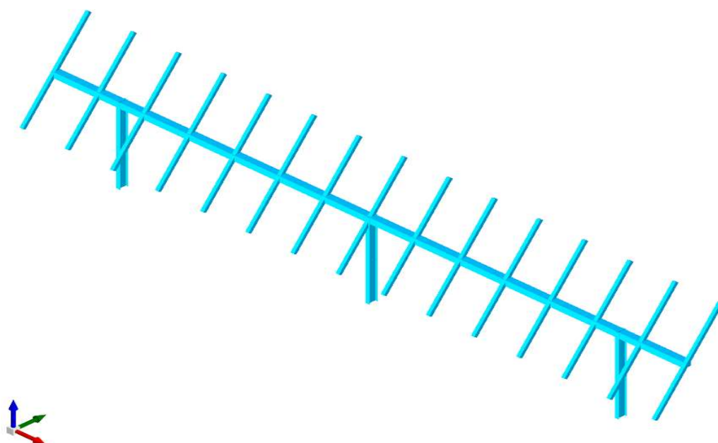
Figura 4.4: Vista assonometrica modello strutturale con posizione della “vela” inclinata di 55°
