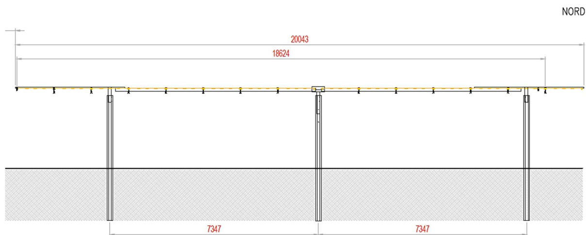
Figura 4.1: Geometria portale di sostegno pannelli fotovoltaici
