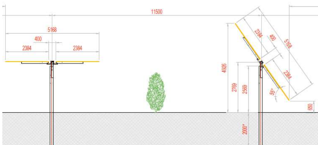
Figura 4.2: Sezione trasversale portale
