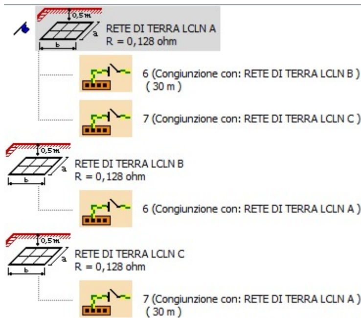
Figura 5.1.4: Calcolo resistenza di terra globale
