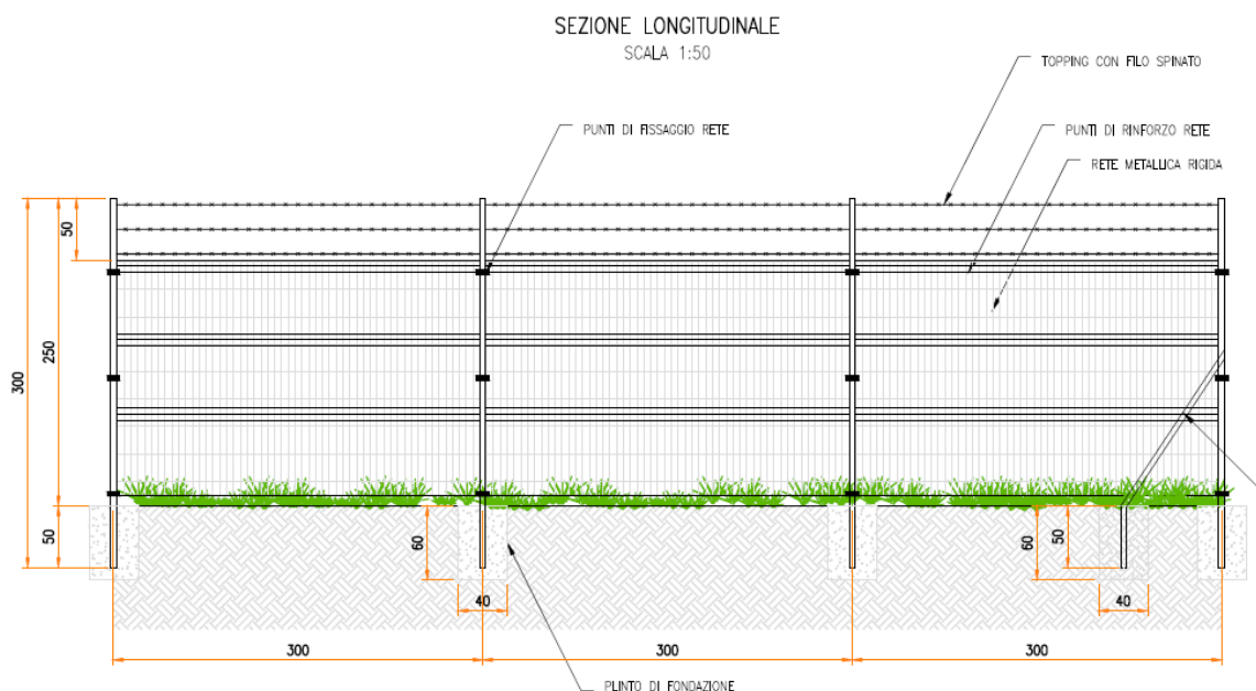
Figura 5.1: Tipico recinzione
