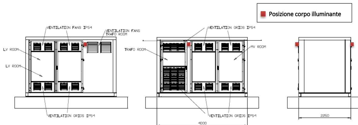
Figura 3.1: Tipologico Cabina di campo (PS) con indicazione della posizione dei corpi illuminanti
