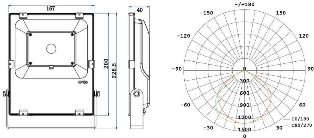
Figura 3.6: Diagramma Fonometrico e Viste Proiettore
