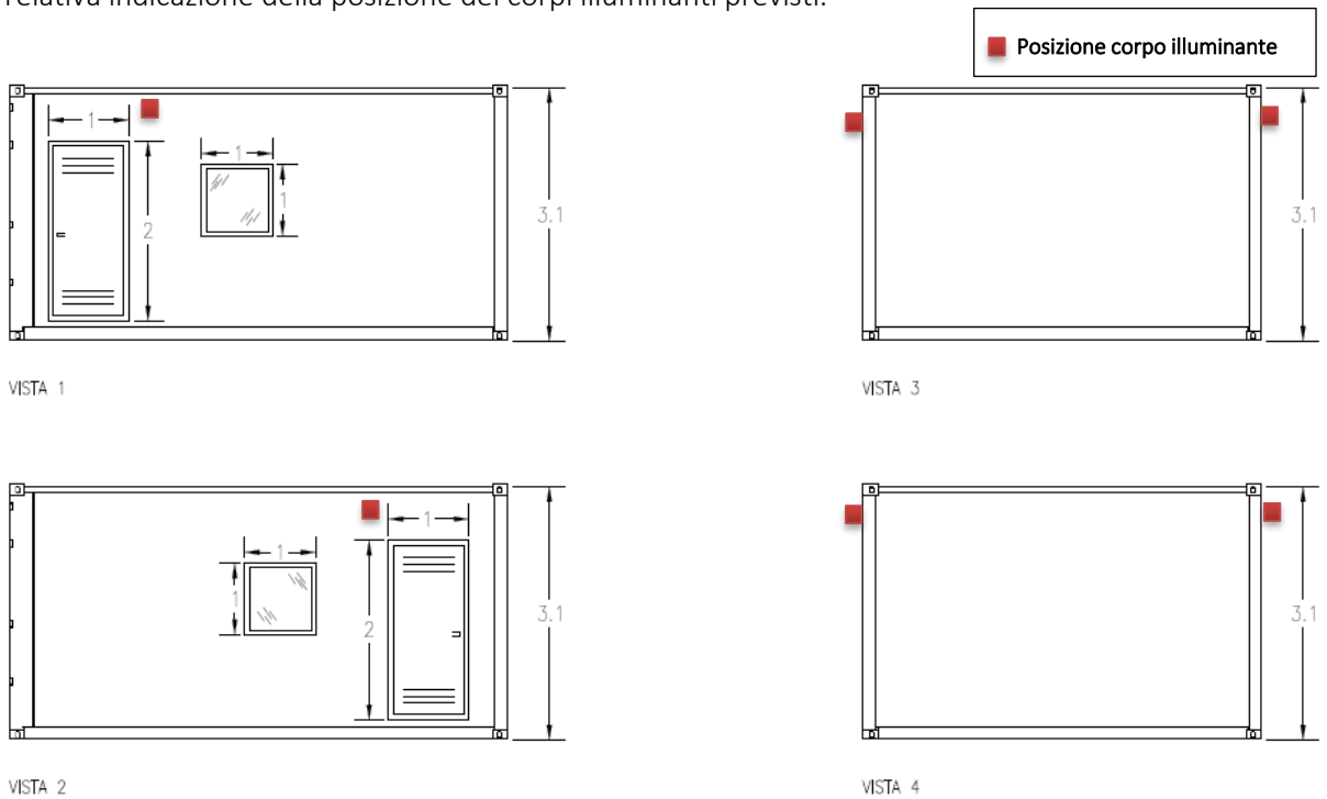
Figura 3.4: Tipologico Cabinato Ufficio
