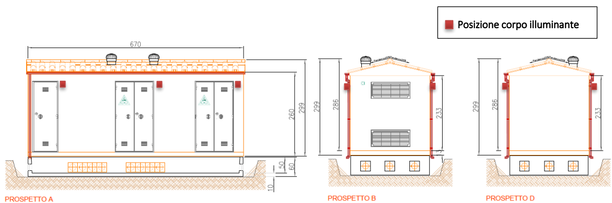
Figura 3.3: Tipologico Cabina di Consegna con indicazione della posizione dei corpi illuminanti
