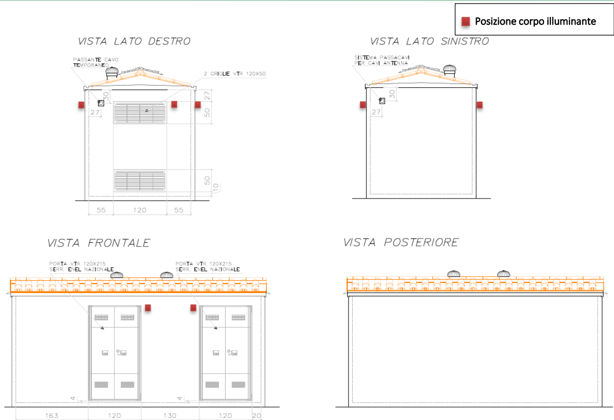
Figura 3.2: Tipologico Cabina di Utente con indicazione della posizione dei corpi illuminanti
