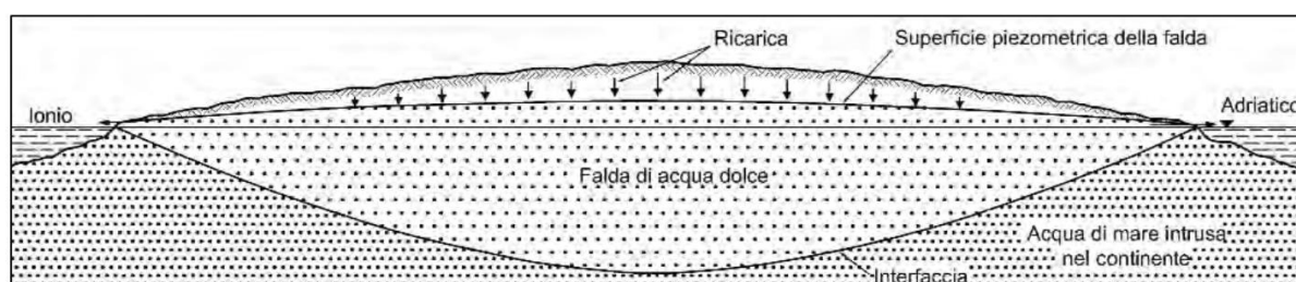
Figura 4.1: Sezione idrogeologica schematica della Penisola Salentina: si noti come la falda profonda galleggi sull'acqua marina d'ingressione continentale
