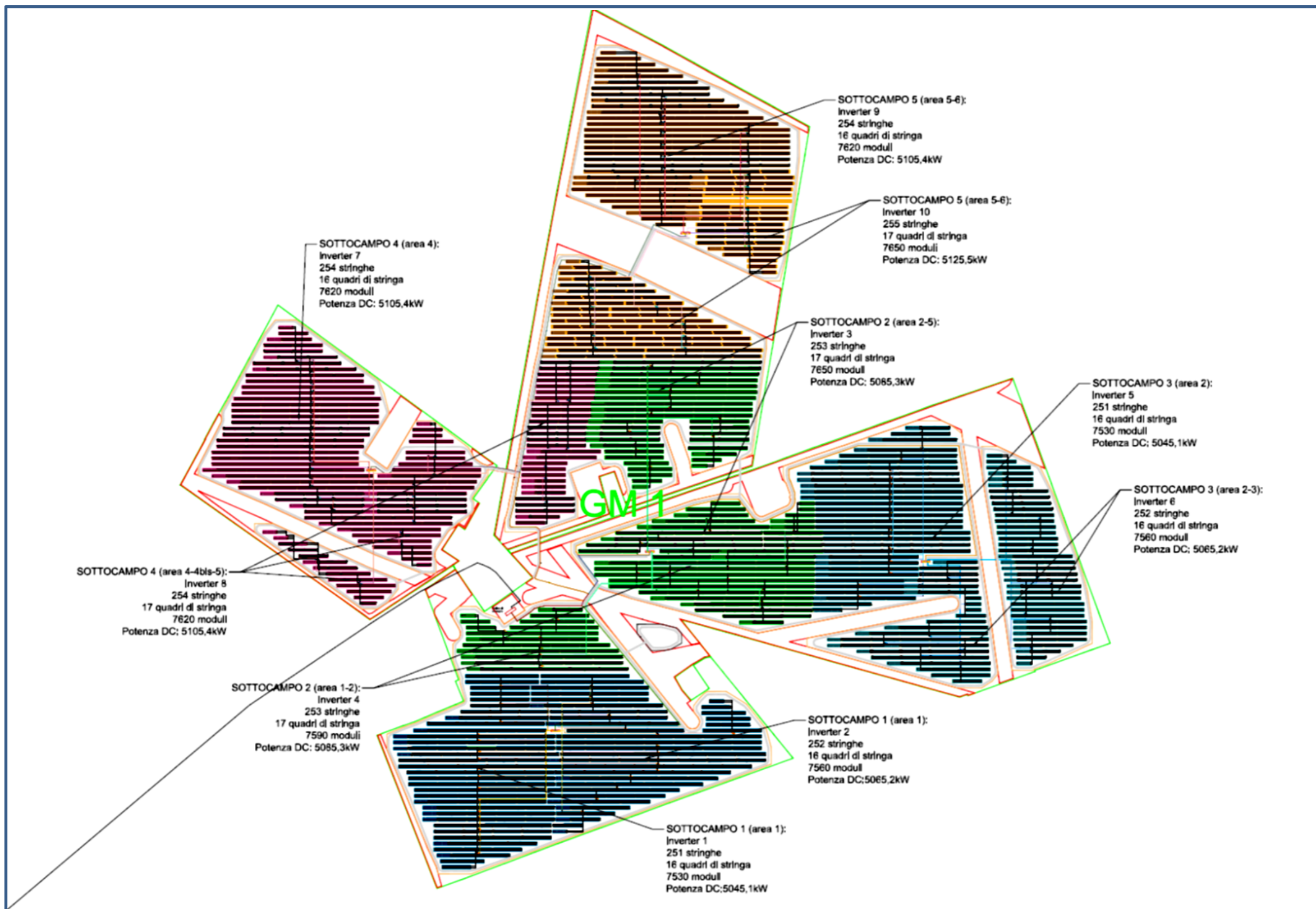
Tav.1.4 Particolare layout di progetto
