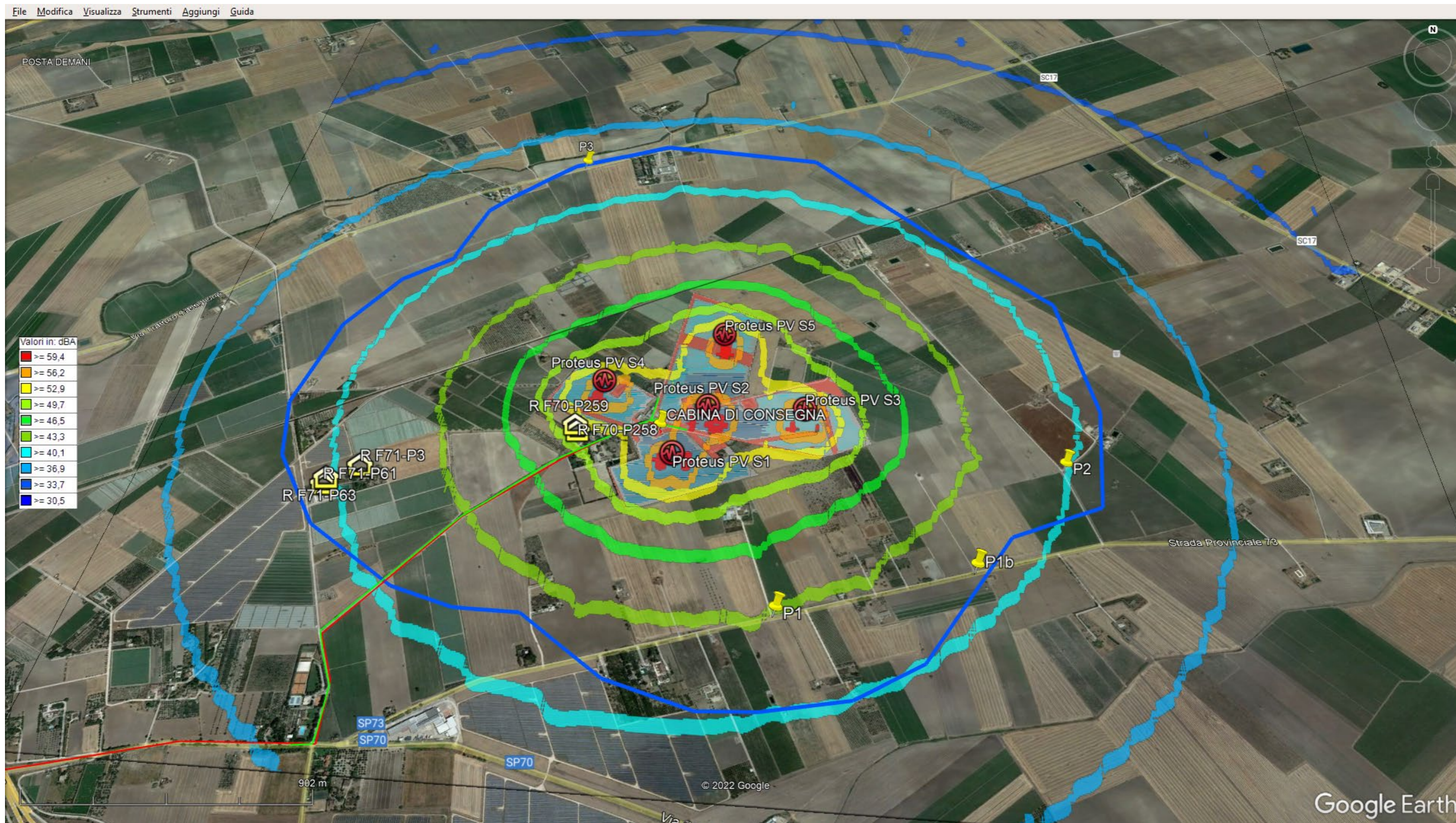
Tavola IS-2 NFTP ISO 9613: sviluppo isofoniche impatto cumulativo su area omogenea senza attenuazioni
