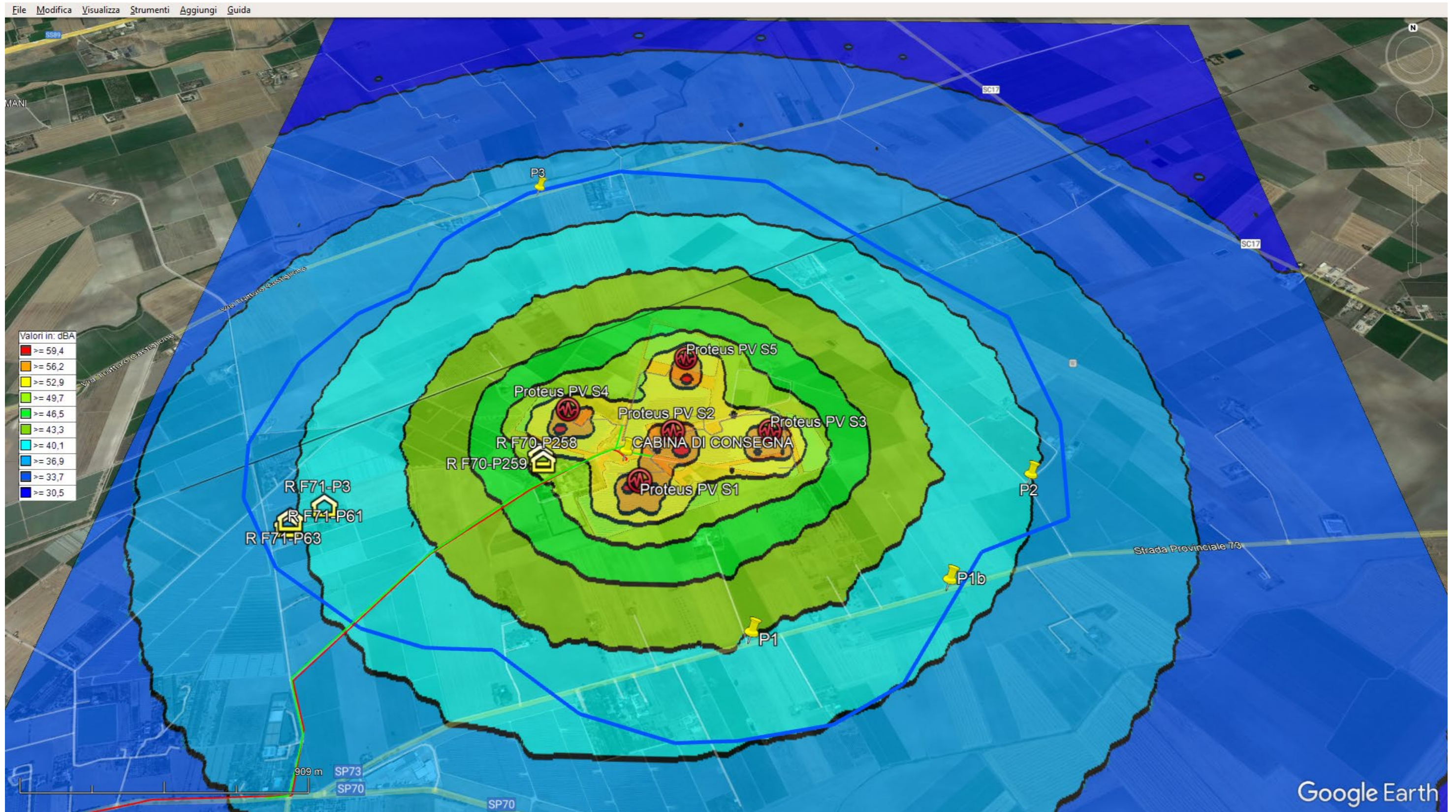
Tavola IS-1 NFTP ISO 9613: sviluppo isofoniche impatto cumulativo su area omogenea senza attenuazioni
