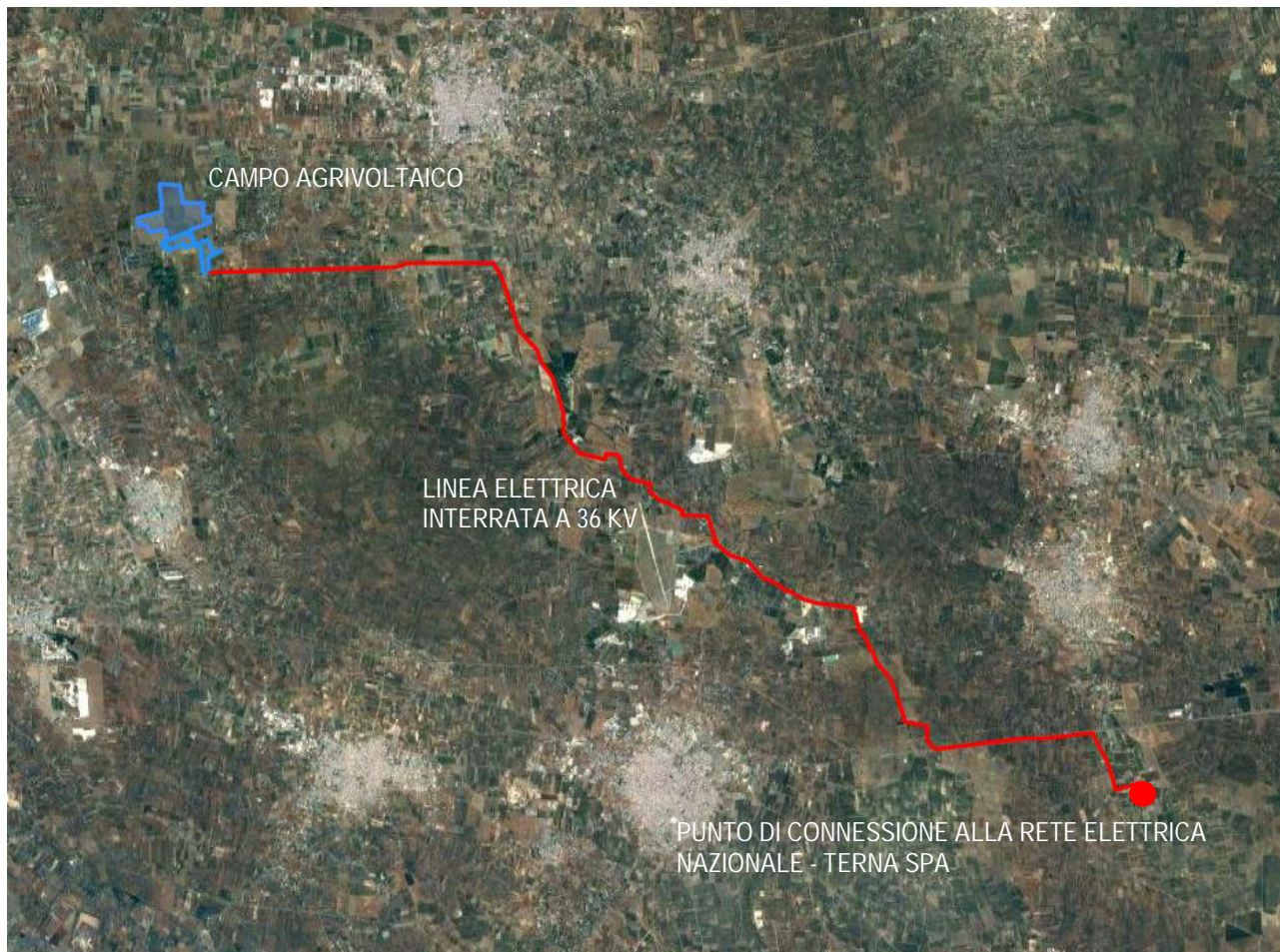
Rappresentazione schematica dell'area d'intervento su base ortofoto
