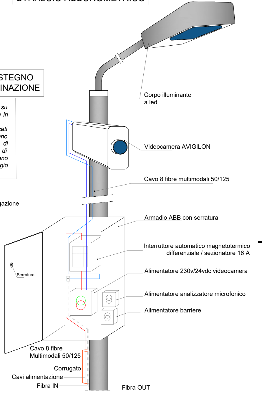
STRALCIO ASSONOMETRICO
